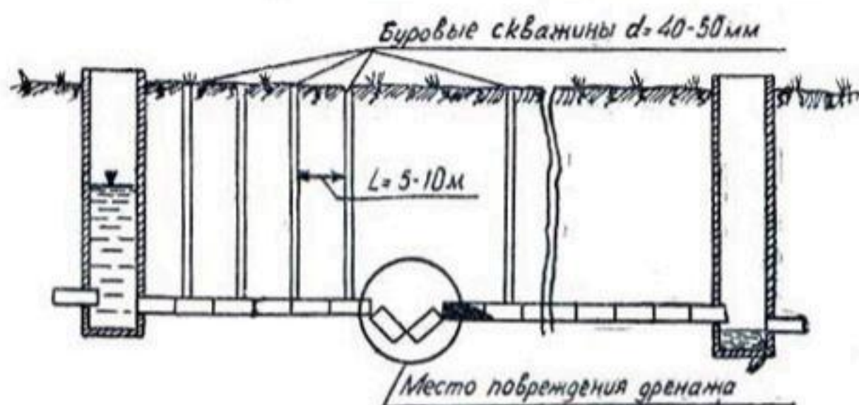
Рис. 8. Определение места повреждения закрытой дренажной трубы с помощью буровых скважин.
