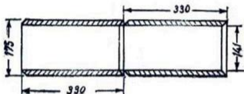
Рис. 3. Фасочное соединение коготких дренажных труб.
