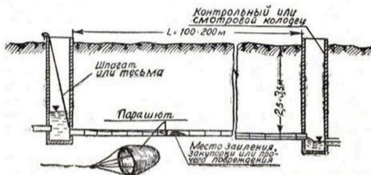
Рис. 7. Определение места повреждения закрытой дренажной системы с помощью «парашюта».
