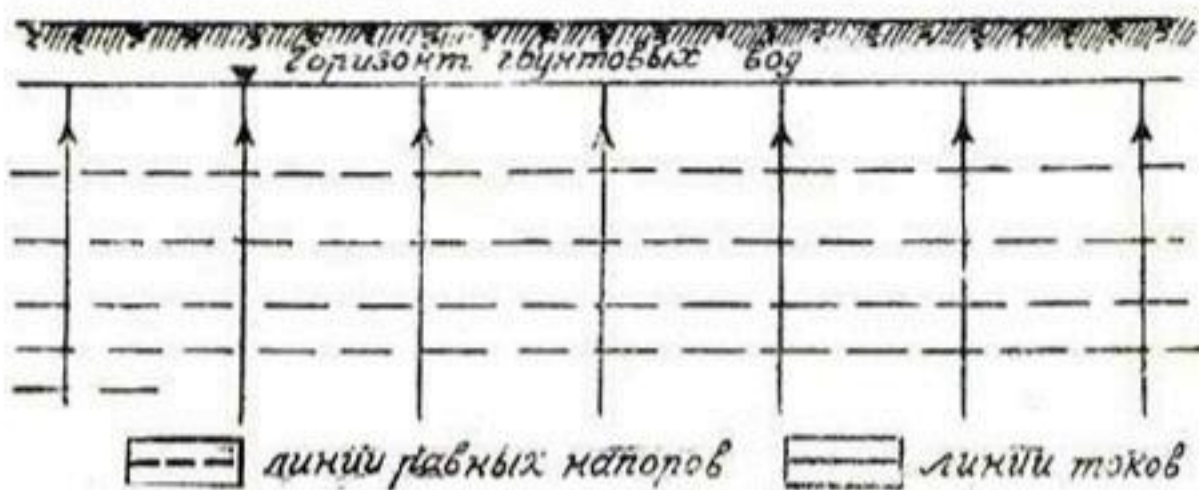
Рис. 12. Схема движения грунтовых вод при напорном питании их в естественных бездренажных условиях.
