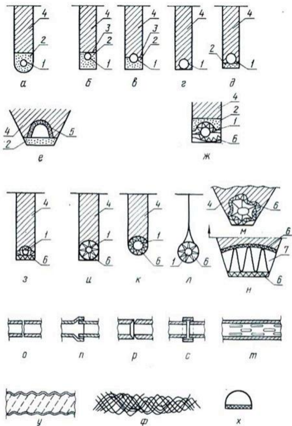
Рис. 24. Конструкция дренажа:
