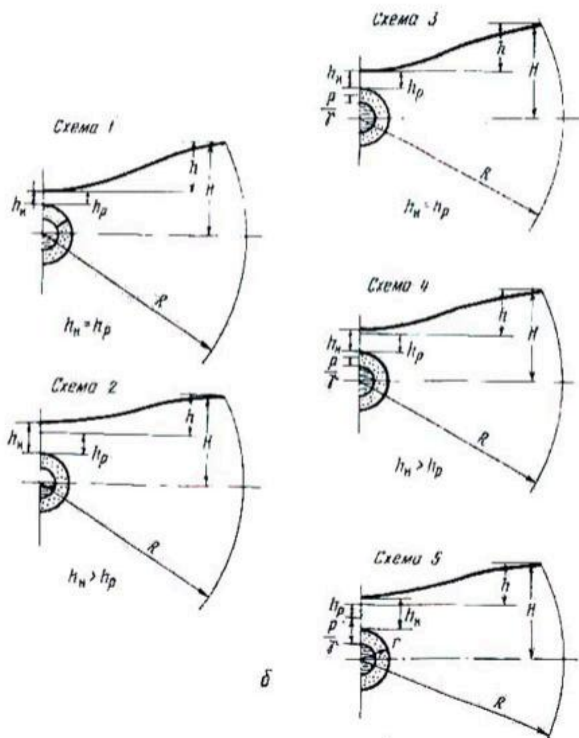
Рис. 29 (продолжение): б — диаметр дрены меньше критического.
