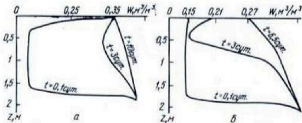
Рис. 7. Эпюра расчета изменения промачивания почвы при постоянной влажности на поверхности и неизменном уровне грунтовых вод: а — коэффициент диффузии на два порядка выше коэффициента водопроницаемости; б — при равных порядках коэффициентов диффузии и водопроницаемости.
