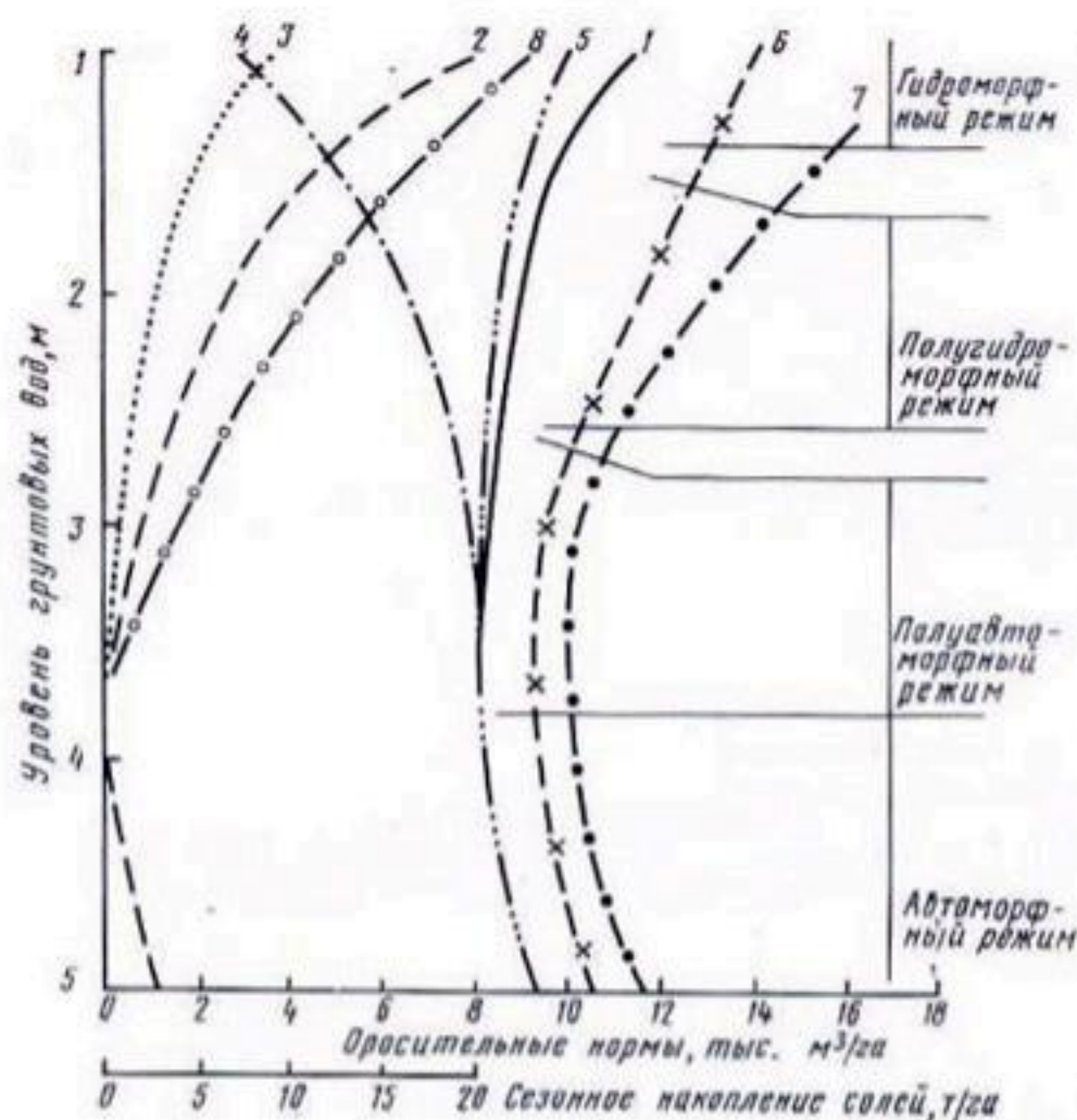
Рис. 17. Сравнительные зависимости оросительных норм, суммарного водопотребления и сезонного соленакопления для различных мелиоративных режимов:
