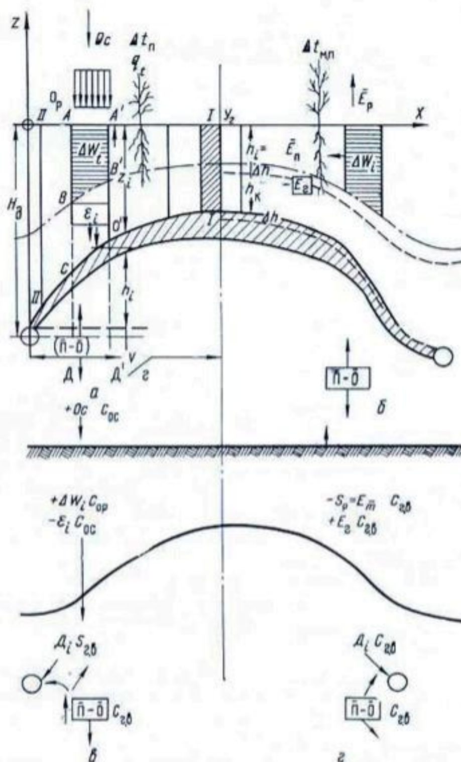
Рис. 6. Формирование положения грунтовых вод на фоне горизонтального дренажа:
