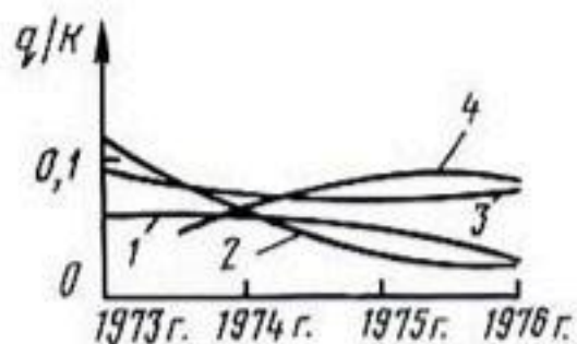
Рис. 40. Изменение дренажного модуля во времени для дрен, уложенных бестраншейным дрепоукладчиком с различными фильтрами:
