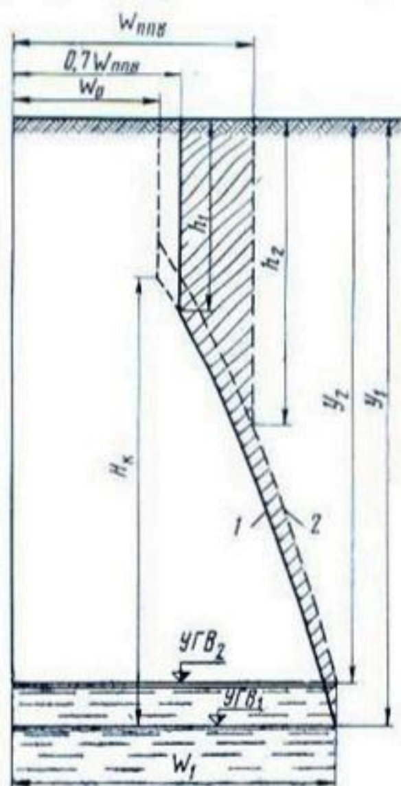
Рис. 19. Расчетные эпюры влажности на начало (1) и конец (2) увлажнения активного слоя почвы при поливе (заштрихована зона изменения влажности).
