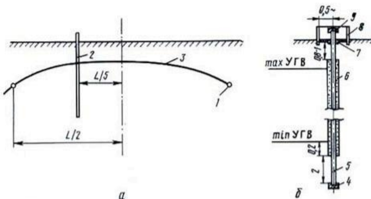
Рис. 43. Наблюдательная скважина горизонтального дренажа: а — схема размещения; б — конструкция скважины; 1 — дрена; 2 — скважина; 3 — депрессионная кривая; 4 — пробка; 5 — отстойник; 6 — фильтр; 7 — глиняный замок; 8 — колодец; 9 — оголовок. (Размеры в м.)
