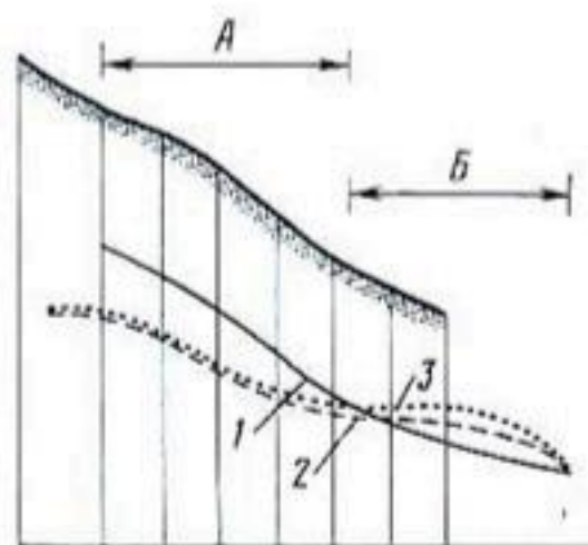
Рис. 23. Схема дрена в совхозе № 14 Каршинской степи:
