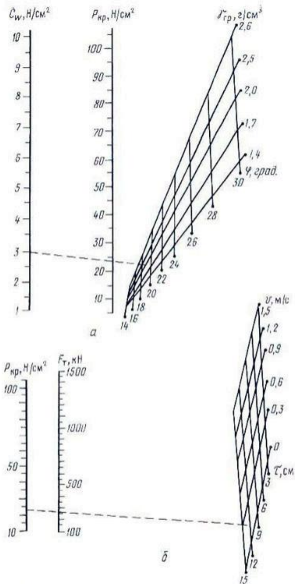
Рис. 38. Номограммы для определения критического напряжения ( a ) и тягового сопротивления ( б ) бестраншейных дренаукладчиков.
