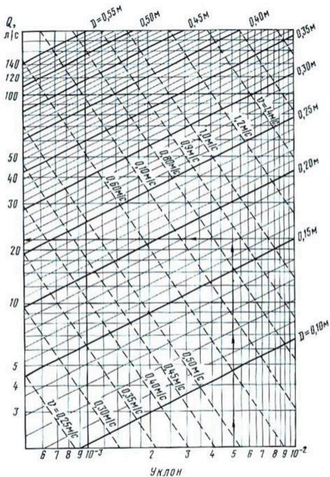
Рис. 31. Помограмма для гидравлического расчета закрытой коллекторно-дренажной сети.
