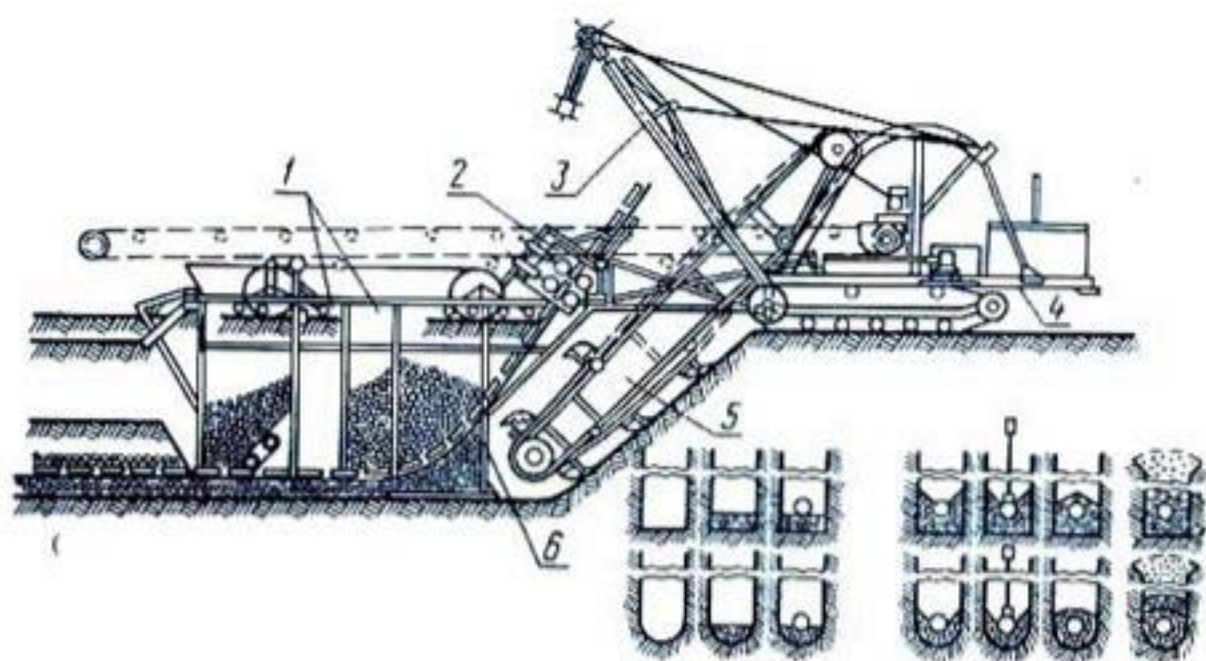
Рис. 32. Последовательность выполнения операций при устройстве закрытого дренажа траншейным дрепоукладчиком в сухих грунтах: 1 — бункер; 2 — подающий механизм; 3 — подъеска бункера; 4 — базовый трактор; 5 — ковшовая рама; 6 — трубоукладчик.
