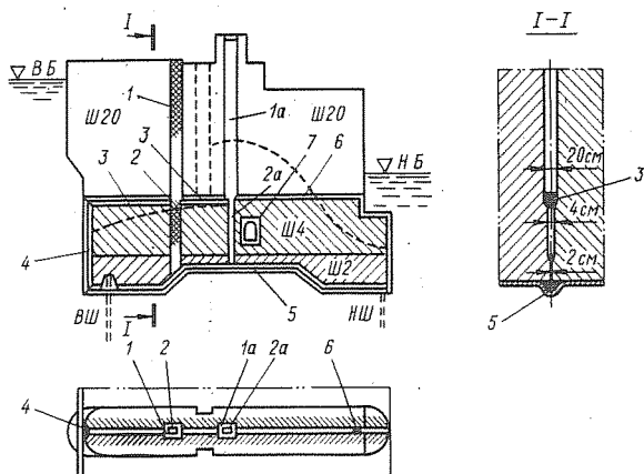
Рис. 2-5. Размещение уплотнений в деформационных швах и швах-надрезах массивного гидросооружения на сжимаемом основании (размеры в см)
