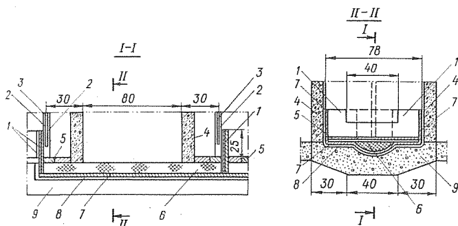
Рис. 6-33. Спряжения горизонтальных (донных) уплотнений с вертикальными асфальтовыми шпонками с вынесенными ограждениями (размеры в см)
