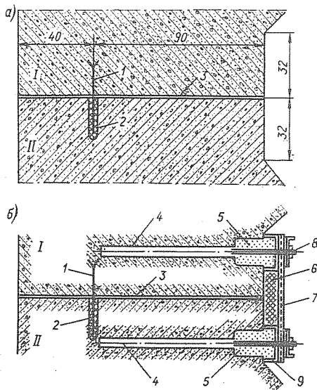
Рис. 6-30. Схема уплотнения осадочного шва в камере шлюза Волжской ГЭС имени ХХП съезда КПСС (размеры в см): а - до ремонта; б - после ремонта
