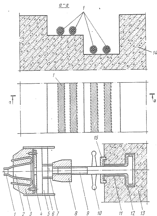
Рис. 1-11. Схема расположения тросов, их натяжения и крепления
