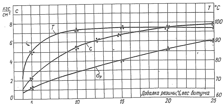
Рис. 3–21. Изменение свойств горячих асфальтовых мастик при введении резины
