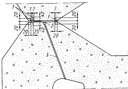
Рис. 6-14. Схема уплотнения температурного шва контрфорсной плотины Миранда (размеры в см)
