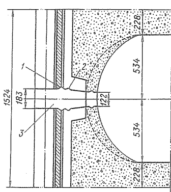
Рис. 6-7. Широкий усадочный шов в контрфорсной плотине Ствян (США) (размеры в см.)
