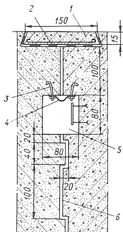
Рис. 6-10. Схема уплотнения температурного шва плотины Чиньяна (размеры в см)
