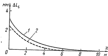
Рис. 1-5. Зависимость величины шва по глубине от наружной грани секции сооружения (при среднегодовой температуре наружного воздуха -0,4^\circ \text{C} )
