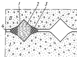
Рис. 3-15. Асфальтовая шпонка с эластичной водонепроницаемой камерой
