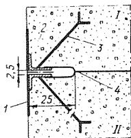
Рис. 6-12. Схема уплотнения температурного шва плотины Альпе Джера (размеры в см)
