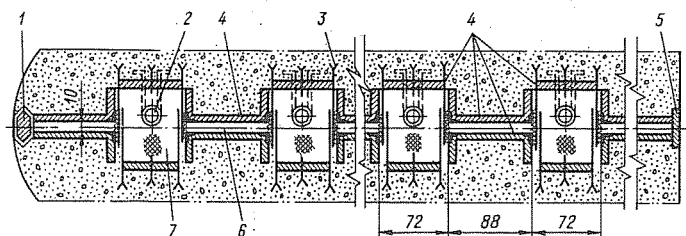
Рис. 6-23. Схемы уплотнения осадочного шва плотины Волжской ГЭС имени В. И. Ленина (размеры в см)
