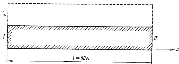
Рис. 1-1. Схема теплового расчета секции плотины Красноярской ГЭС
