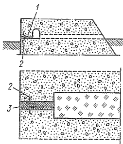
Рис. 2-4. Поперечный разрез плиты горизонтальными швами-надрезами
