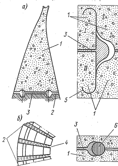
Рис. 2-10. Новые виды конструкции уплотнений горизонтальных (а) и вертикальных (б) температурно-усадочных швов в арочной плотине
