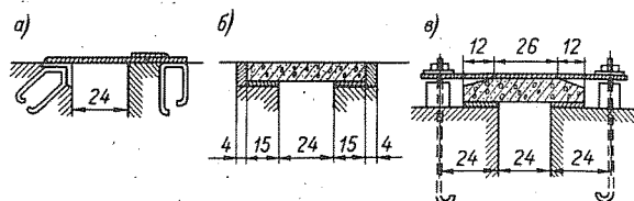
Рис. 3-17. Схемы защитных наружных контурных уплотнений осадочных швов (размеры в см): а - от мусора; б - в горизонтальных перекрытиях; в - на вертикальных стенах
