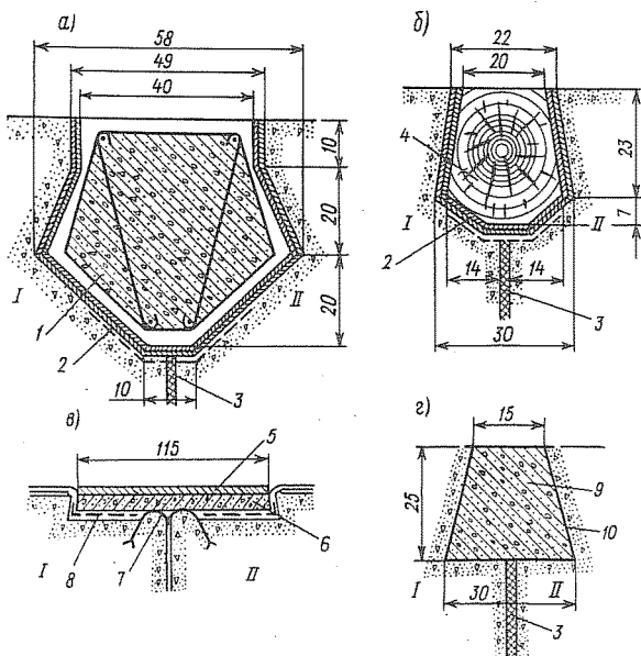
Рис. 3-16. Схемы наружных контурных уплотнений температурных швов на напорных гранях плотины (размеры в см): а - выше уровня минимальной сработки водохранилища; б - ниже уровня минимальной сработки водохранилища; в - плотина Карсер (Италия); г - на тыловой грани сооружения.
