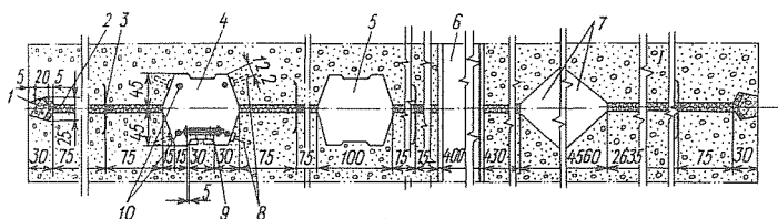
Рис. 3-10. Схема асфальтовой шпонки в температурном шве плотины Братской ГЭС (размеры в см)
