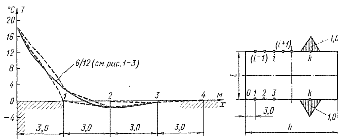
Рис. 1-4. Схема приложения треугольной температурной нагрузки единичной интенсивности
