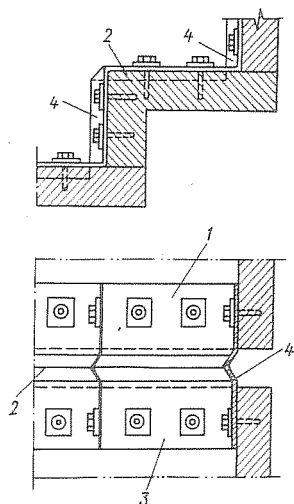
Рис. 5-15. Приспособление V-образного профиля для соединения сборной конструкции уплотнения по рис. 5-14
