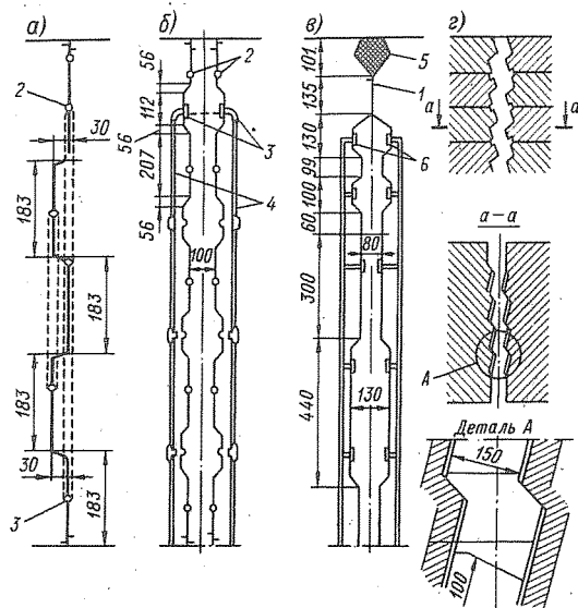
Рис. 2–7. Схема конструкции температурно-усадочных швов (размеры в см): а – нормальный (узкий) шов; б – расширенный шов; в – смешанный шов; г – расширенный шов смешанного типа
