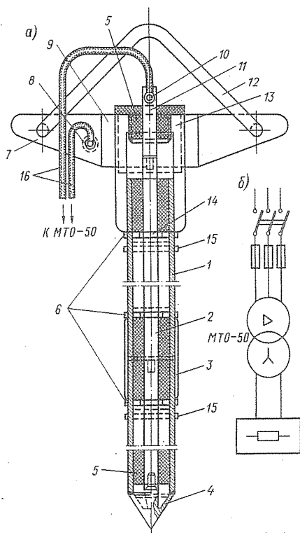
Рис. 3-23. Переносный сборно-разборный электронагреватель: а - общий вид; б - схема электрического соединения (размеры в см)
