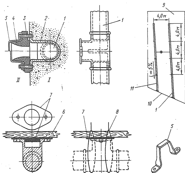
Рис. 2-12. Схема выпуска "капитан" для многократной цементации шва
