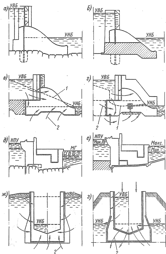
Рис. 1-9. Принципиальные схемы расположения контура уплотнений в деформационных швах гидротехнических сооружений
