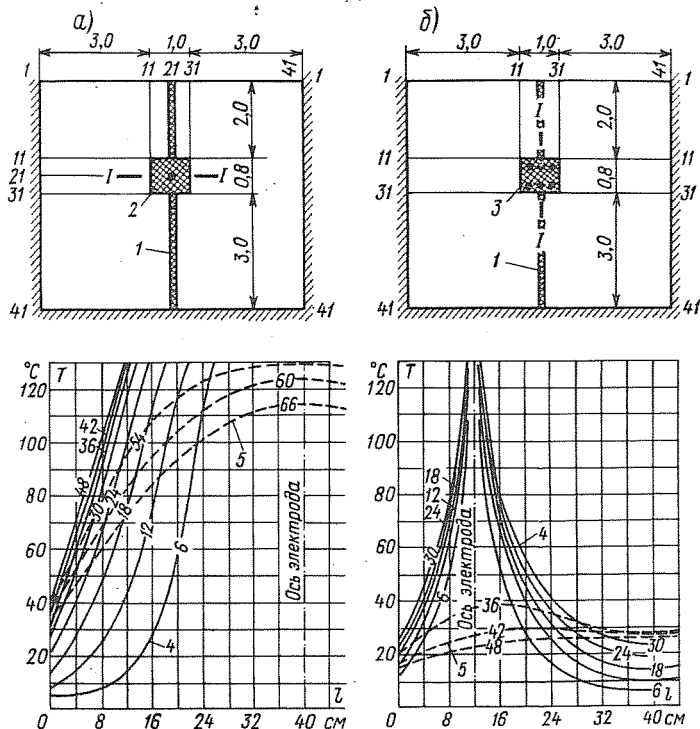
Рис. 3-25. Расчетные схемы и кривые распределения температуры в асфальтовой мастике: а - при Э-электронагревателе ( q_3^0 = 3600 \text{ ккал}/(\text{м}^2 \cdot \text{ч}) ); б - при U-электронагревателе ( q_4^0 = 600 \text{ ккал}/(\text{м}^2 \cdot \text{ч}) ). Обозначения те же, что и на рис. 3-24
