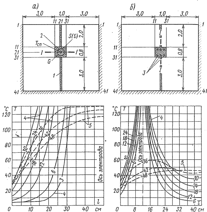
Рис. 3-24. Расчетные схемы и кривые распределения температуры в асфальтовой мастике: а - при Э-электронагревателе ( q_{\text{Э}}^0 = 4800 \text{ ккал}/(\text{м}^2 \cdot \text{ч}) ); б - при U-электронагревателе ( q_{\text{U}}^0 = 800 \text{ ккал}/(\text{м}^2 \cdot \text{ч}) )
