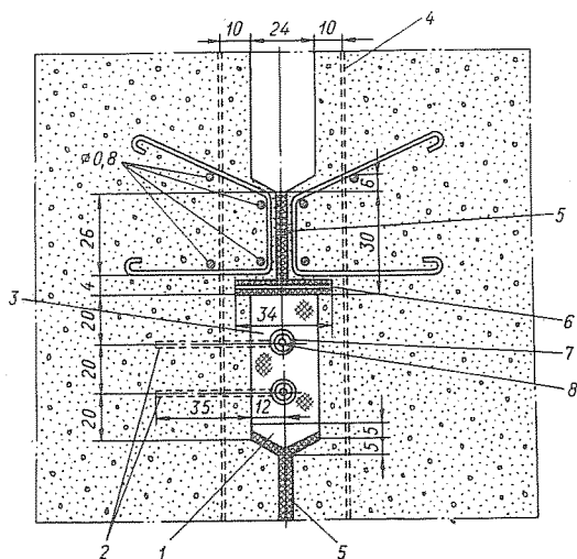
Рис. 3-12. Схема горизонтальной асфальтовой шпонки (размеры в см)
