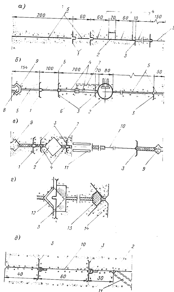
Рис. 6-8. Уплотнения температурных швов плотин металлическими диафрагмами (размеры в см): а - Саньмынься; б - Красноярская ГЭС; в - Усть-Илимская ГЭС; г - Кременчугская ГЭС (шлюз); д - Кайтакоски
