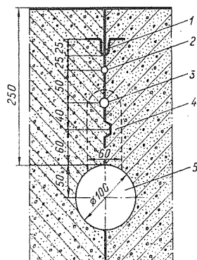
Рис. 6-17. Схема уплотнения температурного шва плотин Саланфе, Талепперо и Клэзон (размеры в см)
