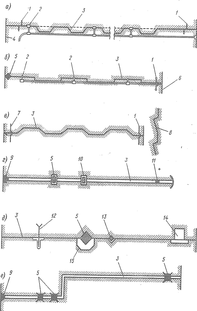
Рис. 1-8. Схема компоновки уплотнений в деформационных швах гидросооружений (горизонтальные разрезы): а - плотина Дакан (Ирак); б - плотина Кушман (США); в - плотина Чиркейской ГЭС; г - плотина Каховской ГЭС; д - Усть-Каменогорская плотина; е - Рыбинская ГЭС
