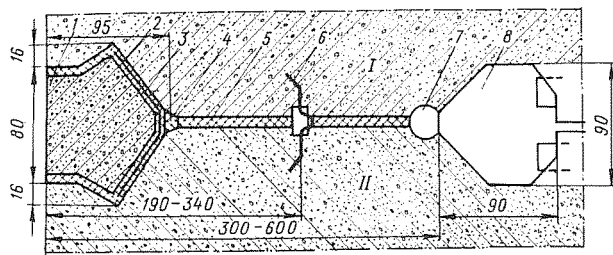
Рис. 6-13. Схема уплотнения температурного шва плотины Биказ имени В. И. Ленина (размеры в см)
