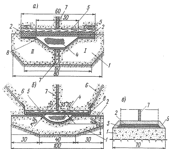
Рис. 3-11. Схемы горизонтальных уплотнений деформационных швов по подшове сооружения (размеры в см) на сжимаемых (а, б) и на скальных (в) основаниях: а - на плотине и здании Каховской ГЭС; б - на плотине Воткинской ГЭС; в - на плотине Братской ГЭС
