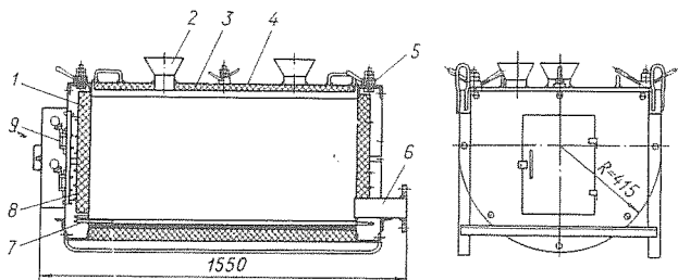
Рис. 5-7. Раздаточный котел емкостью 300 л (размеры в см)
