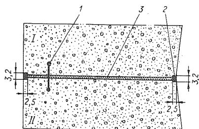
Рис. 6-3. Схема уплотнения температурного шва плотины Борисоглебской ГЭС (размеры в см)
