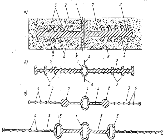
Рис. 3-2. Конструкции уплотнений из эластичного синтетического материала (Швеция)
