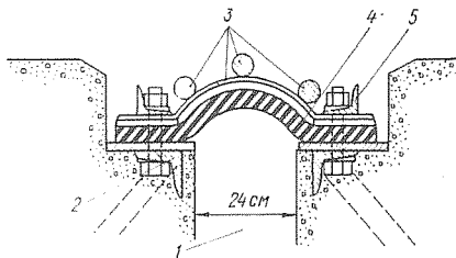
Рис. 6-20. Схема резинового контурного уплотнения машинного зала здания Воткинской ГЭС
