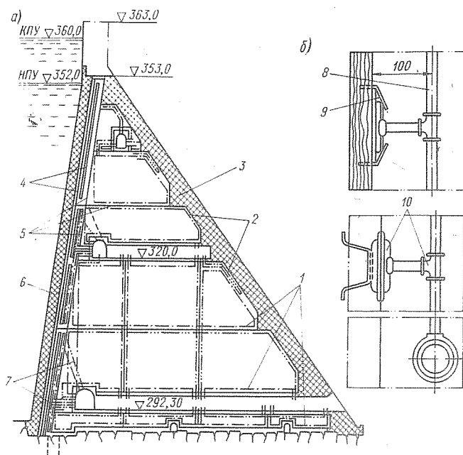
Рис. 2-11. Схема поперечного разреза плотины Саньмынься (а) и тарельчатого выпуска (б) для одноразовой цементации шва (размеры в мм)
