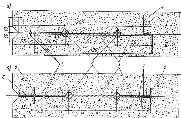
Рис. 6-4. Уплотнение температурного шва частей плотины План д'Амон (Франция), расположенных на кристаллических (а) и зеленых (б) сланцах (размеры в см)
