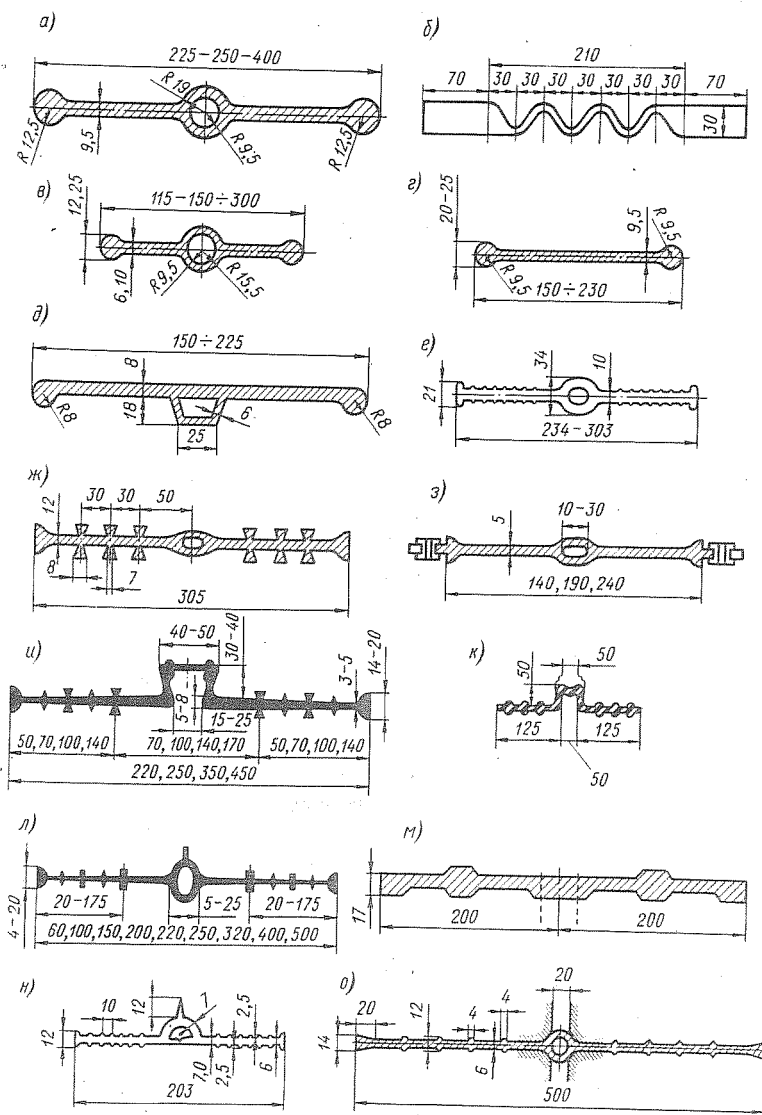
Рис. 3-1. Схемы некоторых профилей резиновых (а-д) и полимерных (е-о) лент (размеры в мм)
