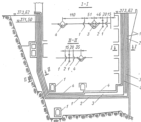
Рис. 6-2. Схема уплотнения температурного шва здания ГЭС Бхакра (Индия) (размеры в см)
