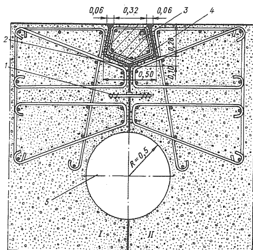
Рис. 6-6. Схема уплотнения температурного шва итальянской плотины Кварра Делла Миньера (размеры в м)
