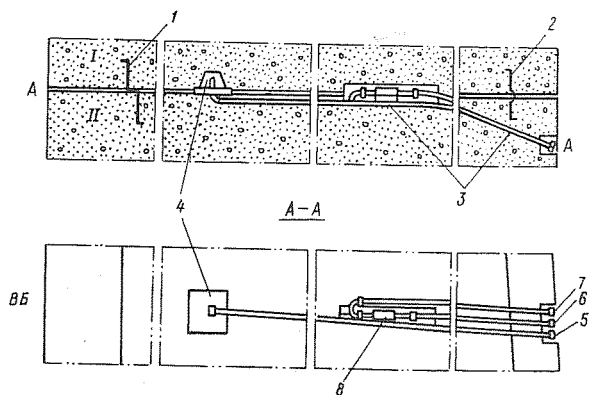
Рис. 6-26. Уплотнение температурно-усадочных швов арочно-гравитационных плотин Спеккери (Италия)
