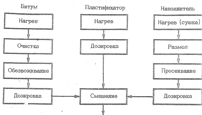
Рис. 5-5. Технологическая схема приготовления битумно-полимерного герметика
