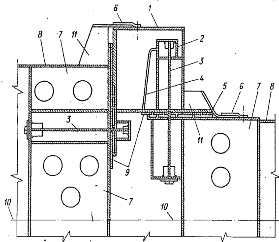
Рис. 1-12. Схема скользящего соединения трубопровода (по дну залива Сан-Франциско)
