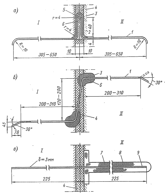
Рис. 3-3. Схемы металлических диафрагм (размеры в мм): а, б - с компенсаторами; в - без компенсатора; I - первая очередь бетонирования; II - вторая очередь (в дальнейшем для очередности бетонирования сохранены те же обозначения)
