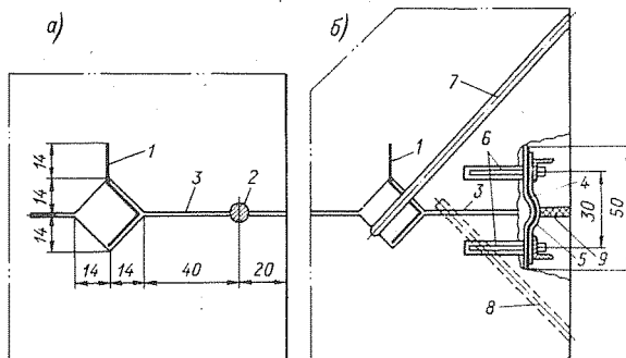
Рис. 6-31. Схема уплотнения осадочного шва в камере шлюза Верхне-Свирской ГЭС (размеры в см): а - до ремонта; б - после ремонта
