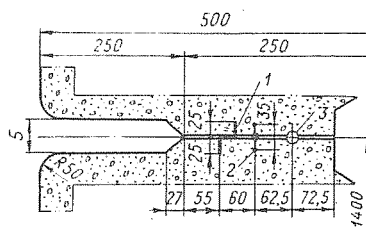
Рис. 6-25. Уплотнение температурного шва контрфорсной плотины Менжил (размеры в см)
