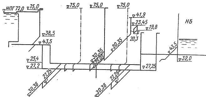
Рис. 6-29. Схема электронагрева асфальтовых шпонок здания Плявиньской ГЭС
