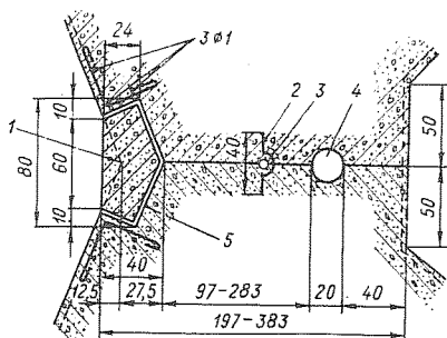
Рис. 6-5. Схема уплотнения температурного шва контрфорсной плотины Дживаретто (размеры в см)
