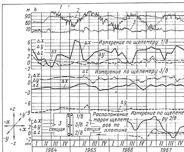
Рис. 1-7. График измерения раскрытия швов по щелемерам
