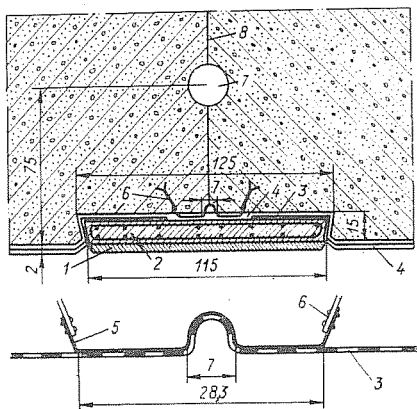
Рис. 6-9. Схема уплотнения температурного шва плотины Карсер (размеры в см)
