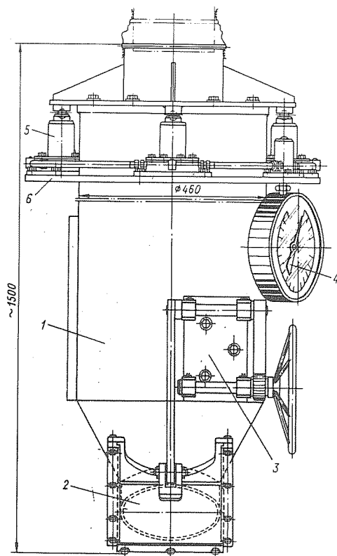
Рис. 5-2. Дозатор минеральных наполнителей ДМ-200 (размеры в мм)
