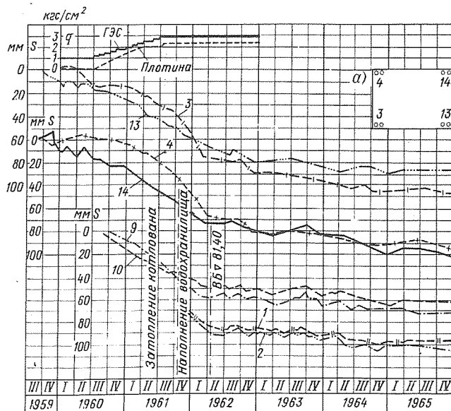
Рис. 1-6. Графики нагрузки q и осадки S секции №3 Ватkinsкой сливной плотины. Цифрами у кривых обозначены соответствующие
