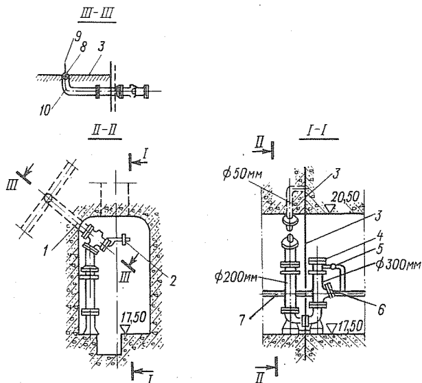
Рис. 3-22. Питательные колонки в инспекционной галерее Кегумской ГЭС
