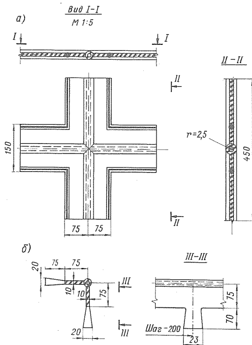
Рис. 6-35. Новая конструкция уплотнения из резины и полимерных диафрагм на пересечениях деформационных швов (размеры в мм): а - при пересечениях горизонтальной и вертикальной диафрагм; б - при оконтуривании вертикальной полости с горизонтальной
