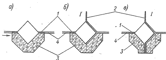
Рис. 3-13. Нерекомендуемые схемы ограждений асфальтовых шпонок в температурных швах: а - ограждение шпонок конопаткой, просмоленной паклей; б - ограждение шпонок, установленной внутри металлической диафрагмы, и одним концом заделанной в бетон I; в - ограждение шпонок металлической диафрагмой, одним концом заделанной в бетон I, вторым концом выпущенной между корытами
