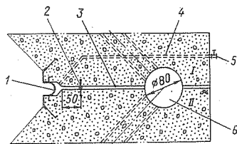
Рис. 6-1. Схема уплотнения температурного шва плотины Мерайе (Франция) (размеры в см)
