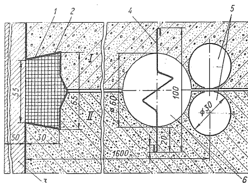
Рис. 6-18. Схема уплотнения температурного шва плотины Бела Искер (Болгария) (размеры в см.) 1 - медный лист; 2 - асфальтовая шпонка; 3 - облицовка напорной грани бутовой кладкой; 4 - медная диафрагма; 5 - дрена; 6 - смотровая шахта
