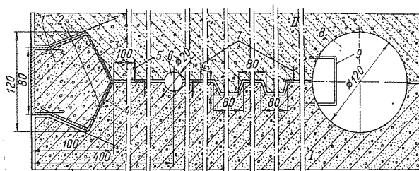
Рис. 6-11. Схема уплотнения температурного шва плотины Гранд-Диксанс (размеры в см)
