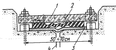
Рис. 3-20. Новый тип прижима резиновых уплотнений
