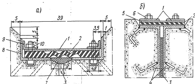
Рис. 3-18. Схемы наружных контурных уплотнений узких осадочных швов (размеры в см) с резиновой профилированной лентой: а - на камерах шлюзов Воткинской ГЭС, Волжской ГЭС имени XXII съезда КПСС; б - на плотине Империзэл (США)
