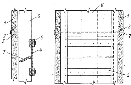
Рис. 5-12. Схема монтажа железобетонных коробов и шандоров
