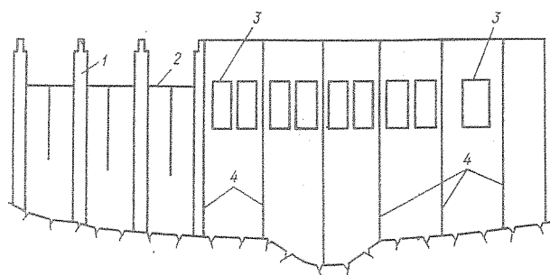
Рис. 2-2. Температурные швы плотины с водопропускными отверстиями на однородном скальном основании
