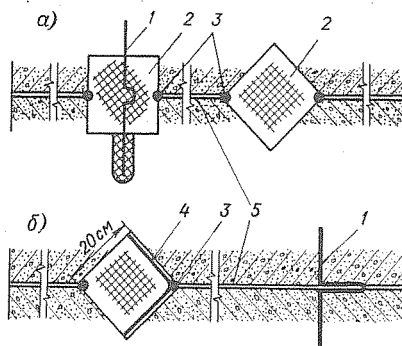
Рис. 6-21. Схемы уплотнений осадочного шва Нижне-Свирской ГЭС: а - на водосливной плотине; б - на здании ГЭС
