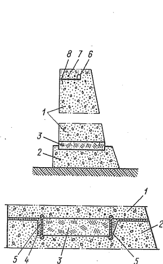
Рис. 2-9. Новые конструктивные швы-надрезы в арочной плотине
