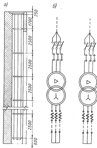
Рис. 6-28. Схема электронагрева асфальтовых шпонок в сооружениях Кременчугской ГЭС: а – общий вид; б – схема электрических соединений электронагрева (размеры в мм)
