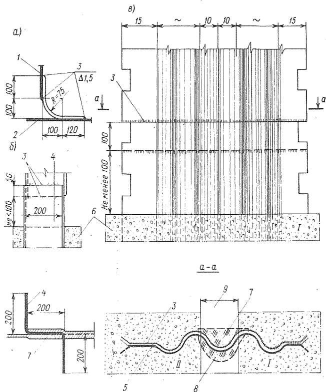
Рис. 5-11. Сопряжения металлических диафрагм (размеры в мм): а – плоских вертикальных и горизонтальных; б – Z-образных; в – вертикальных гофрированных
