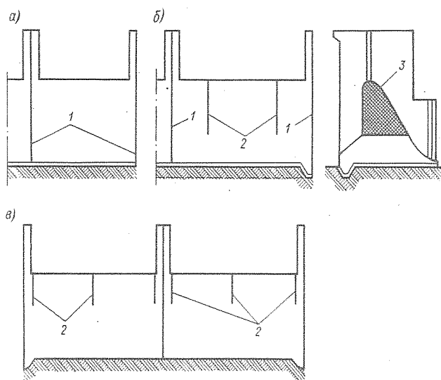
Рис. 2-1. Схема разрезки сооружения на сжимаемом основании деформационными швами: а – только сквозными швами; б – смешанной системой сквозных и несквозных швов; в – только одними несквозными швами
