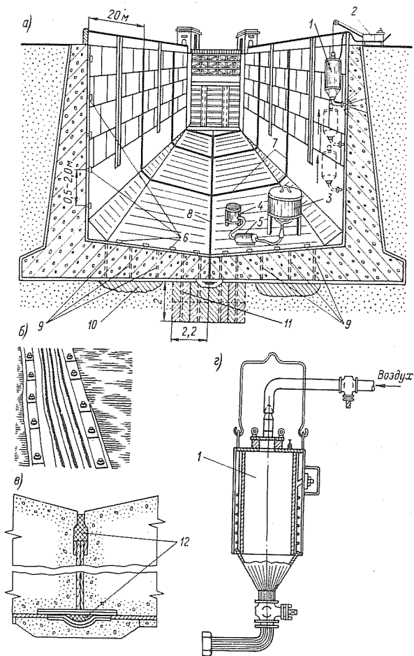
Рис. 6-32. Схема ремонта уплотнений осадочных швов камер шлюзов № 7 и 13 Волго-Донского канала имени В. И. Ленина: а - общая схема камеры шлюза; б - уплотнение продольного шва; в - шпонка продольного шва днища; г - битумный инъе́ктор
