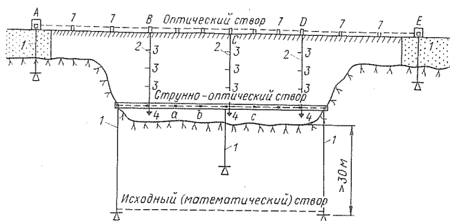
Рис. 6-30. Схема измерения плановых перемещений высокой бетонной гравитационной плотины на скальном основании
