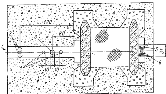
Рис. 6-34. Схема ремонта уплотнений осадочных швов здания Волжской ГЭС имени В. И. Ленина (размеры в см)
