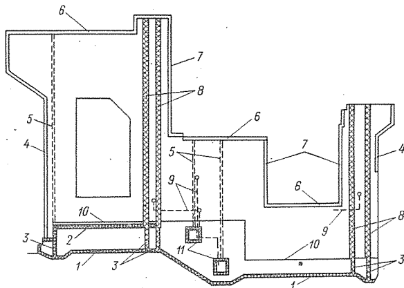
Рис. 1-10. Схема расположения уплотнений в широком деформационно-осадочном шве здания ГЭС с замкнутым контуром с верхней и нижней сторон, при частичном или полном осушении полости шва и при наличии неоднородного сжимаемого основания
