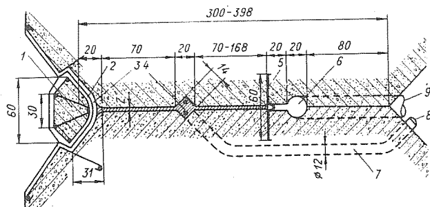
Рис. 6-15. Уплотнение температурного шва контрфорсной плотины Бай Муджерис и Саббиона (размеры в см)
