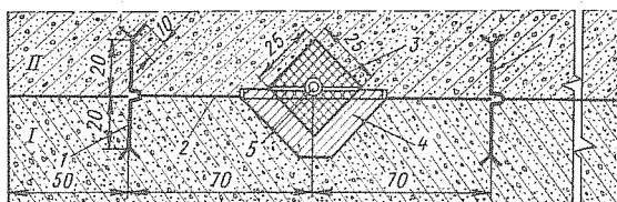
Рис. 6-16. Уплотнение температурного шва плотины Маманской ГЭС (размеры в см)
