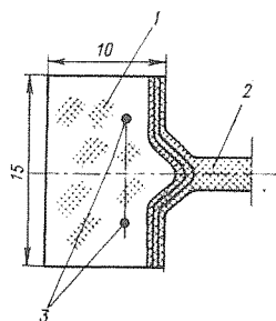
Рис. 6-22. Схема уплотнения осадочного шва Фархадской ГЭС (размеры в см)
