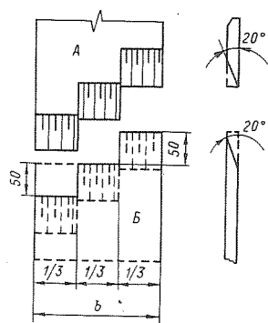
Рис. 5-10. Схема сращивания резиновых лент
