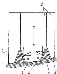
Рис. 2-3. Секция плиты с разрезкой температурного шва в основании наклонными или клиновидными швами
