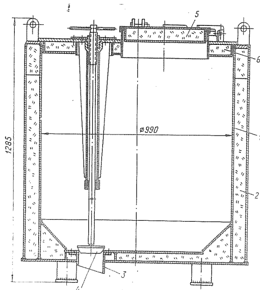
Рис. 5-4. Бадья-термос емкостью 600 л (размеры в мм)
