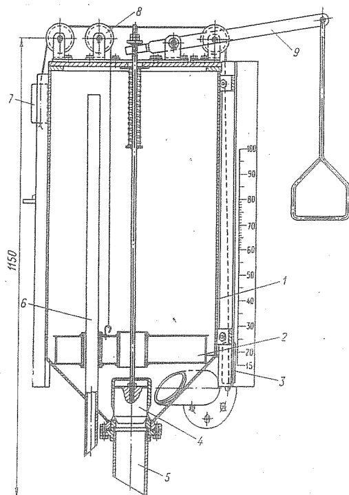
Рис. 5-1. Дозатор битума ДБ-100 (размеры в мм)
