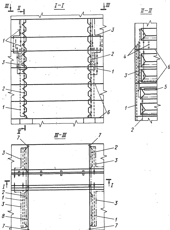
Рис. 2-6. Столбчатая разрезка плотины и схема цементации температурных швов
