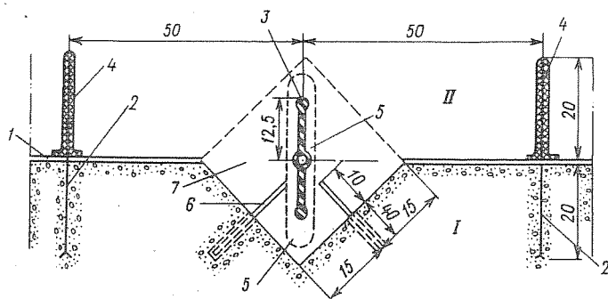
Рис. 3-14. Комбинированная вертикальная асфальтовая шпонка с профилированной резиновой лентой
