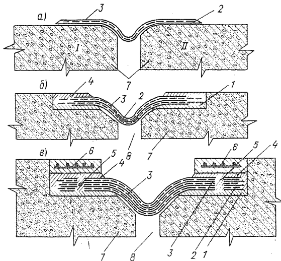
Рис. 5-16. Безанкерные поверхностные уплотнения клеечного типа: а — однослойное; б — двухслойное с пластрастворной подготовкой площадок сцепления; в — трехслойное усиленное с перфорацией
