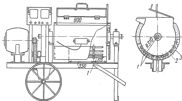
Рис. 5-6. Асфальтосмесительная установка ВНИИГ
