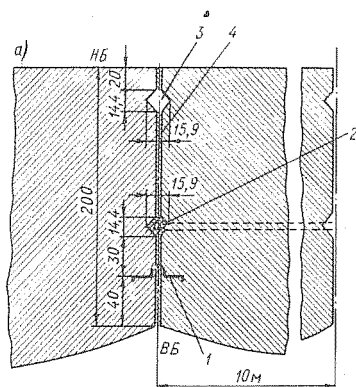
Рис. 6-18. Схема уплотнения температурного шва плотины Бела Искер (Болгария) (размеры в см.) 1 - медный лист; 2 - асфальтовая шпонка; 3 - облицовка напорной грани бутовой кладкой; 4 - медная диафрагма; 5 - дрена; 6 - смотровая шахта
