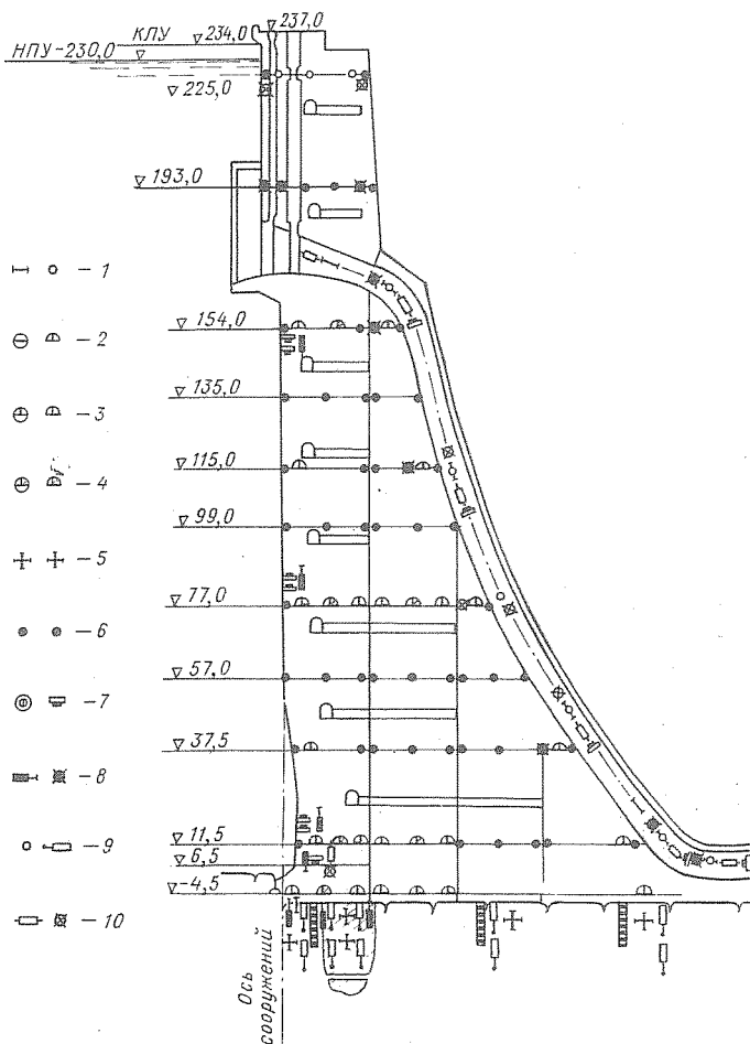
Рис. 6-38. Схема размещения КИА в арочно-гравитационной плотине
