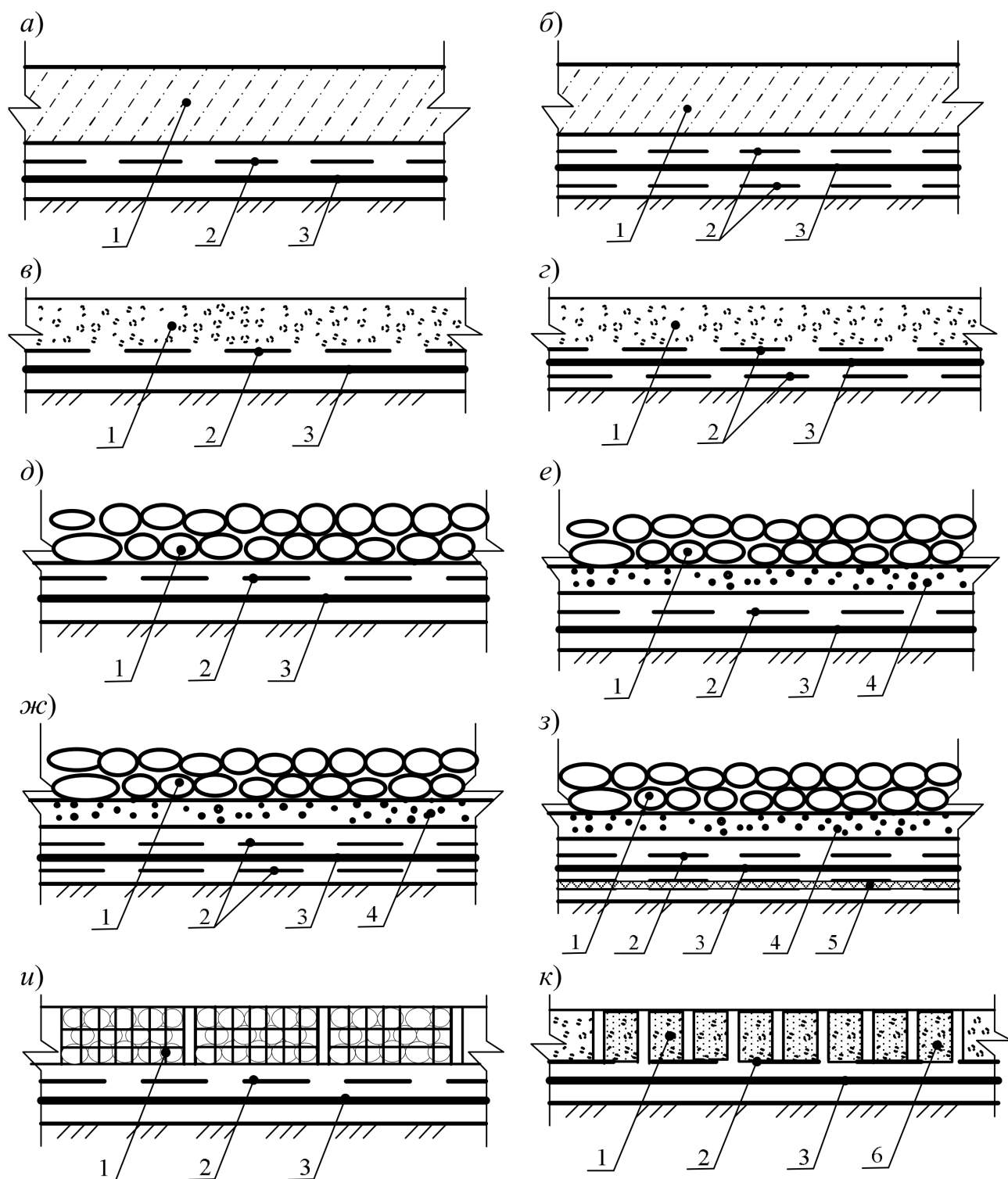
а, б – с геомембраной и защитным покрытием из бетона; в, г – с геомембраной и защитным покрытием из грунта; д, з – с геомембраной и защитным покрытием из каменной наброски; и, к – с геомембраной и защитным покрытием из габионов и георешетки; 1 – защитное покрытие; 2 – защитная прокладка из геотекстиля; 3 – противофильтрационный элемент из геомембраны; 4 – защитный слой из песка; 5 – дренажный элемент из геокомпозита; 6 – георешетка; 7 – габионы
