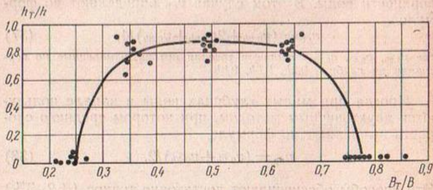
Рис. 11. График зависимости B_T/B = f(h_T/h) .
