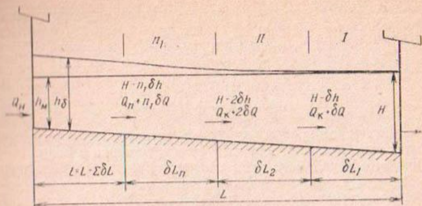
Рис. 45. Расчетная схема:
