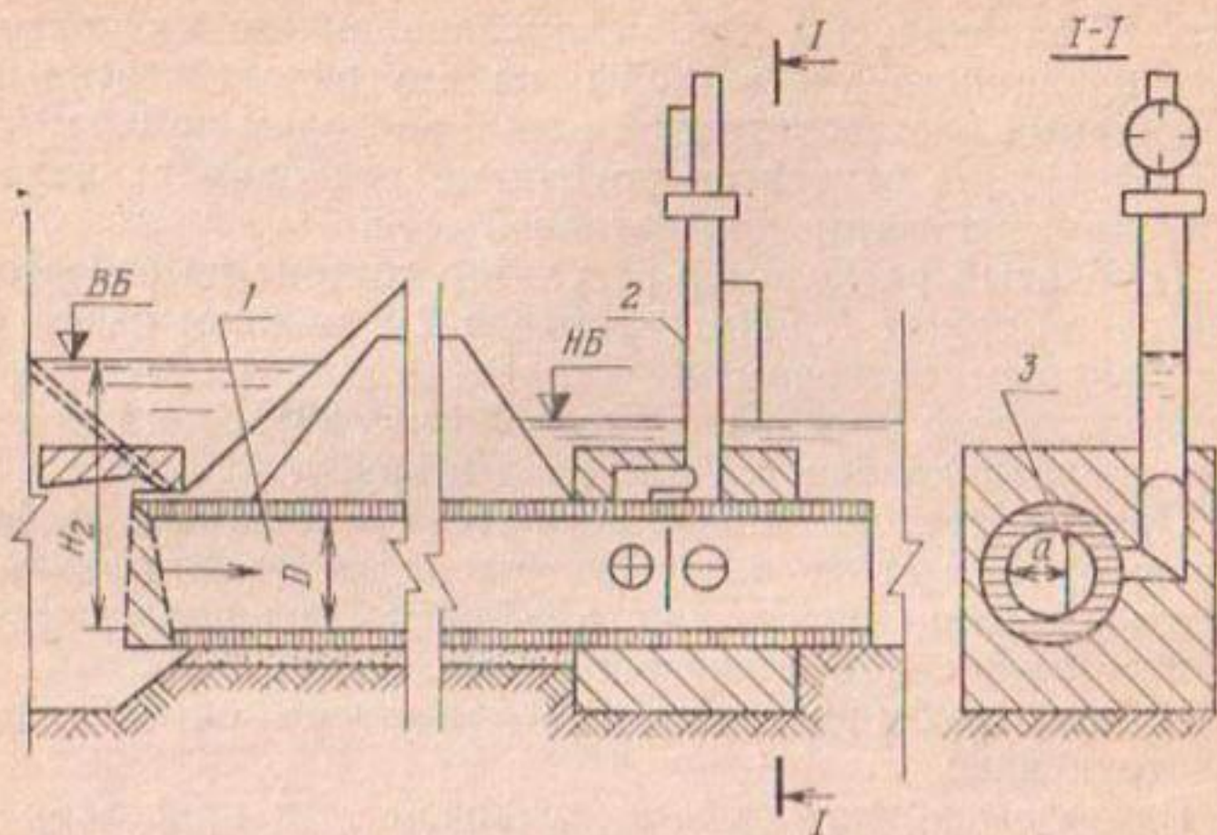
Рис. 24. Схема расходомера-водовыпуска с сегментной диафрагмой:
