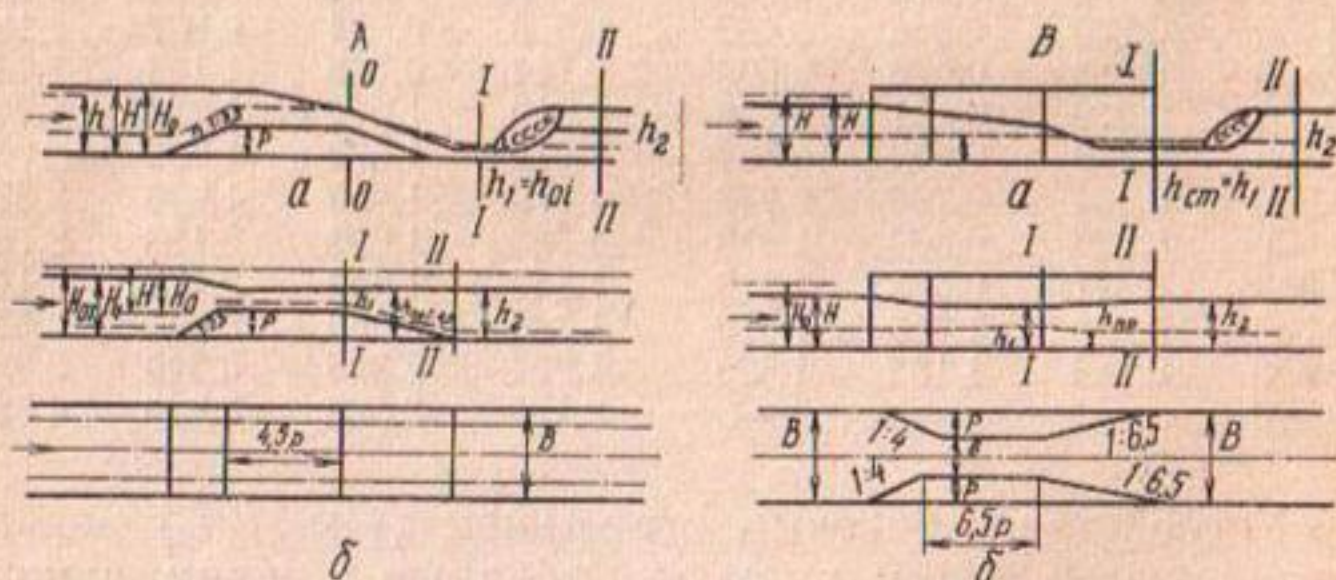
Рис. 7. Схема устройства с донным стеснением (А) и с плавным боковым (В): а — свободное истечение; б — затопленное.
