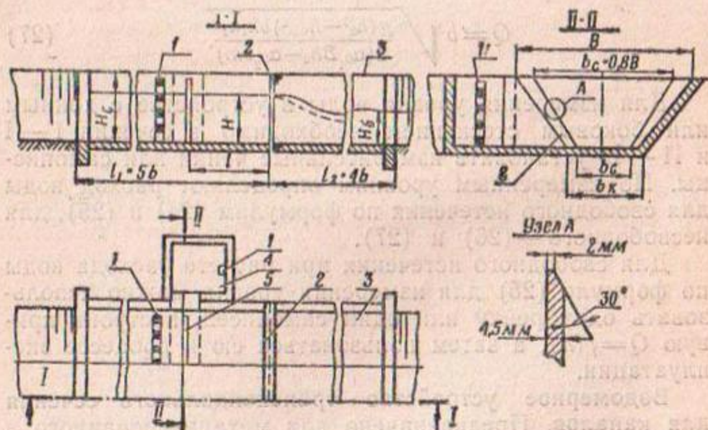
Рис. 8. Схема водомерного устройства для каналов трапецеидального сечения:
