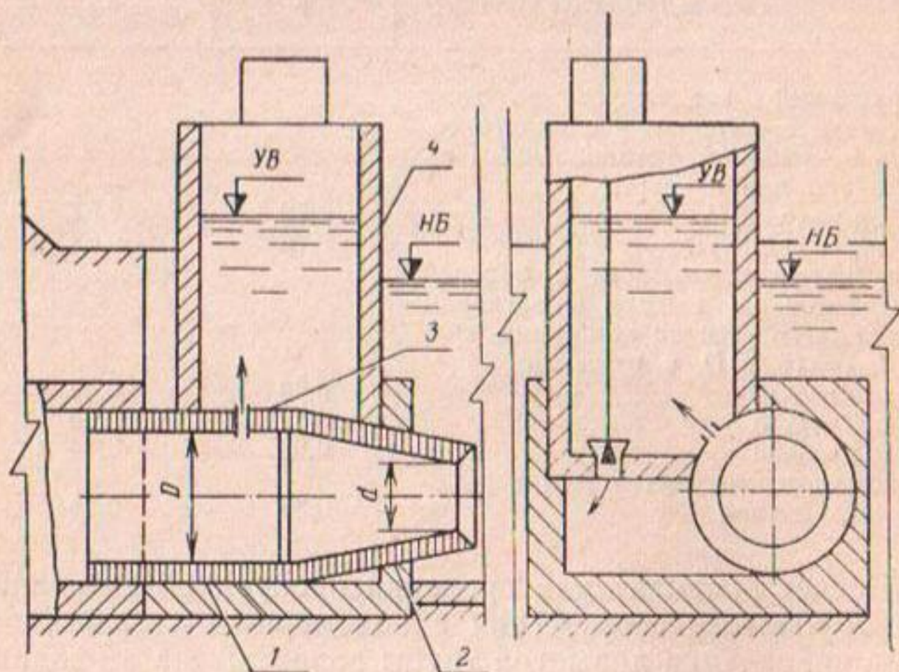
Рис. 26. Схема трубчатого расходомера-регулятора с насадком на входе:
