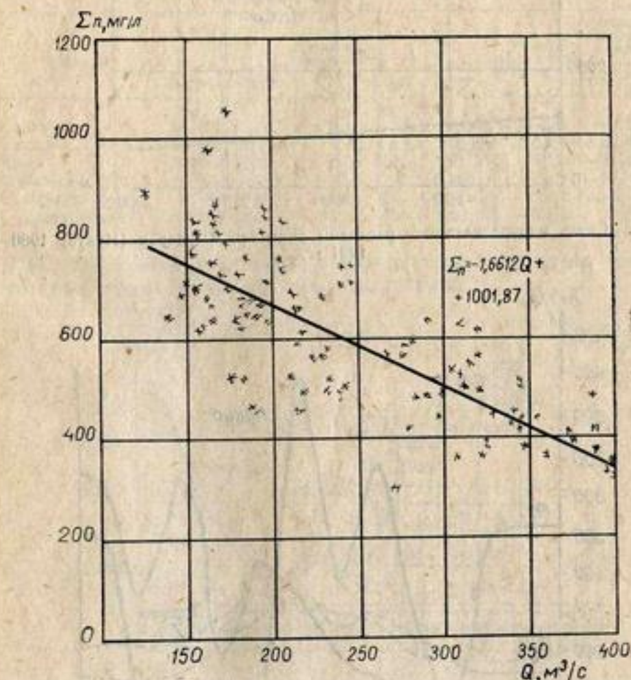
Рис. 3. Связь минерализации с расходом воды р. Амударьи (Термез, протока) 1980—1991 гг.
