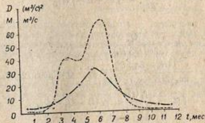
Рис. 1. Математическое ожидание (М) и спектр дисперсий (Д) средних месячных расходов воды р. Акдарья за 1927—1989 гг.
