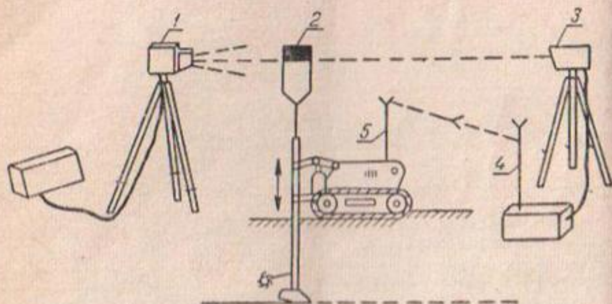
Рис. 39. Поддержание глубины копания автоматизированным визированием:
