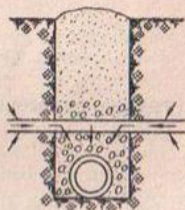
Рис. 5. Комбинированный дренаж.
