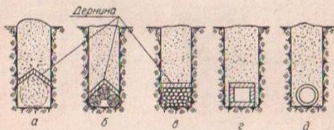
Рис. 3. Материальный дренаж:
