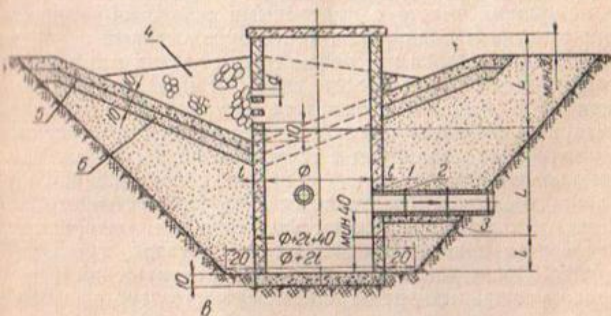
Рис. 12. Колодцы:
