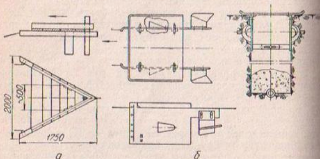
Рис. 72. Схема присыпателей:
