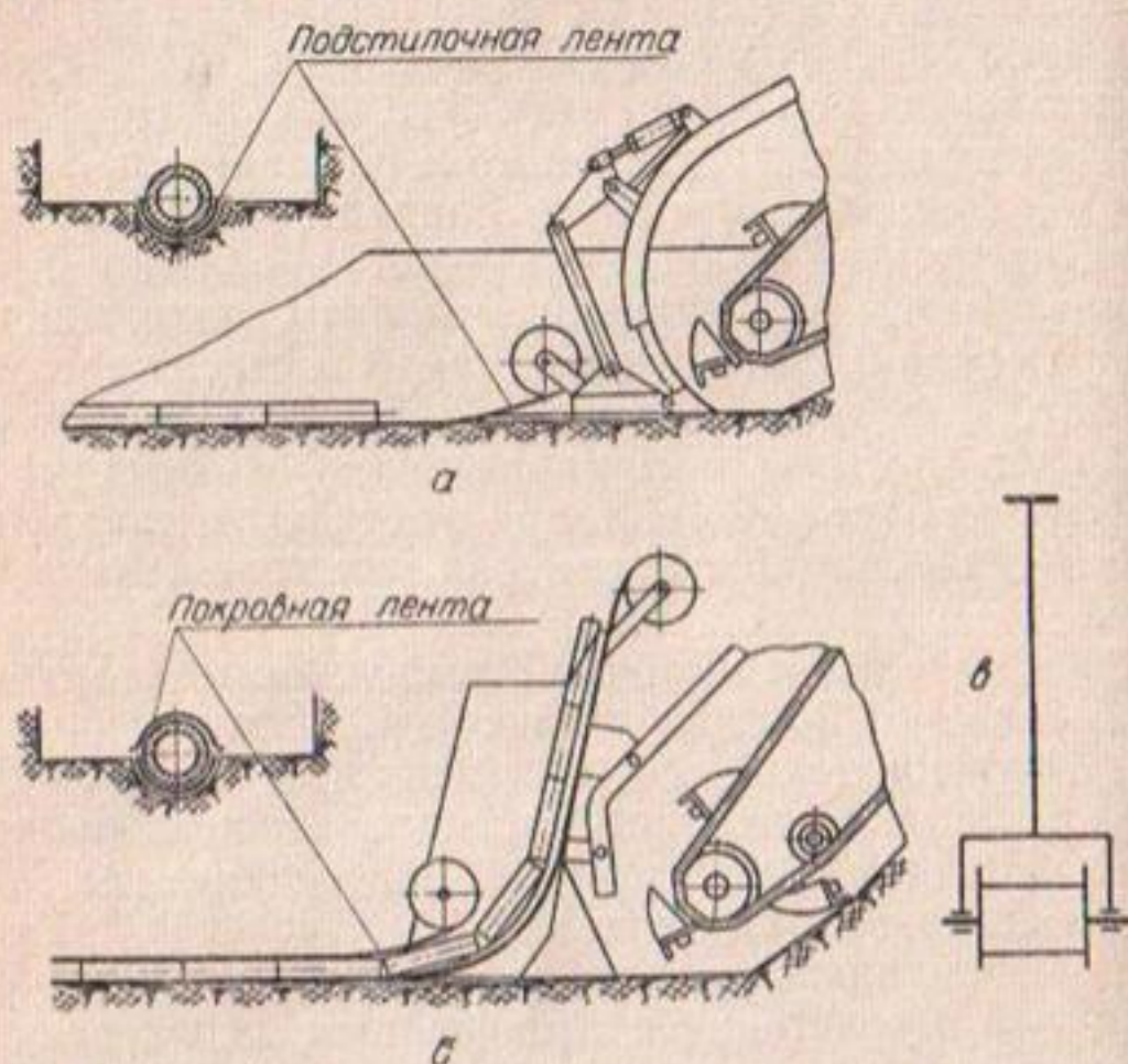
Рис. 65. Схема защиты труб рулонным материалом:
