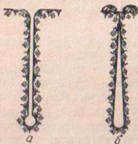
Рис. 4. Земляной дренаж: а — кротовый и б — щелевой.
