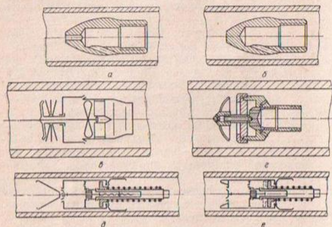
Рис. 80. Гидравлические головки для очистки дрен:
