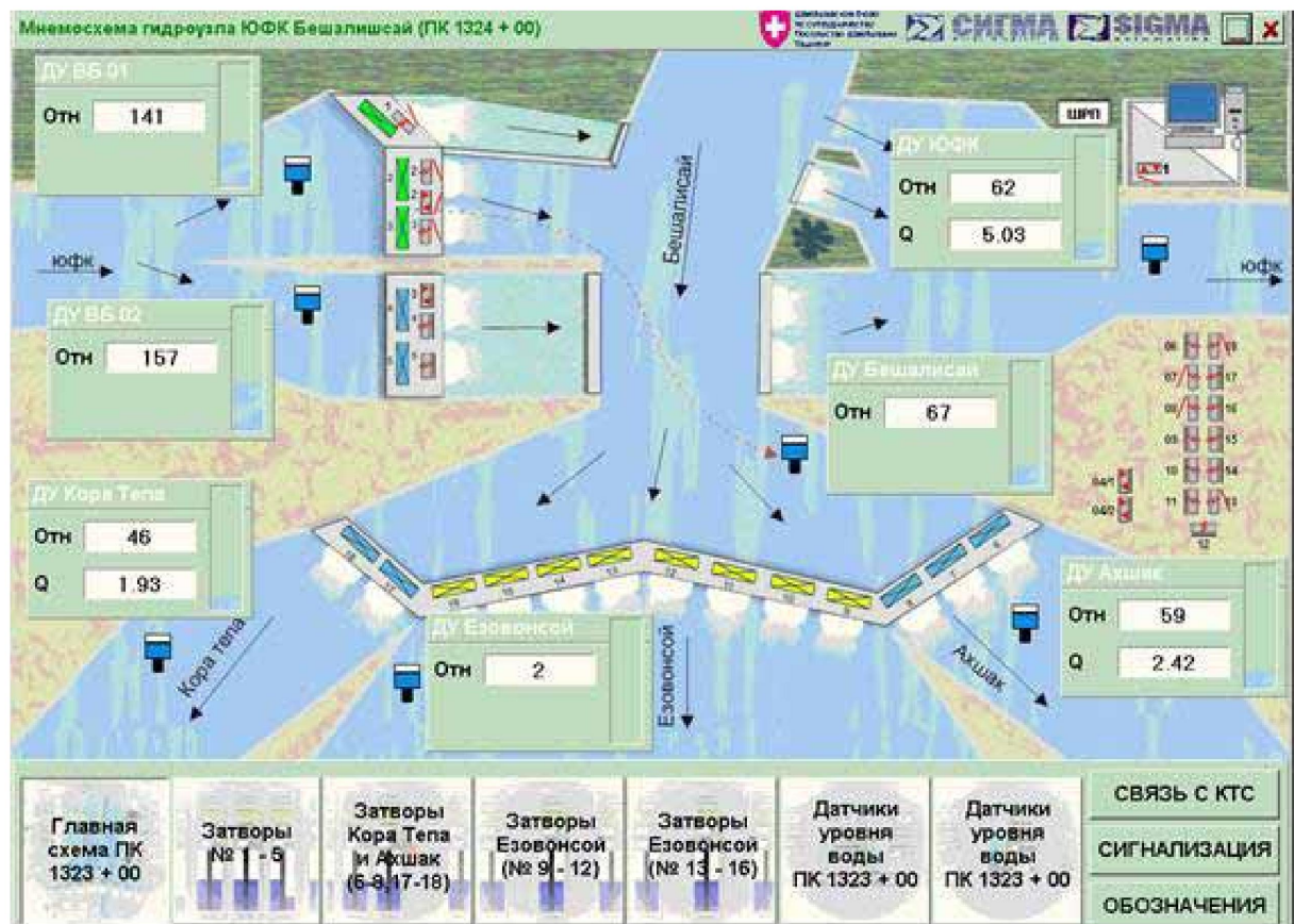
Рис.16. Сооружение Хамза главная мнемосхема системы SCADA
