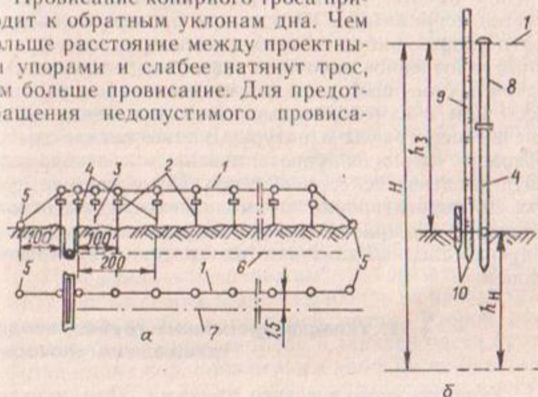
Рис. 45. Установка копирного троса на фиксирующие упоры:
