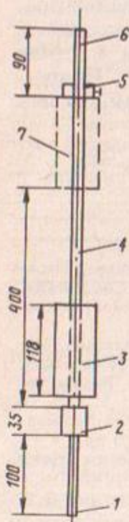
Рис. 57. Ударник ДорНИИ:
