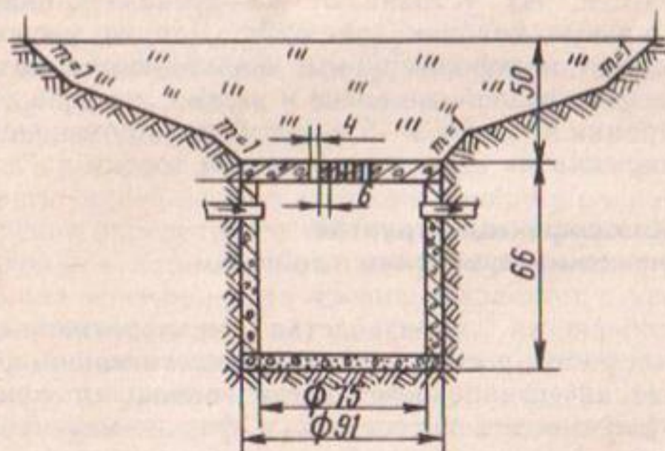
Рис. 21. Поглощающий колодец:
