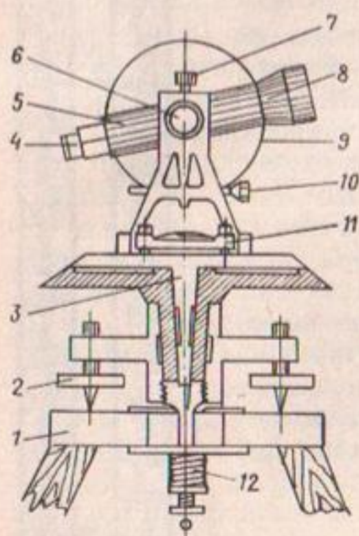
Рис. 4. Теодолит:
