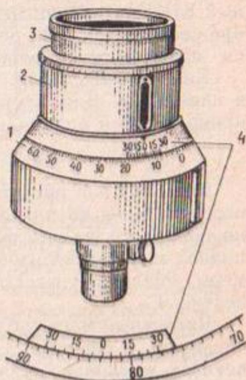
Рис. 6. Гониометр:
