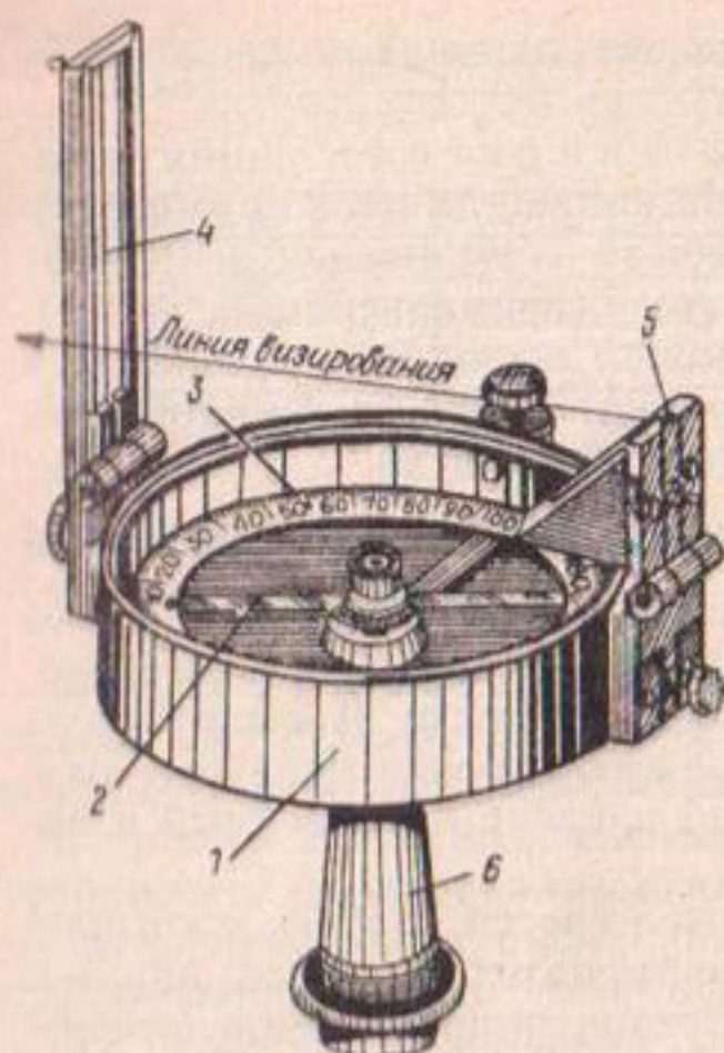
Рис. 5. Буссоль:
