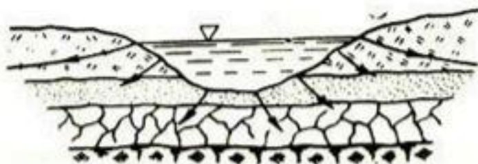
Рис. 8-8. Схема фильтрации через дно и борта водохранилища.
