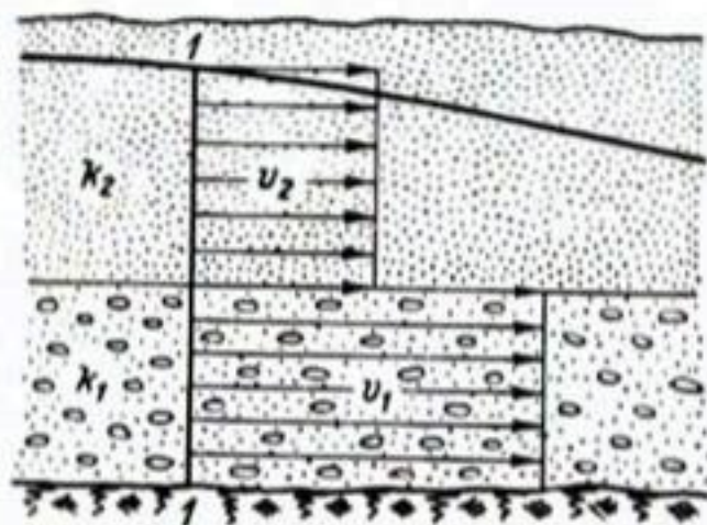
Рис. 2-7. Эпюра скоростей фильтрации в слоистом пласте.
