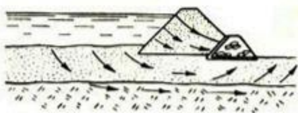
Рис. 8-7. Схема фильтрации из водохранилища через тело и основание плотины.
