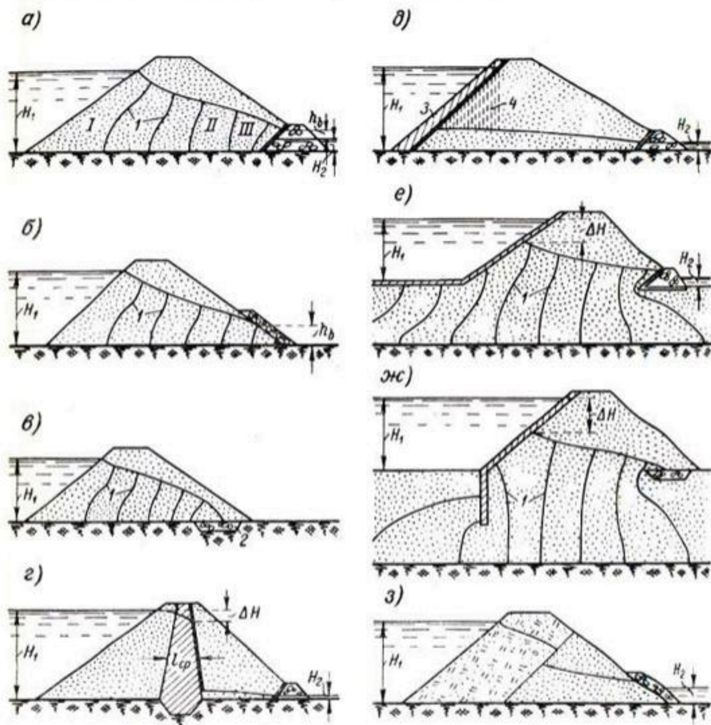
Рис. 3-22. Схемы фильтрации в земляных плотинах: а — на непроницаемом основании; б — с наклонным дренажем; в — с тюфячным дренажем; з — в земляной плотине с ядром; д — с экраном; е — с экраном и понуром; ж — с экраном и зубом; з — смешанного типа.
