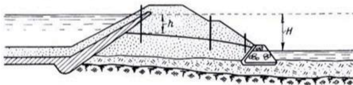
Рис. 3-10. Пьезометрический створ в земляной плотине с экраном.
