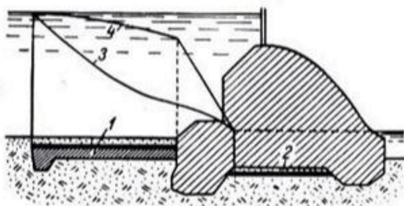
Рис. 8-23. Схемы эпюр напоров в плотине из непроницаемого и относительно сильнопроницаемого бетона.
