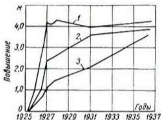
Рис. 8-33. Изменение уровней грунтовых вод в створе на оросительной системе Голодной степи на различных расстояниях от канала. 1 — 340 м; 2 — 2700 м; 3 — 4330 м.
