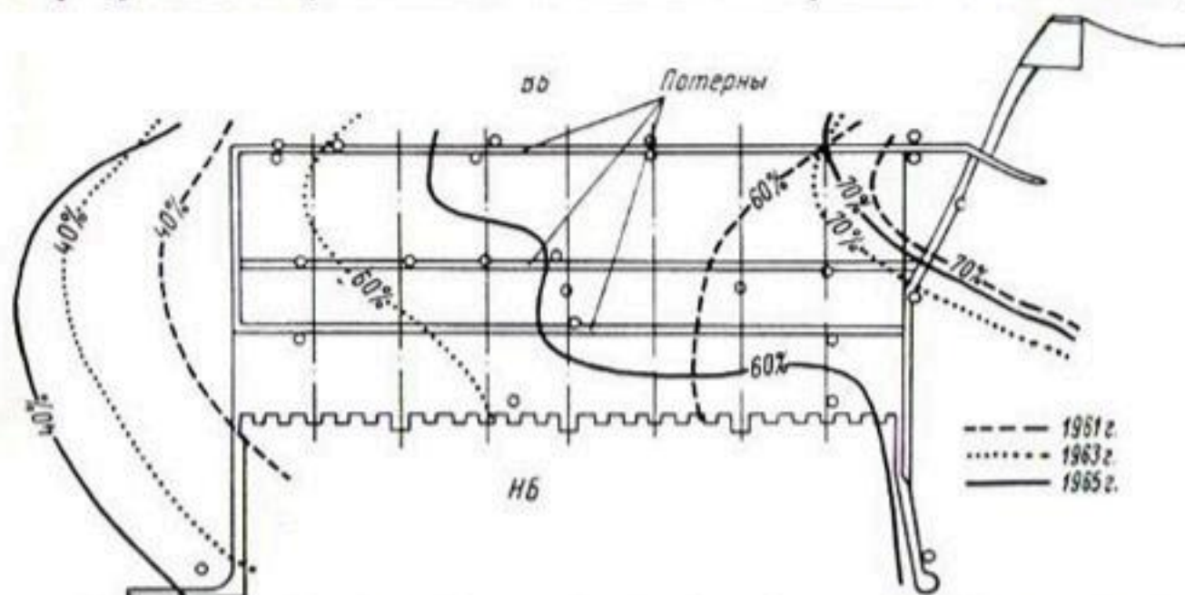
Рис. 3-20. План гидроизопьез нижне-соликамского горизонта Камской ГЭС.
