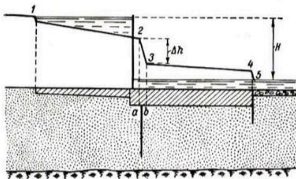
Рис. 8-30. Флютбет с исследуемой шпунтовой стенкой. 1, 2, 3, 4, 5 — эюра напоров по контуру флютбета.
