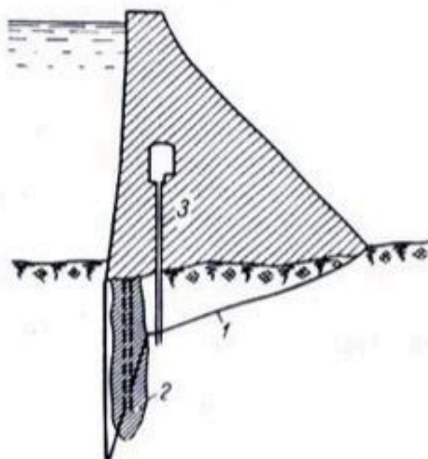
Рис. 8-25. Эпюра приведенного противодействия плотины. 1 — эпюра противодействия; 2 — завеса; 3 — дренаж.
