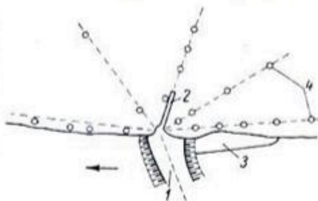
Рис. 3-6. Схема лучевого расположения пьезометров в береговом примыкании.
