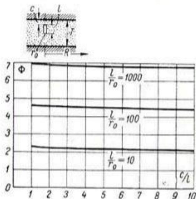
Рис. 5-5. Зависимость фильтрационного сопротивления несовершенной скважины от отношения c/l .
