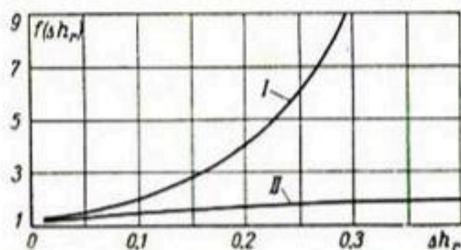
Рис. 8-19. Определение рационального режима работы дренажа.
