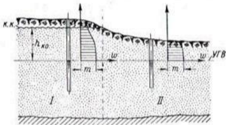
Рис. 6-3. Схематическое изображение влияния рельефа местности на величину коэффициента водоотдачи (коэффициент водоотдачи капиллярной каймы m_n' ).
