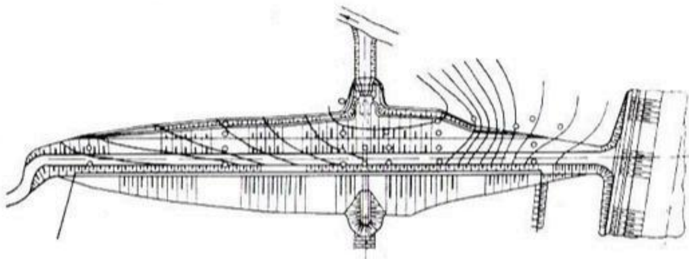
Рис. 9-7. Гидроизогинсы в земляной плотине с экраном.
