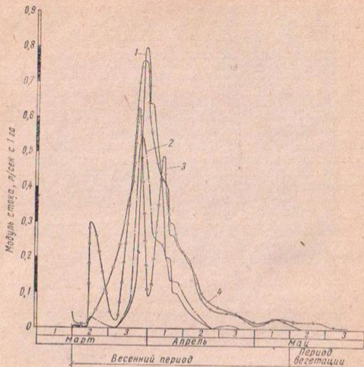
Рис. 27. Работа дрена из различных материалов:
