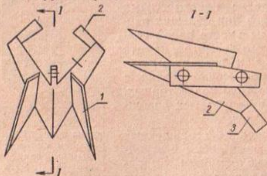
Рис. 22. Обжим-рыхлитель:
