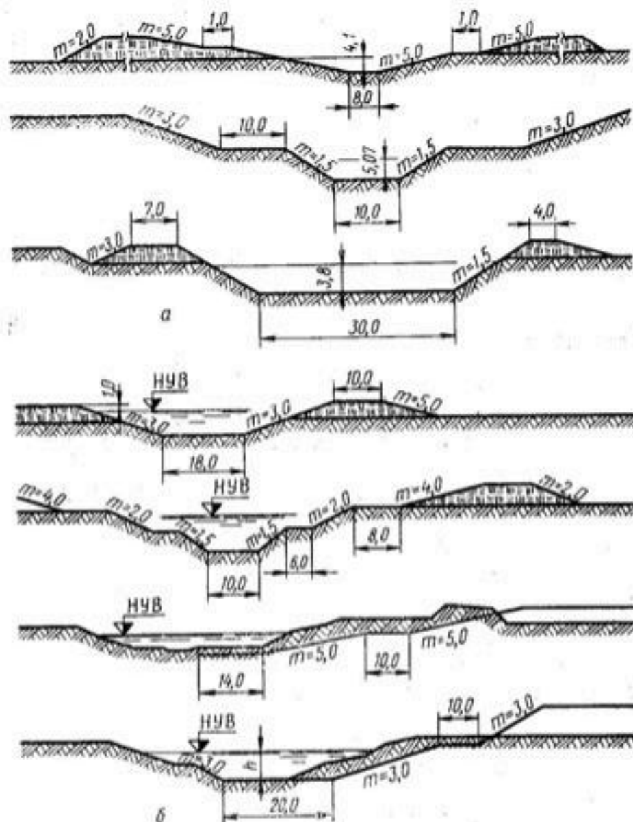
Рис. 13. Типовые поперечные сечения Амубухарского канала: а — I очередь; б — II очередь. (Размеры в м).
