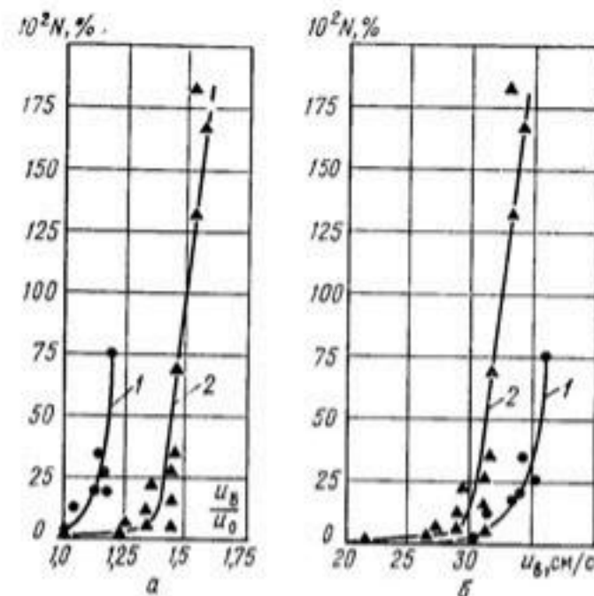
Рис. 43. Зависимости характеристики N от относительной скорости u_w/u_0 (а) и средней скорости на вертикали u_w (обозначения те же, что и на рис. 42).
