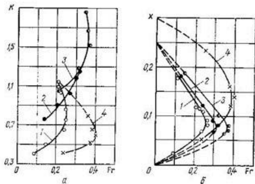
Рис. 47. График зависимости k=k(Fr) (а) и x=x(Fr) (б): 1, 2, 3 — песчаное дно ( d_{cp}=0,21 мм) с уклонами соответственно I=0,0012 , I=0,0025 и I=0,005 ; 4 — дно, сложенное из мелкой гальки ( d_{cp}=5,2 мм), I=0,0025 .
