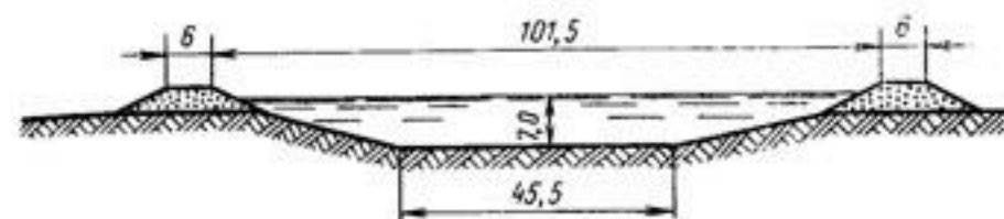
Рис. 17. Типовое поперечное сечение Донского магистрального канала. (Размеры в м).
