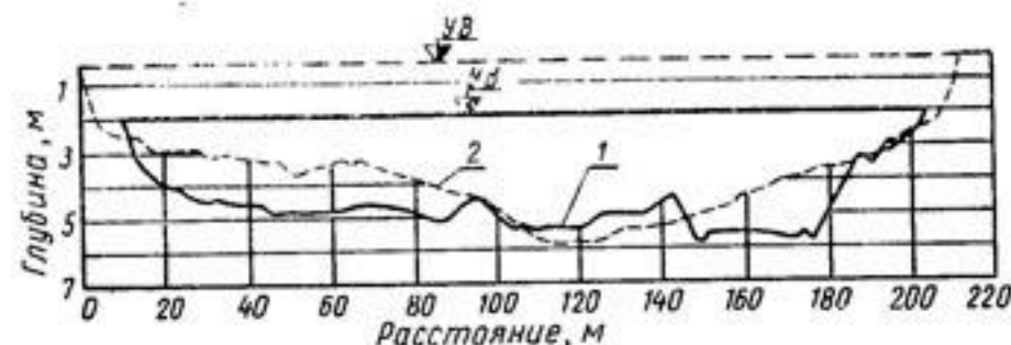
Рис. 37. Переформирование живого сечения Каракумского канала (223 км), сложенного мелкопесчаными грунтами, после землеразработных работ:
