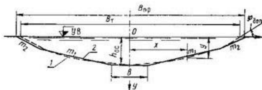
Рис. 55. Схема поперечного сечения канала, принятая В. П. Троицким при уточнении метода влекущей силы: 1 — теоретическое сечение; 2 — проектное. ( B_T , B_{пр} — ширина соответственно теоретического и проектного сечений канала).
