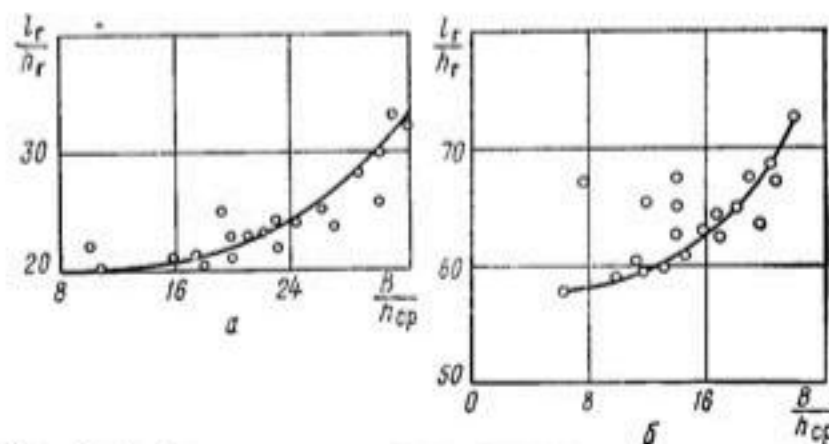
Рис. 46. График зависимости l_r/h_r = f(B/h_{cp}) для несвязного (а) и связного (б) грунтов.
