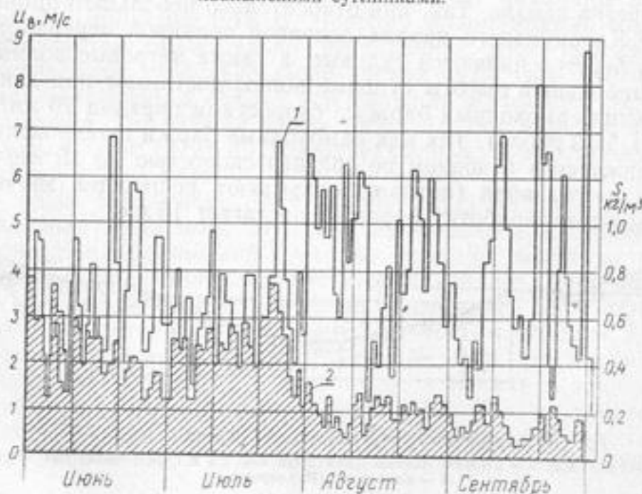
Рис. 7. Совмещение графика скорости ветра v_w (1) и средней мутности потока s (2) в Правоегорлыкском канале (по данным Н. И. Кириенко).
