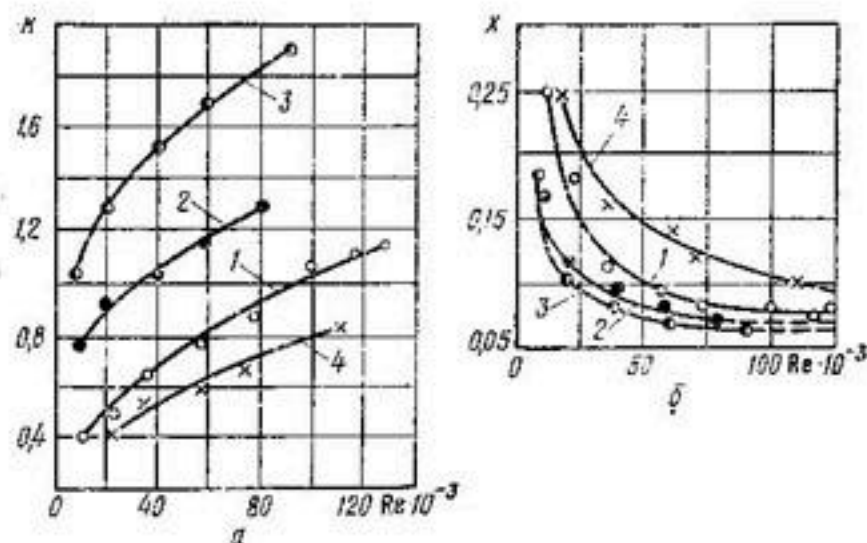
Рис. 48. График зависимости k=k(Re) (а) и x=x(Re) (б) (обозначения те же, что и на рис. 47).
