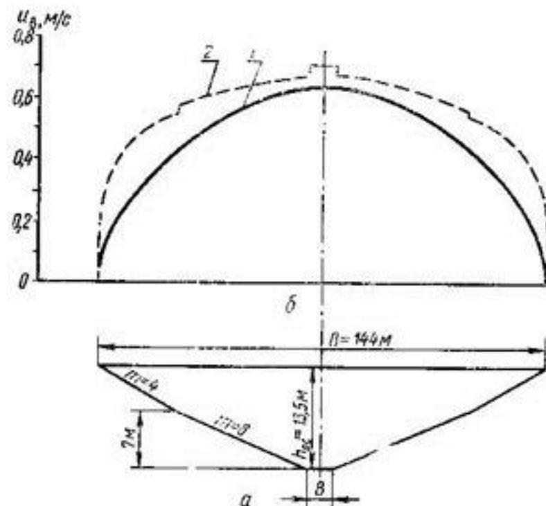
Рис. 56. Поперечный профиль канала (а) в мелкопесчаных грунтах, рассчитанный по методу эпюр скоростей (б) при расходе воды Q=600 \text{ м}^3/\text{с} :
