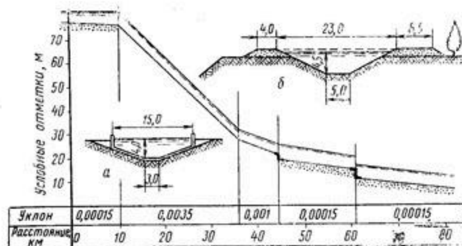
Рис. 11. Продольный профиль и поперечные сечения бетонного (а) и земляного (б) русла Большого Андижанского канала. (Размеры в м).
