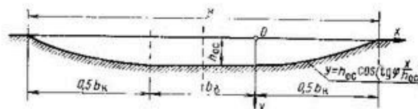
Рис. 54. Безмерный профиль живого сечения канала, рассчитанный по методу влекущей силы: b_v — ширина вставки.
