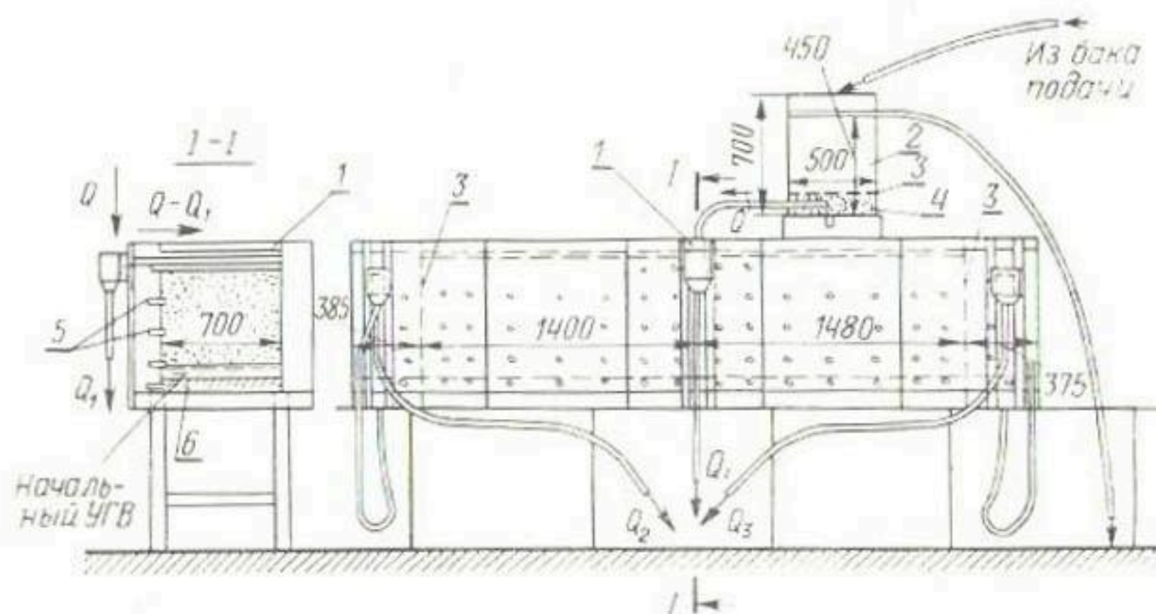
Рис. 43. Схема опытной установки:
