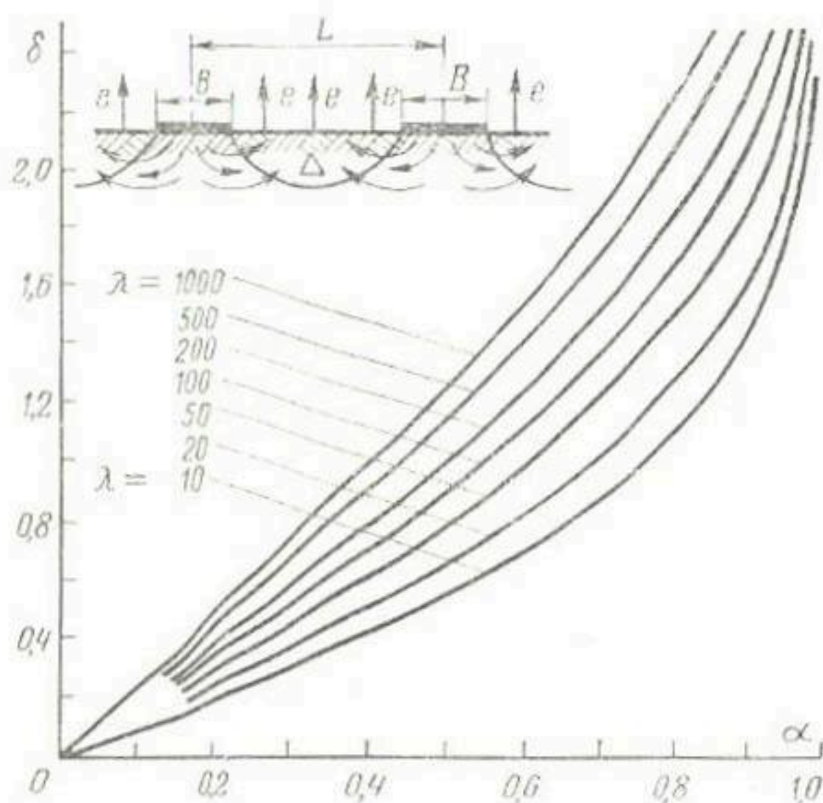
Рис. 13. Влияние изменения уровня грунтовых вод на фильтрацию из канала с учетом испарения. Коэффициент уменьшения потерь \alpha находится по графику в зависимости от \lambda = L/B и \delta = \Delta/B .
