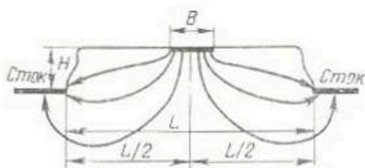
Рис. 4. Схема к расчету фильтрации из канала при симметрично расположенных понижениях и глубоком залегании водоупора.
