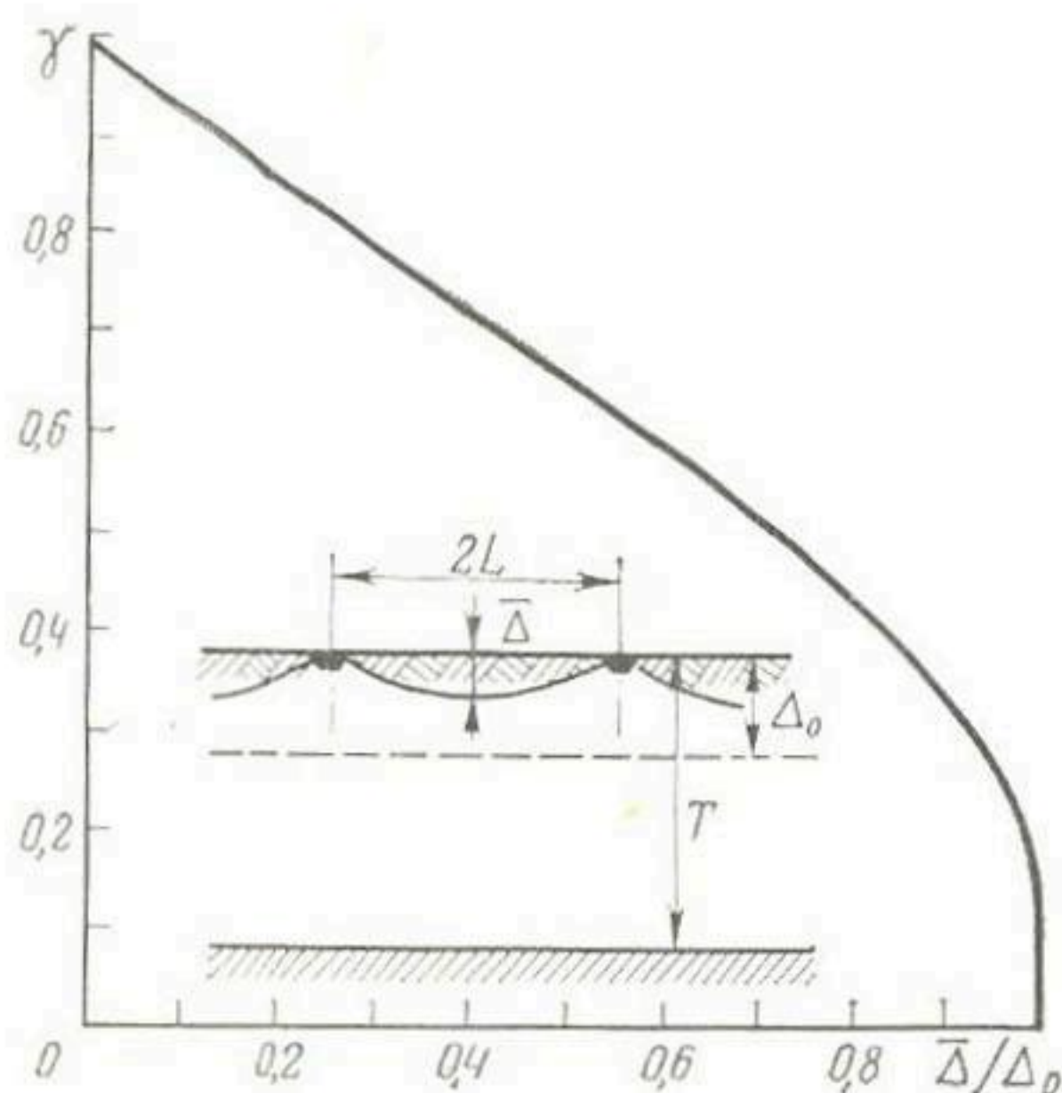
Рис. 17. Зависимость между \bar{\Delta}/\Delta_0 и \gamma (подземный отток отсутствует, потери расходуются на испарение).
