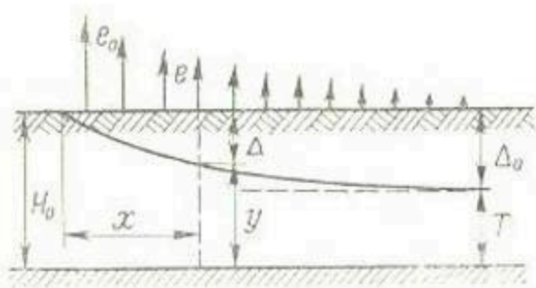
Рис. 14. Схема к расчету фильтрации из канала, расходуемой на испарение с поверхности грунтовых вод.
