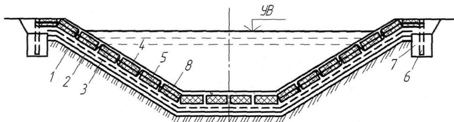
1 – грунт подстилающего основания; 2 – геомембрана; 3 – геотекстиль; 4 – габионы; 5 – канат; 6 – металлическая стойка; 7 – монолитный бетон; 8 – кольматирующий слой.
