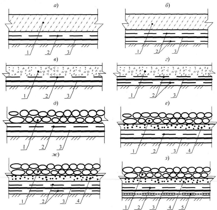
а, б – с геомембраной и защитным покрытием из бетона; в, з – с геомембраной и защитным покрытием из грунта; д – з – с геомембраной и защитным покрытием из каменной наброски; 1 – защитное покрытие; 2 – защитная прокладка из геотекстиля; 3 – противofильтрационный элемент из геомембраны; 4 – защитный слой из песка; 5 – дренажный элемент из геокомпозита; Рис 2. Усовершенствованные конструкции противofильтрационных облицовок каналов и водоемов с использованием геосинтетических материалов
