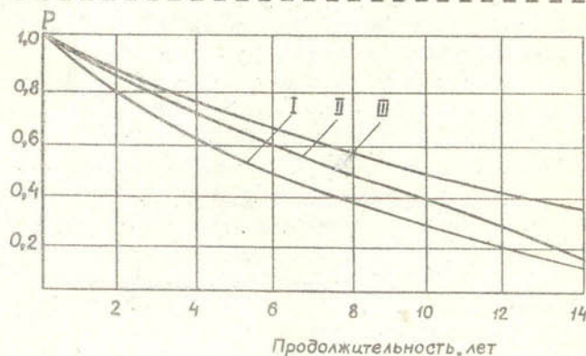
Рис. 3. Распределение вероятности безотказной работы дрена различных конструкций
