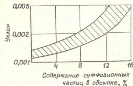
Рис. 5. Область допустимых отклонений конструктивных параметров дренажной системы, позволяющая установить периодичность и объем обследований.
