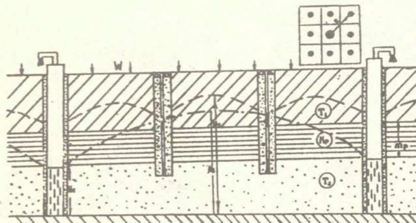
Рис. 4.1а. Схема вертикального дренажа с усилителями перетекания.
