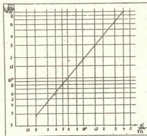
Рис. 4.1б. График зависимости h_r \sqrt{\frac{4K_1}{W}} = f\left(\frac{b}{\sqrt{n}}\right)
