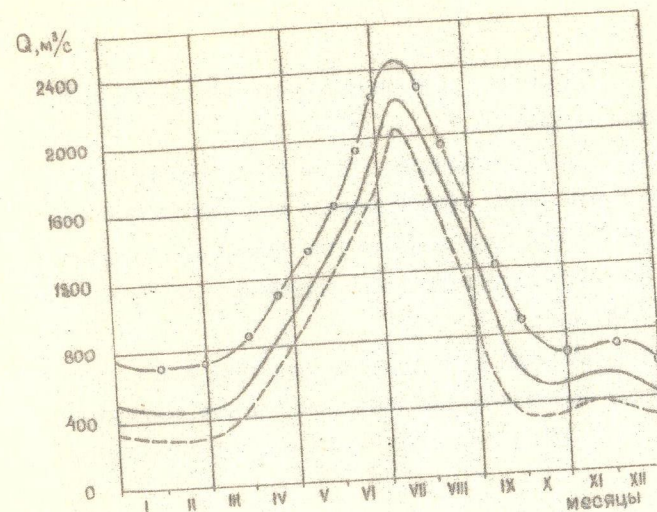
Рис. 1. Изменение осредненного значения расхода воды в створе Туямуви с 1974 по 1984 гг. —○— многоводный ( P = 20\% ), ——— средний по водности ( P = 50\% ), - - - маловодный ( P = 95\% )
