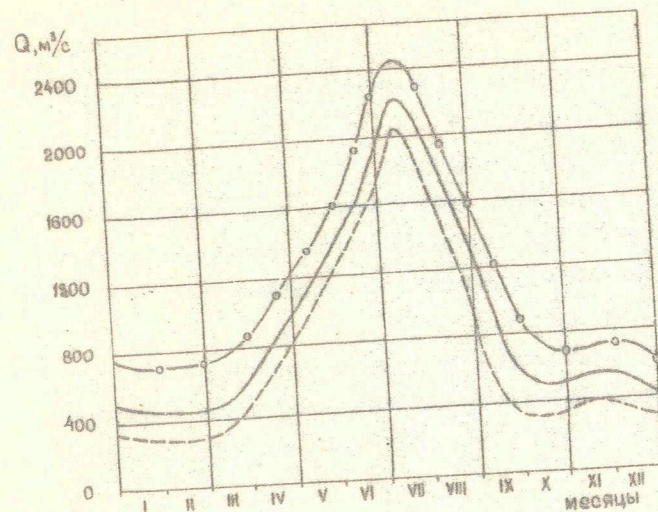
Рис. 1. Изменение среднего значения расхода воды в створе Туямуви с 1974 по 1984 гг. о—о многоводный ( P = 20\% ), ——— средний по водности ( P = 50\% ), - - - маловодный ( P = 95\% )
