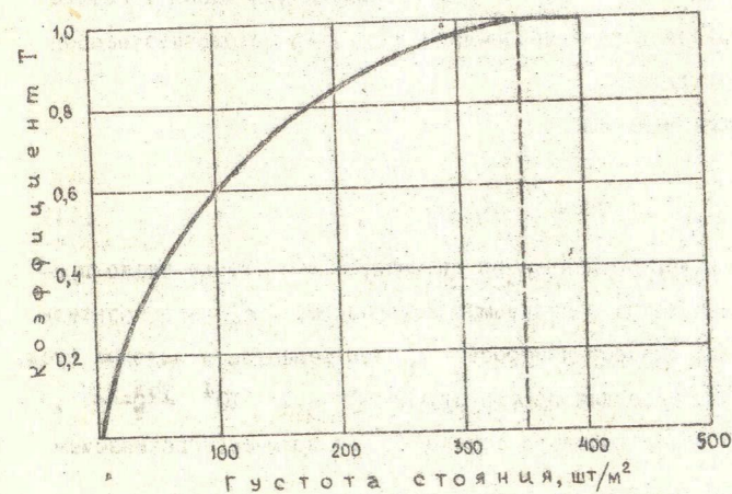
Рис. 5. Коэффициент Т в зависимости от густоты стояния тростника на биоплато
