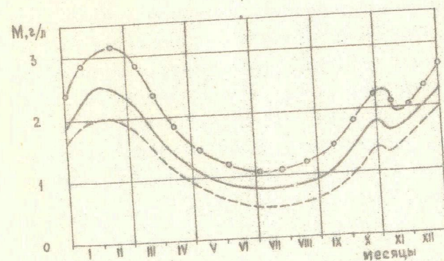
Рис. 2. Прогнозное изменение минерализации воды в Амударье в створе Туямуви о—о многоводный ( P = 20\% ), ——— средний по водности ( P = 50\% ), - - - маловодный ( P = 95\% )
