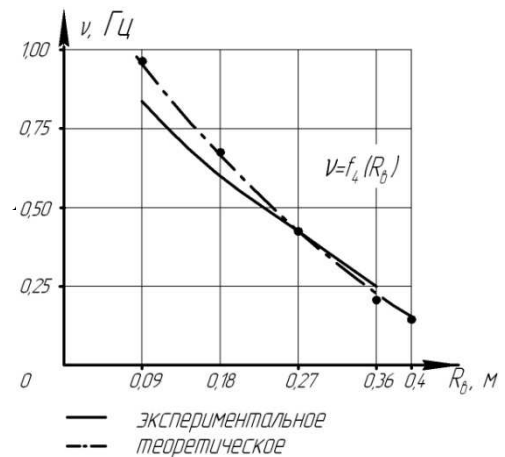
Рисунок 8 – График функции \nu = f_4(R_b) при \alpha = 10^\circ
