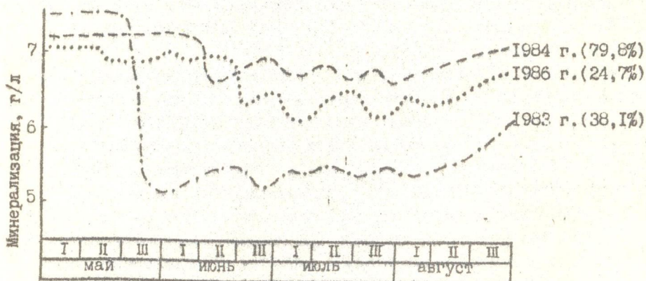
Рис. I. Динамика минерализации поверхностных слоев грунтовых вод в годы различной влагообеспеченности при поливах нормой 500 м 3 /га, пороге предполивной влажности 70...75% от НВ, УГВ=3,0 м.
