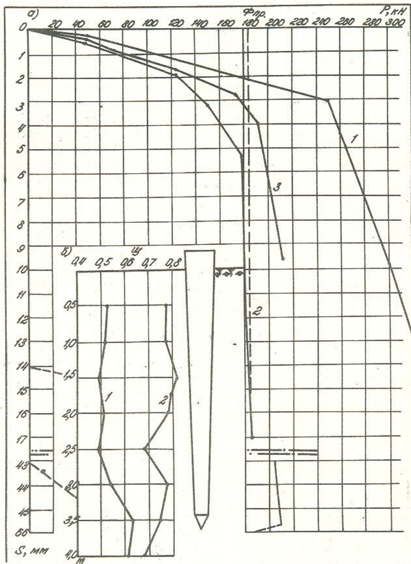
Рис. 3. Графики S=f(P) испытаний несущей способности клиновидной свай: а) 1 - по ускоренной методике без замачивания; 2, 3 - по стандартной и ускоренной методикам в замоченном грунте; б) значения степени влажности грунта w по глубине
