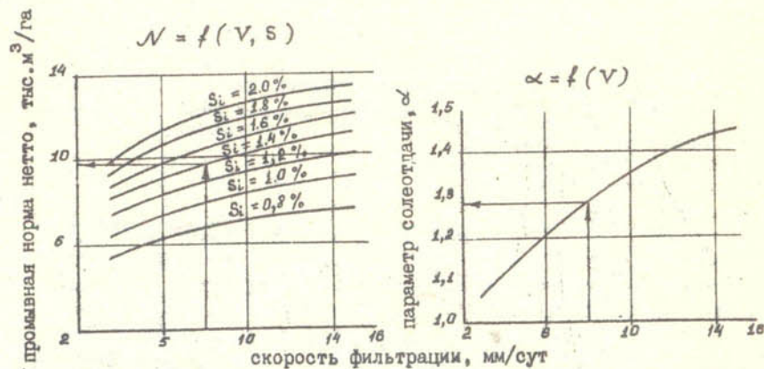
Рис.6 Зависимость параметра засоленности ( \alpha ) от скорости фильтрации ( V )
