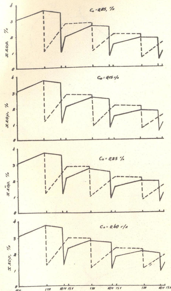
Рис. 6 Прогноз солевого режима орошаемых земель — весенняя влагозарядка, --- осенняя влагозарядка C_n — минерализация оросительной воды по хлору, \text{г/г} Баланс поверхностно-грунтовых и почвенных вод
