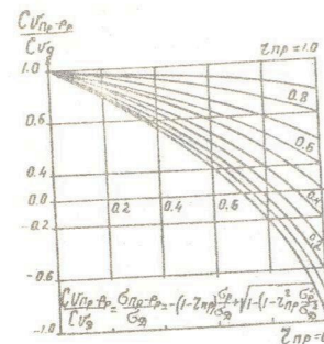
Рис. 3. График зависимости отношения коэффициентов вариации разности равнообеспеченных величин приходной ( \Pi ) и расходной ( P ) частей баланса и результирующей величины баланса ( \mathcal{D} ) от отношения среднеквадратических отклонений расходной ( P ) и результирующей величины баланса.
