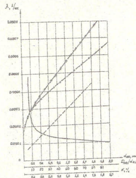
Рис.2. Зависимость интенсивности отказов электронасосов от литологии, состава гравийной обсыпки и пескования скважин в момент пуска. — \lambda_{50} , — \lambda_{50} < 0,20 , — \lambda_{50}/d_{50} , — \lambda_{50} > 0,20
