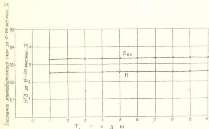
Рис.3. Динамика основных показателей мелиоративного состояния земель Джетысайского района при поддержании "критической" дренированности - 2900 м³/га ( n = 270 шт., КПРС = 0,45, Q_t = 0,42 л/с).
