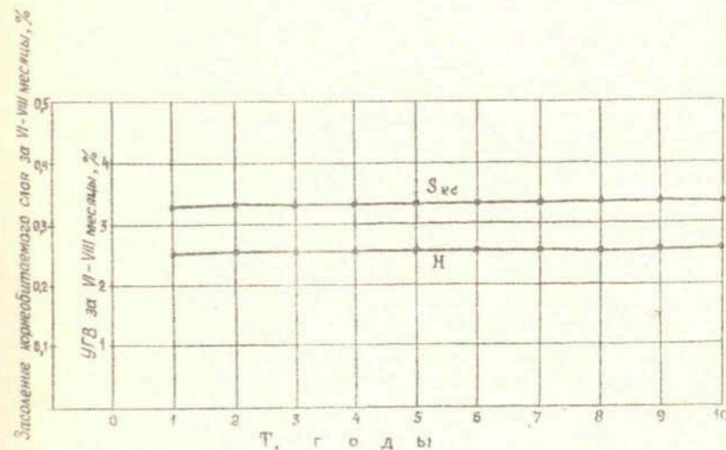
Рис.3. Динамика основных показателей мелиоративного состояния земель Джетысайского района при поддержании "критической" дренированности - 2900 м³/га ( \rho = 270 шт., КПРС = 0,45, Q_t = 0,42 л/с).
