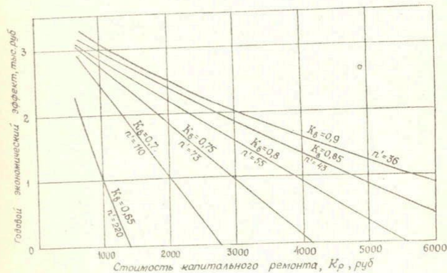
Рис.5. Изменение экономической эффективности очистки фильтра от кольматации в зависимости от стоимости капитального ремонта (на примере СВД в Джетысайском районе).
