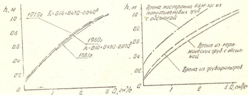
Рис.5. Зависимости Q=f(h) : а) для дрены из трубо-фильтров (за 3 года эксплуатации); б) то же в сопоставлении с дренажной из керамических труб с обсыпкой.
