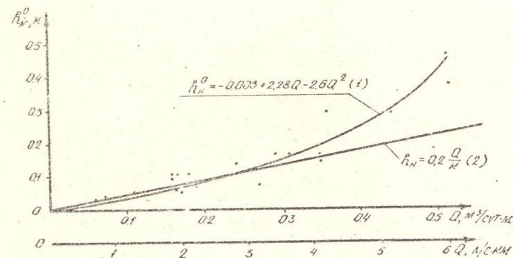
Рис.6. Зависимость действующего напора по оси дрены из трубофильтров от фильтрационного расхода (1) - по фактическим данным, (2) - теоретическая.
