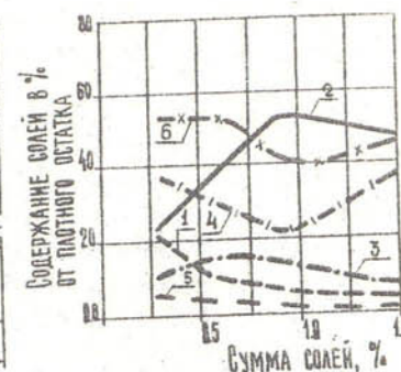
Рис. 2. Изменение состава солей при различных степенях опреснения почв: 1 - \text{Ca}(\text{HCO}_3)_2 ; 2 - \text{CaSO}_4 ; 3 - \text{MgSO}_4 ; 4 - \text{Na}_2\text{SO}_4 ; 5 - \text{NaCl} ; 6 - сумма токсичных солей.
