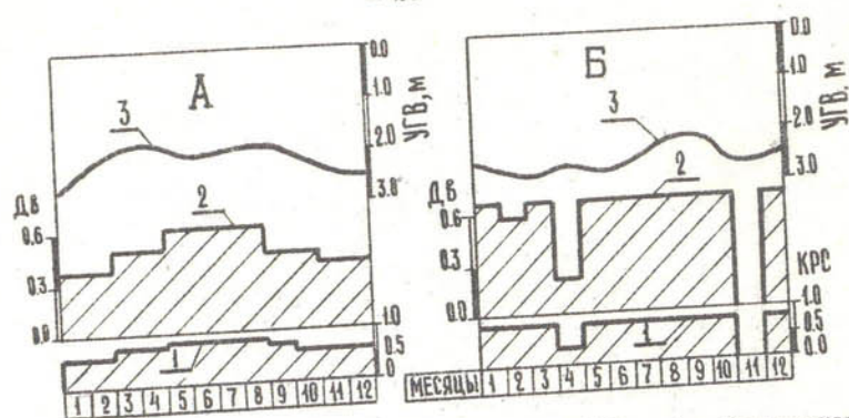
Рис. 6. Показатели режимов откачек из СВД: А - Багдадского района; Б - Кировского района; 1 - КРС; 2 - прогнозный объем откачиваемых вод ( D_в ), m^3/ga ; 3 - глубина грунтовых вод, м.
