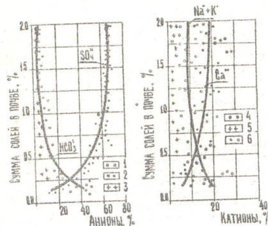
Рис. 3. Зависимость содержания относительных величин отдельных анионов и катионов в почве: 1 - \text{HCO}_3 ; 2 - \text{SO}_4 ; 3 - \text{Cl} ; 4 - \text{Ca} ; 5 - \text{Mg} ; 6 - \text{Na} + \text{K} .
