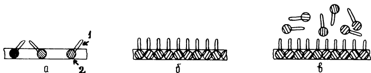
Рис. 8. Поверхностно-активные вещества:
