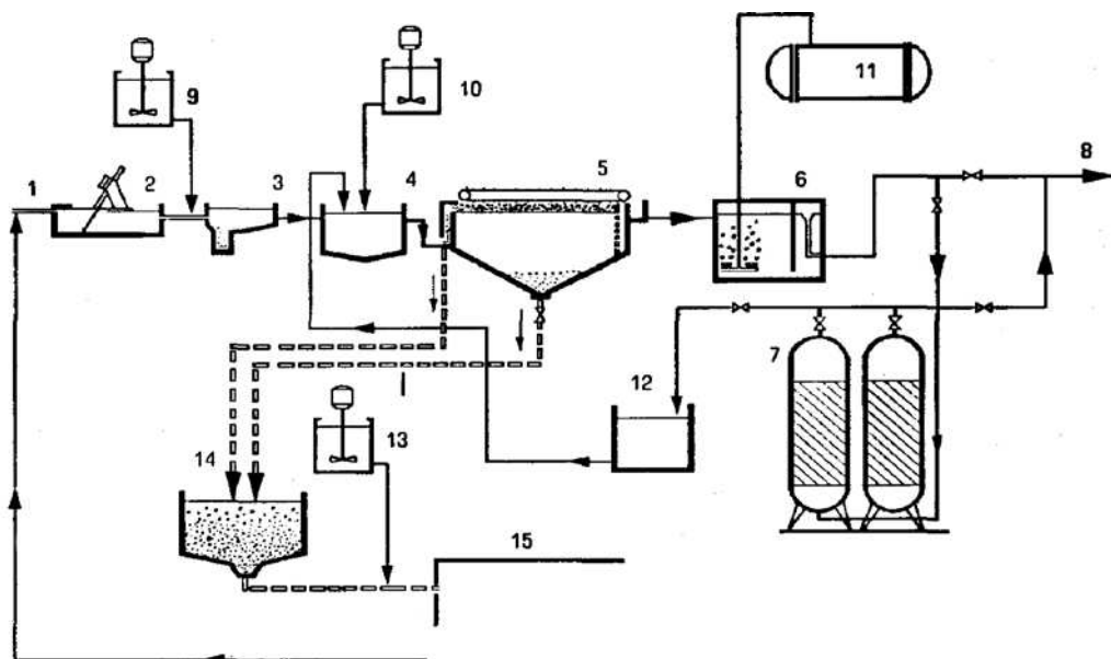
1,8 – подача сточных вод и отведение очищенной воды; 2 – решетка; 3 – песколовка; 4 – камера флокуляции; 5 – отстойник-флотатор; 6 – контактная камера; 7 – адсорбционные фильтры; 9 – подача коагулянта; 10, 13 – подача флокулянта; 11 – озонатор; 12 – резервуар грязных промывных вод; 14 – уплотнитель осадка; 15 – фильтр-пресс
