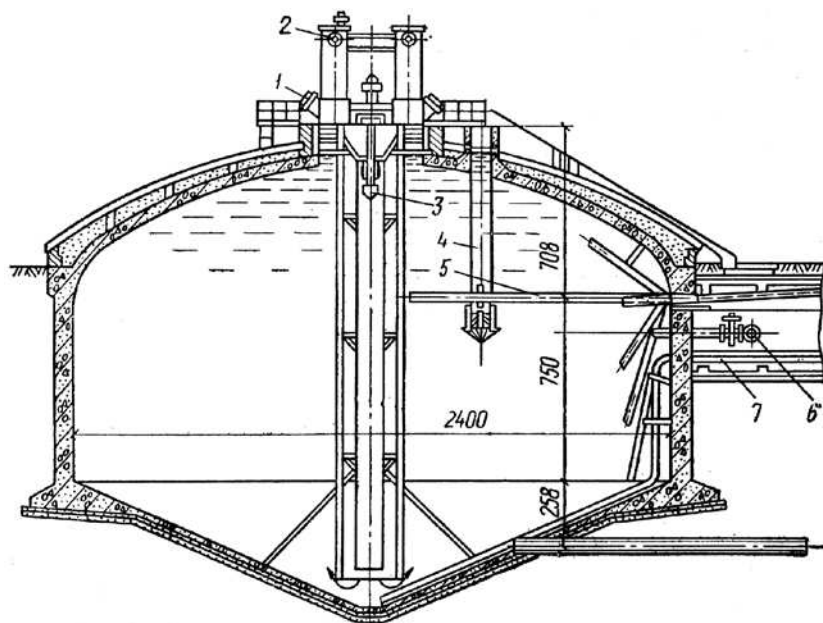
Рисунок 7.2. Метантенк с неподвижным незаопленным перекрытием станции аэрации
