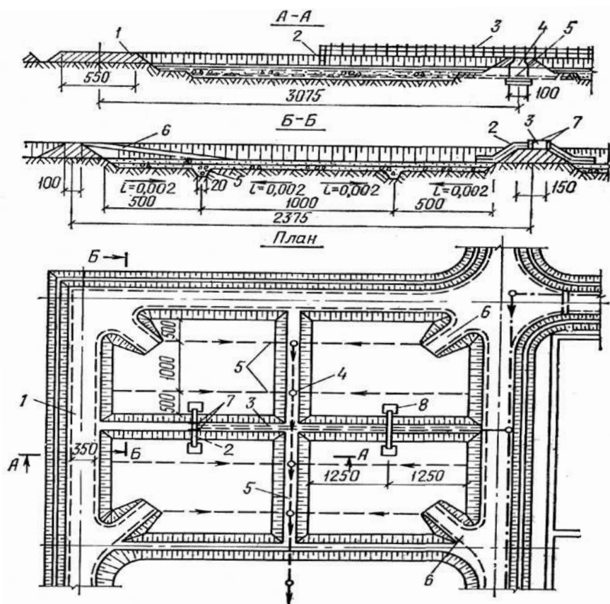
Рисунок 7.3. Иловые площадки
