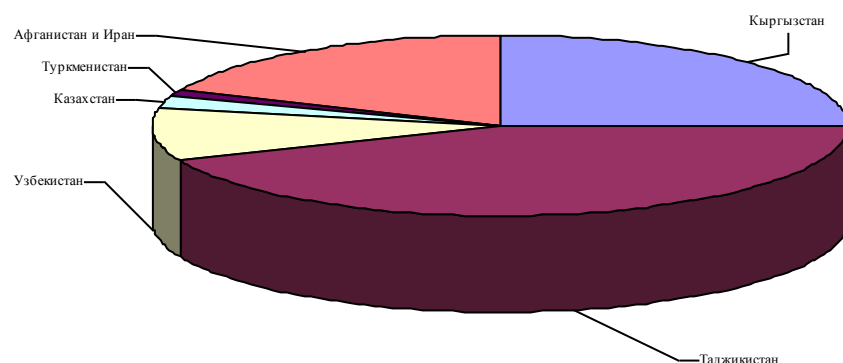
Речной сток в бассейне р. Амударьи (среднесовокупный сток за период трех циклов водности 1934-1992 г.г., км 3 /год)
