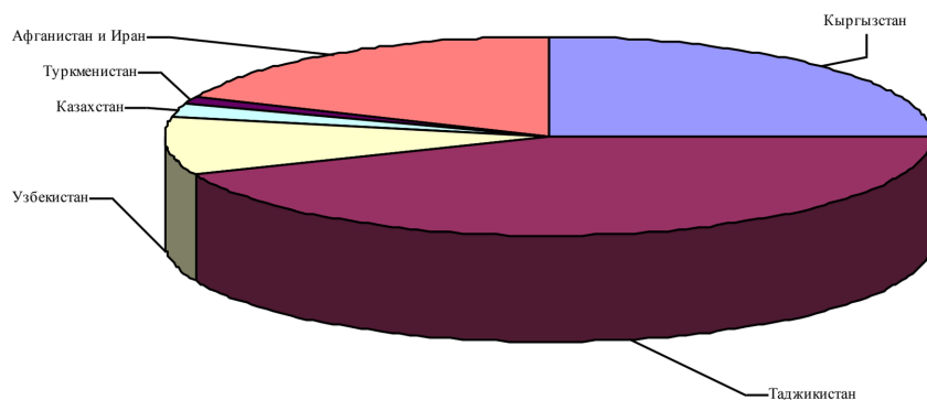
Речной сток в бассейне р. Амударьи (среднегодовое за период трех циклов водности 1934-1992 г.г., км 3 /год)
