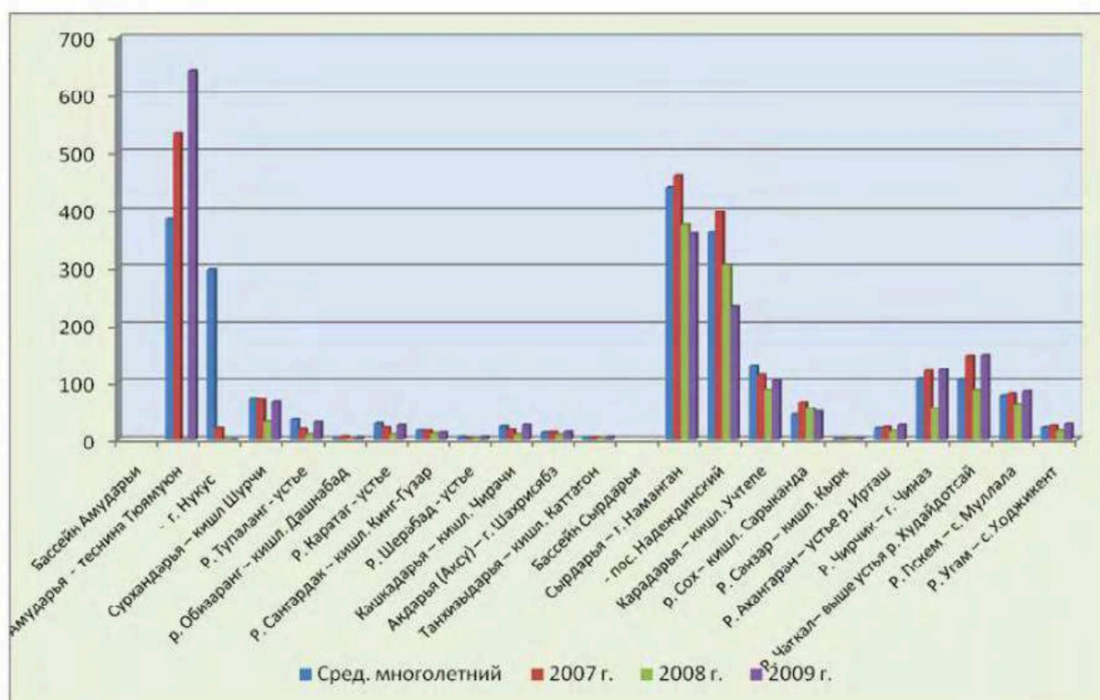
Водность речных бассейнов Амударьи и Сырдарьи, м 3 /сек.
