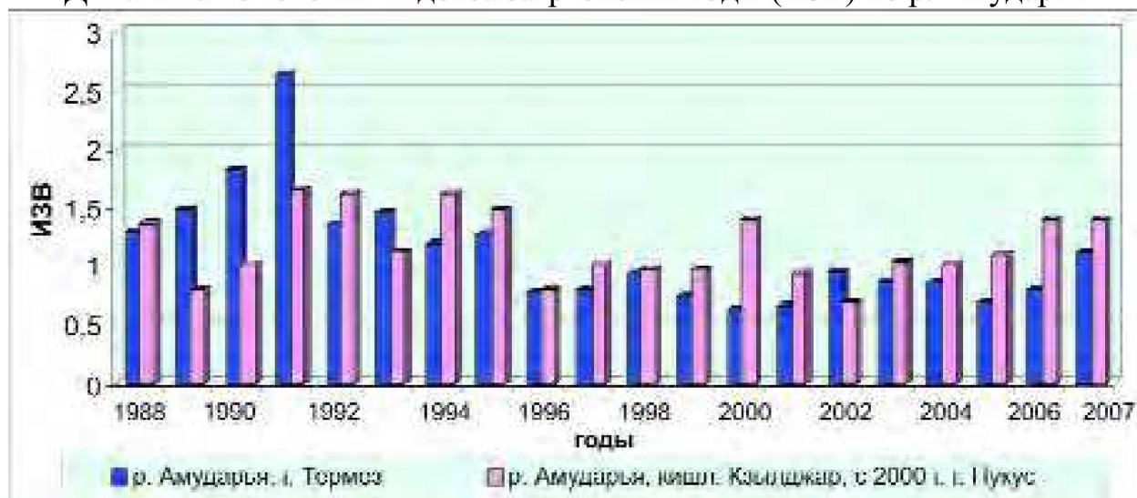
Динамика изменения индекса загрязнения воды (ИЗВ) по р. Амударья
