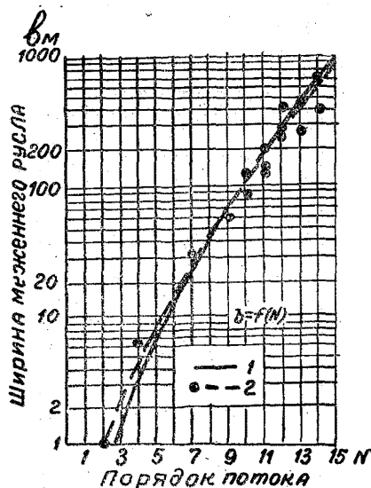
Рис. 14. Изменение ширины меженного русла в зависимости от класса реки:
