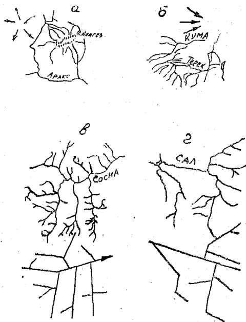
Рис. 8. Характерные рисунки речной сети: а — радиальный; б — центростремительный, в — древовидный; z — прямоугольный
