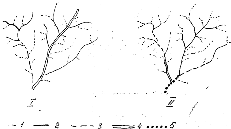
Рис. 10. Выделения порядков притоков по Хортону (I) и Ржаницыну (II): (1, 2, 3 . . . — порядок притоков)
