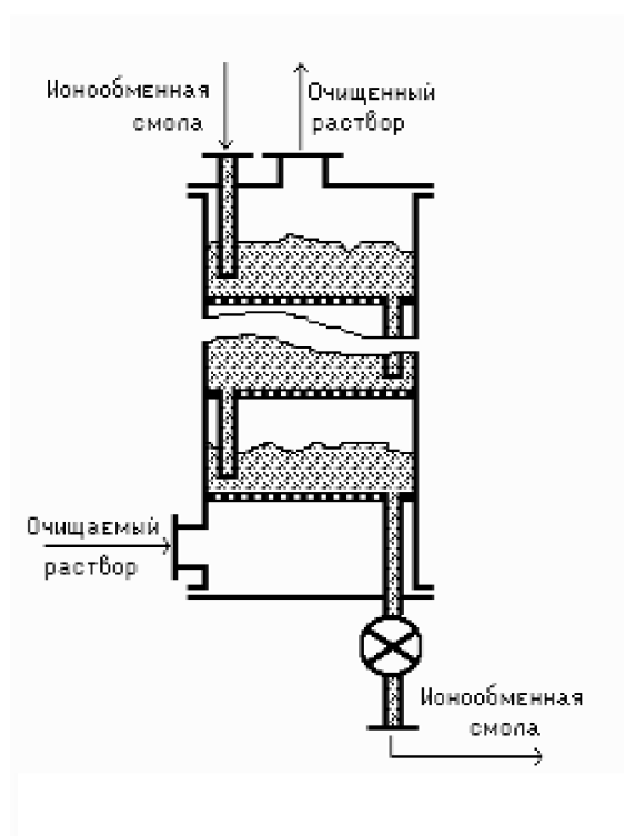
Рис. 10.2. Ионообменный аппарат с движущимся ионитом
