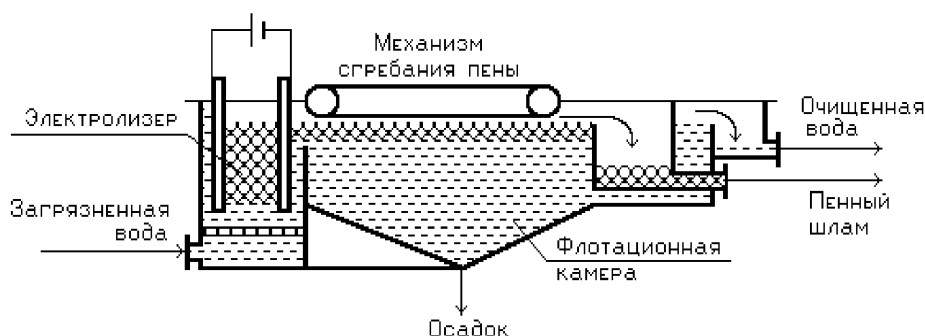
Рис. 11.1. Электрофлотатор
