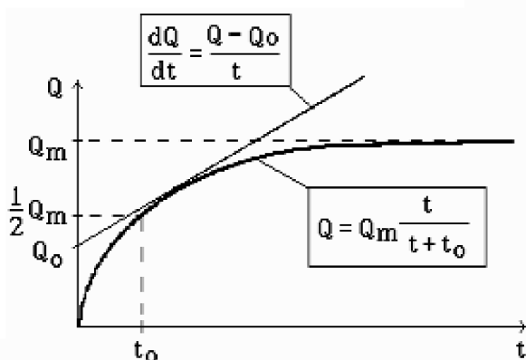
Рис. 7.1. Кривая седиментации
