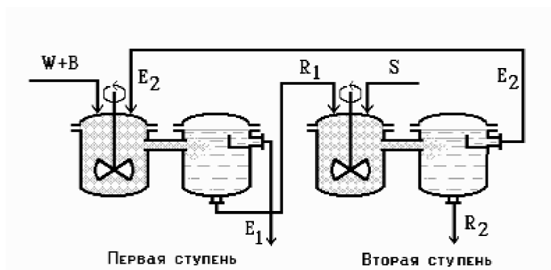
Рис. 9.6. Двухступенчатый смесительно-отстойный экстрактор
