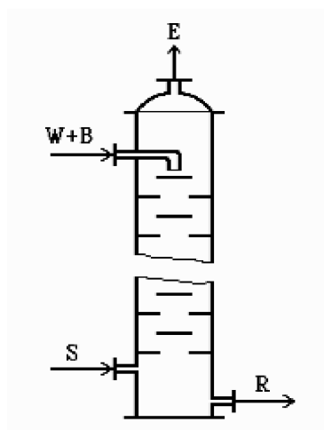
Рис. 9.8. Полочный колонный экстрактор
