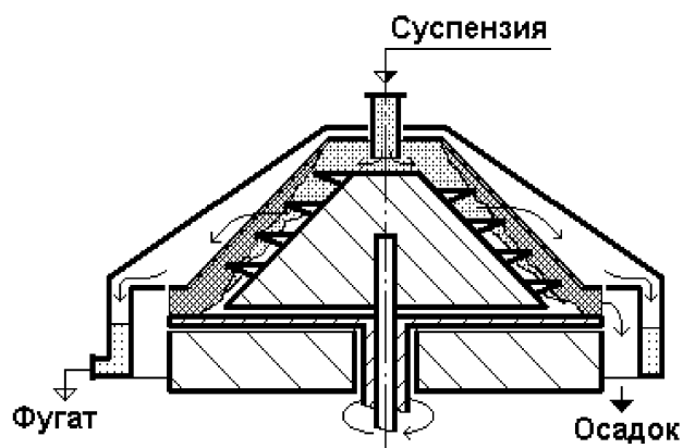
Рис. 4.5. Центрифуга с инерционной выгрузкой осадка
