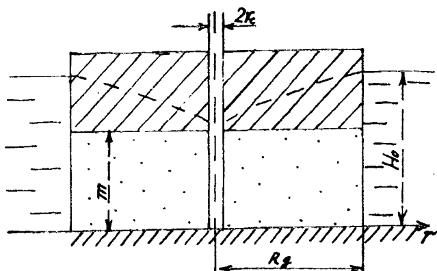
Рис. 3.8. Схема напорной фильтрации к скважине в круговом пласте
