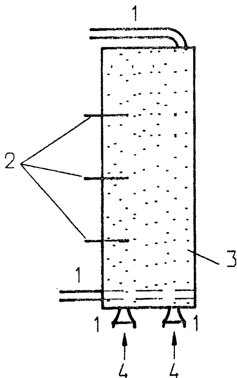
Рис. 6.16. Фильтрационная колонка для проведения индикаторных опытов с песчаными грунтами:
