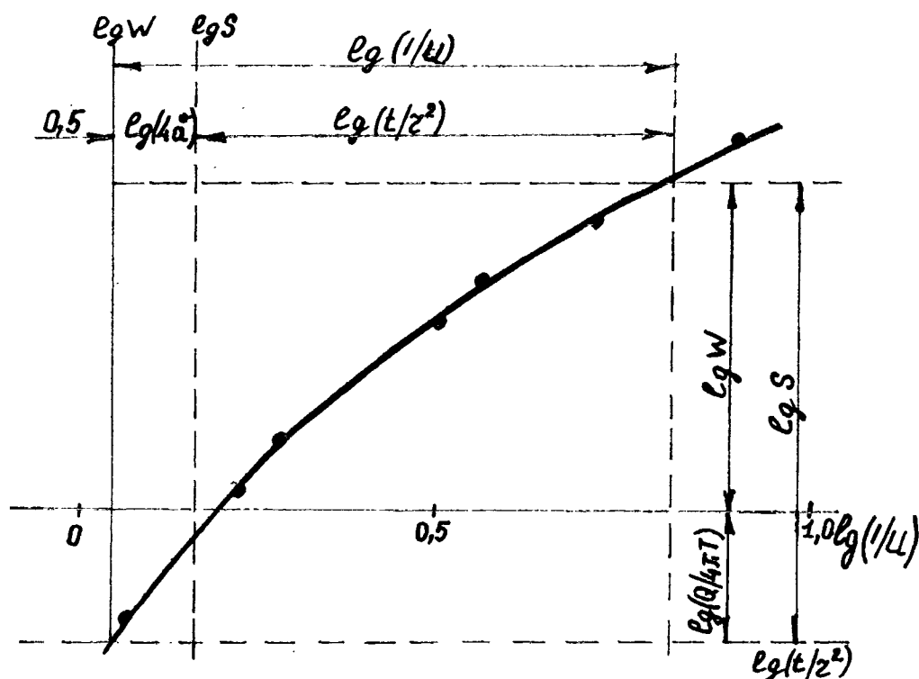
Рис. 5.17. Совмещение опытных точек ( показаны кружками ) с эталонной кривой
