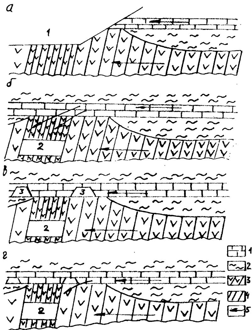
Рис. 7.6. Схемы фильтрационных потоков к горным выработкам: а - при вскрытии месторождения карьером; б-г - при подземной выемке руды; 1 - карбонатный водоносный комплекс; 2 - относительно водоупорные породы; 3 - руднокристаллический водоносный комплекс; 4 - породы рудной полосы; 5 - преобладающие направления движения подземных вод. цифрами на рисунке обозначены: 1 - карьер; 2 - подземные добычные выработки; 3 - дренажные штреки
