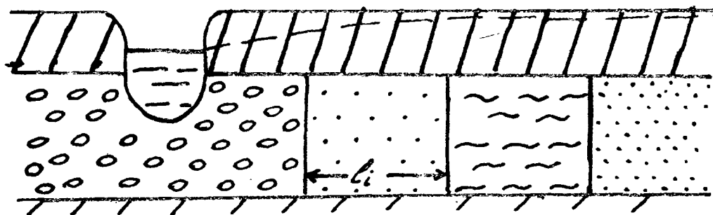
Рис. 3.5. Схема одномерной фильтрации в планово-неоднородном пласте
