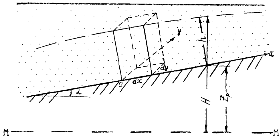
Рис. 2.8. Схема к выводу уравнения плановой фильтрации в безнапорном пласте
