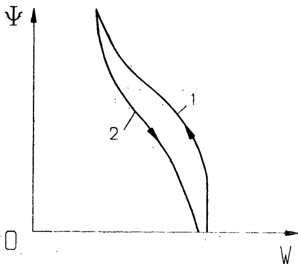
Рис. 6.22. Графики зависимости всасывающего давления от влажности при осушении (1) и водонасыщении (2)
