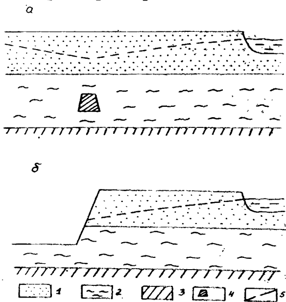
Рис. 2.1. Схема слоистой водоносной толщи, вскрытой штреком (а) и карьером (б):
