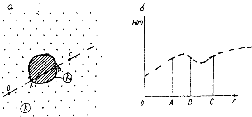
Рис. 5.14. Схема откачки в условиях плановой фильтрационной неоднородности:
