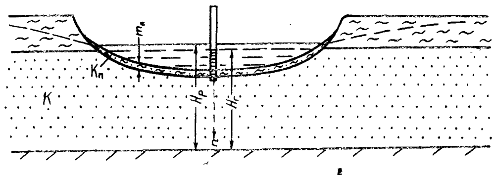
Рис. 2.14. Схема разгрузки подземных вод в водоем с граничным условием III рода
