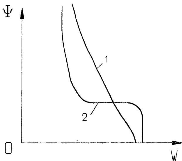
Рис. 6.21. Характерные графики зависимости всасывающего давления от влажности для грунта:
