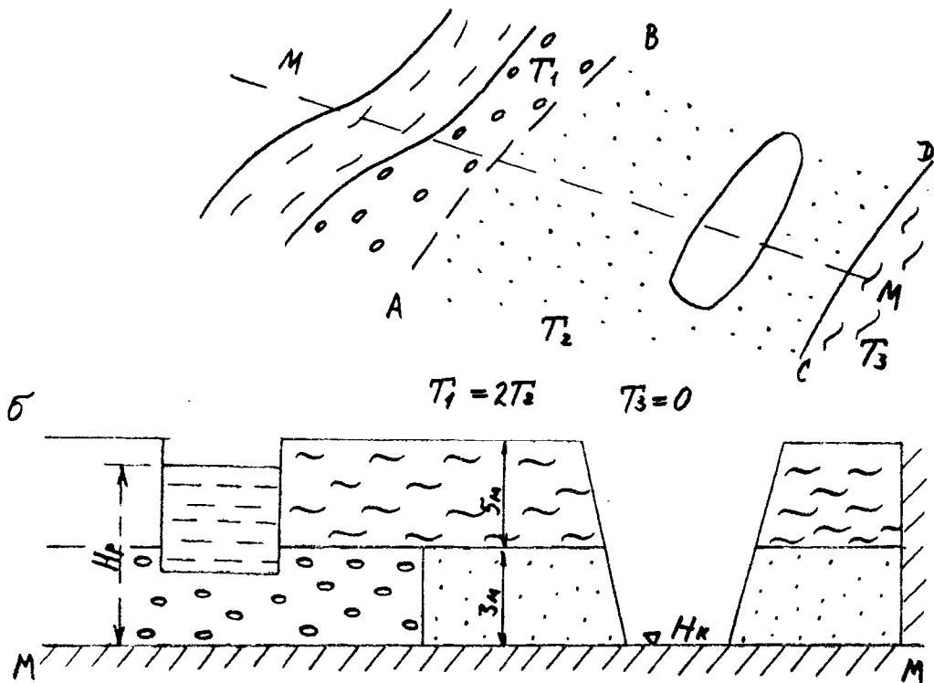
Рис. 3.17. План (а) и разрез (б) планово-неоднородного пласта
