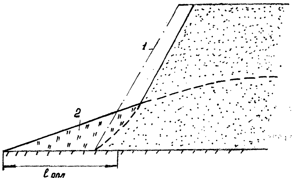
Рис. 8.3. Схема оплывающего откоса:
