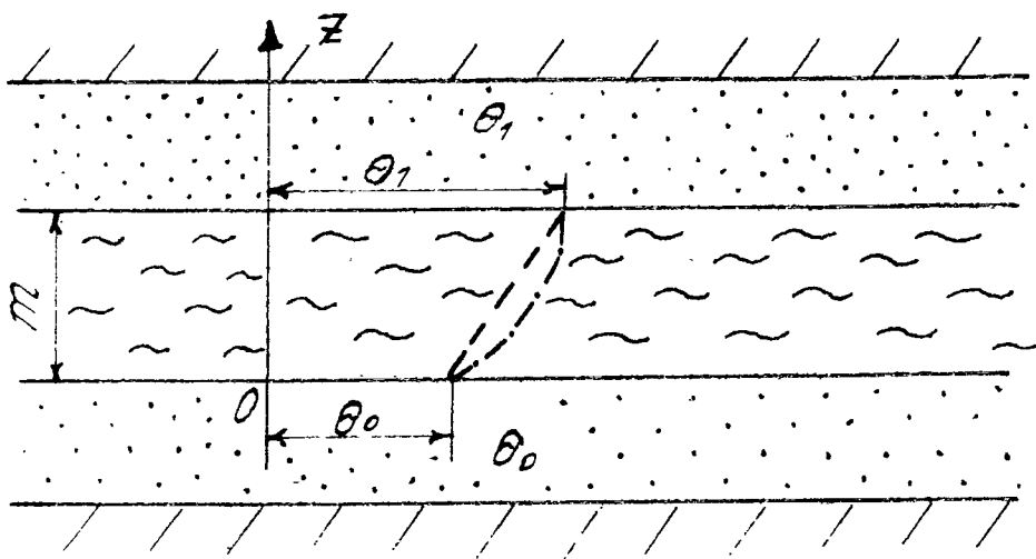
Рис. 6.15. Схема переноса тепла через относительно водоупорный слой
