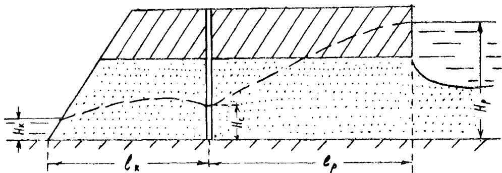
Рис. 3.15. Схема к задаче о контуре скважин между рекой и карьером
