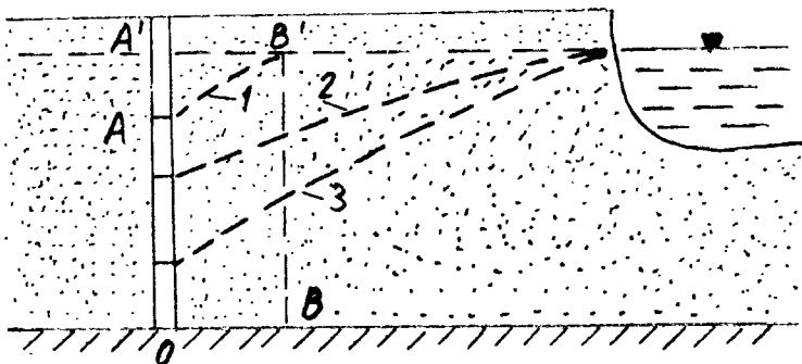
Рис. 4.1. Фильтрация к скважине вблизи реки
