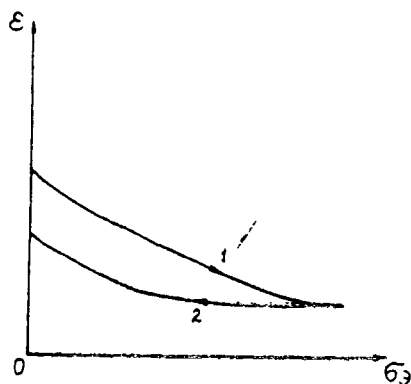
Рис. 1.19. Компрессионная (1) и декомпрессионная (2) кривые
