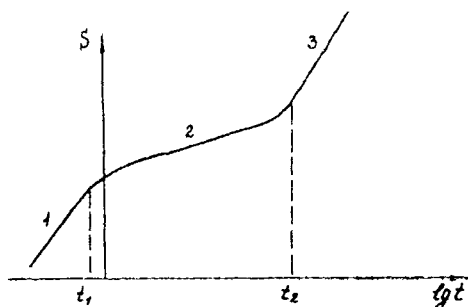
Рис. 5.9. Типовой индикаторный график откачки из пласта пород с двойной емкостью
