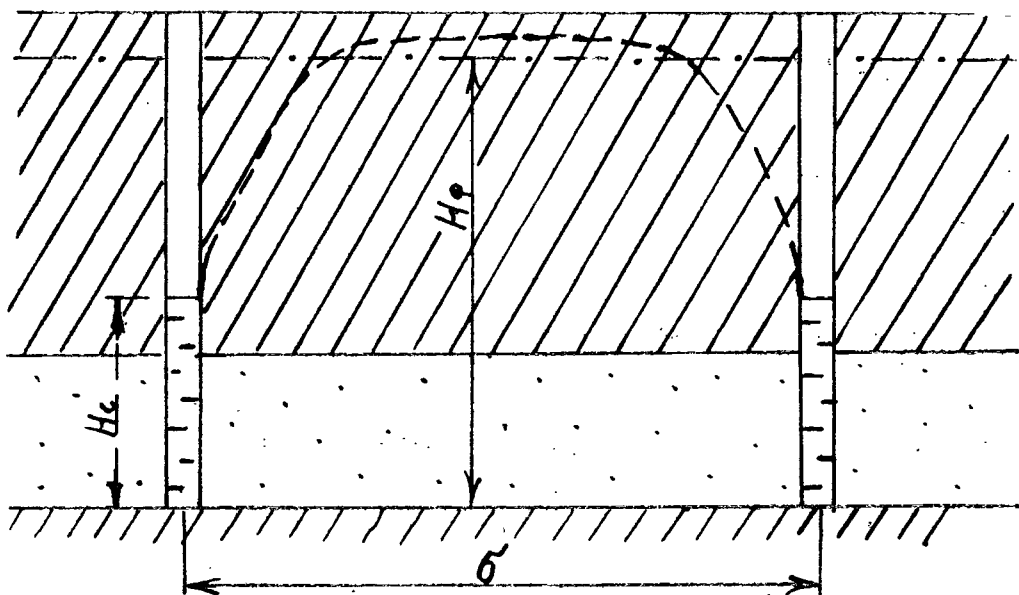
Рис. 3.14. Разрез по линии скважин
