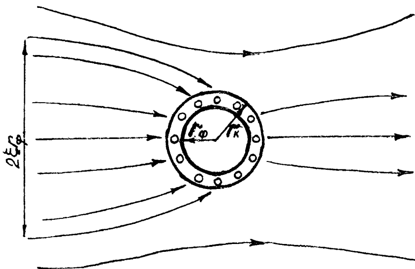
Рис. 6.5. Схема линий тока вблизи наблюдательной скважины
