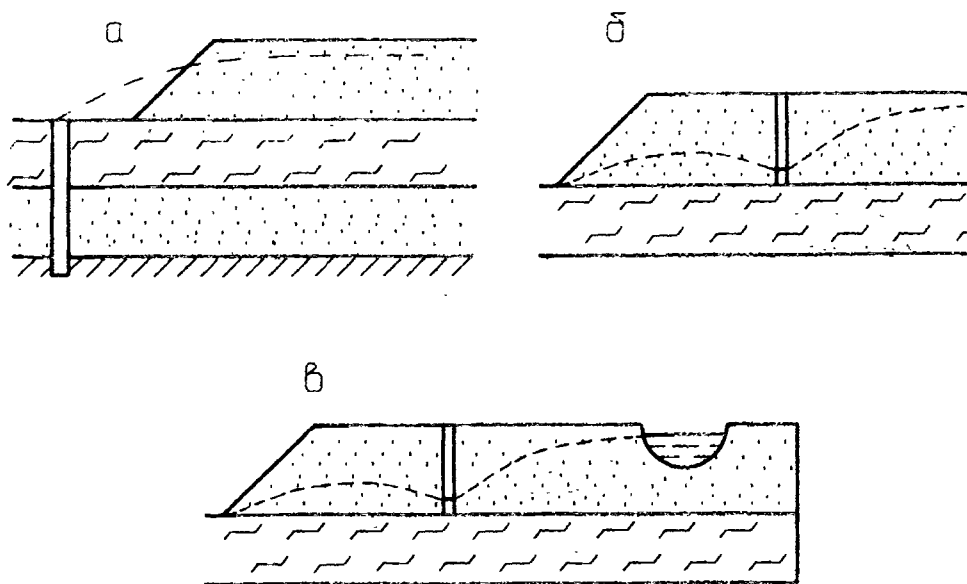
Рис. 8.7. Схемы расположения дренажных скважин для различных типов пласта:
