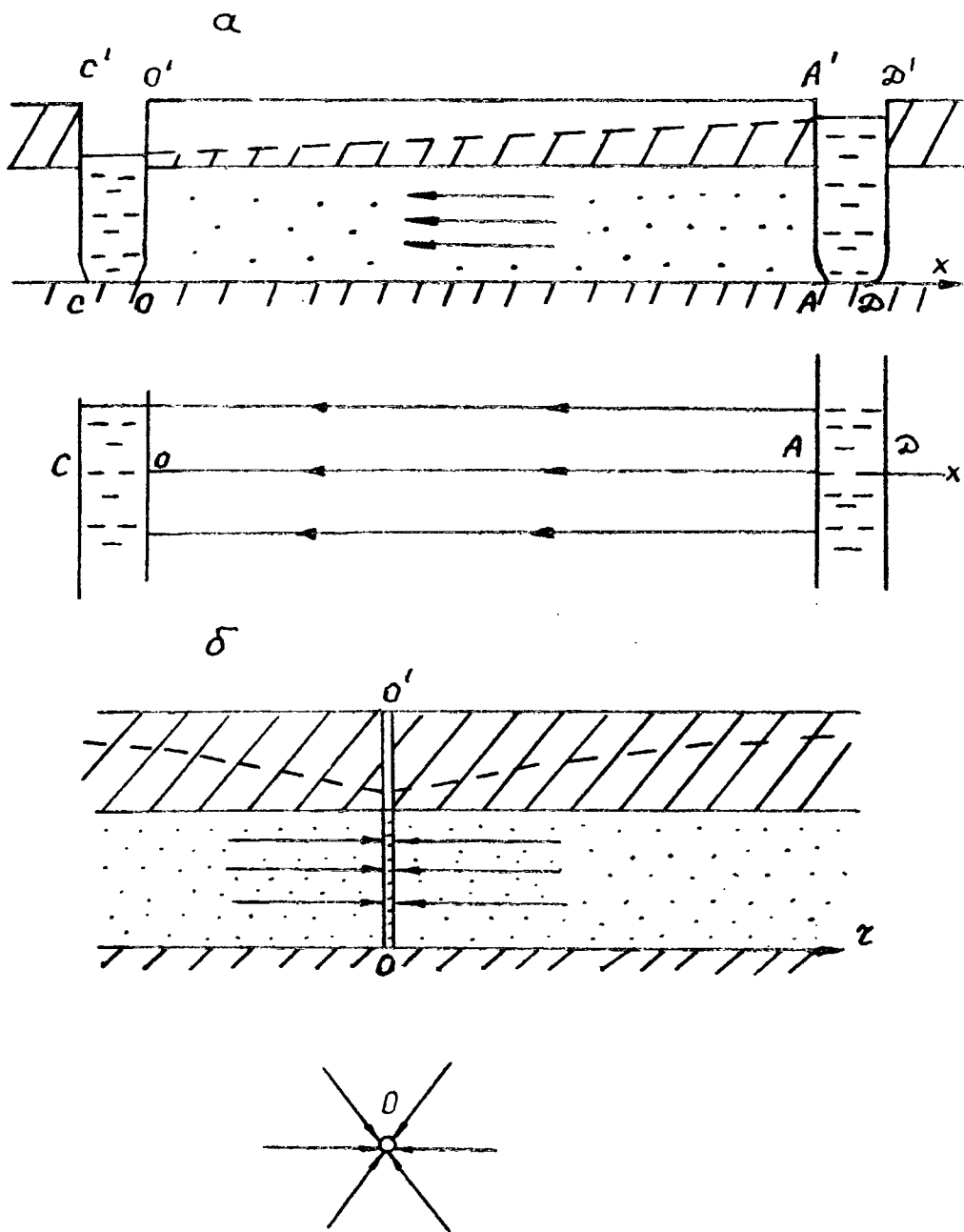
Рис. 2.3. Схемы одномерной фильтрации: а - плоскопараллельной; б - плоскорадиальной
