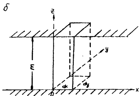
Рис. 2.6. Схемы к выводу уравнений неразрывности для напорного пласта:
