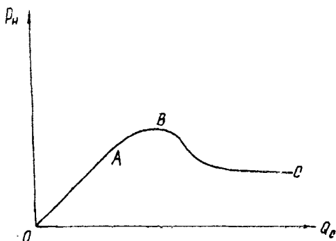
Рис. 5.12. Типовой график зависимости расхода скважины от давления нагнетания
