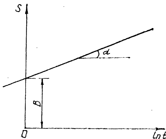
Рис. 5.1. Интерпретация данных откачки по способу прямой
