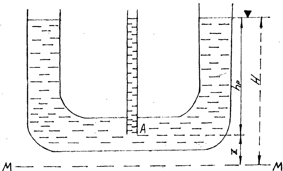
Рис. 1.3. Схема, иллюстрирующая понятие гидростатического напора
