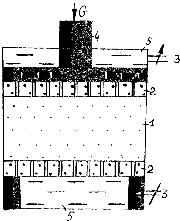
Рис. 1.24. Схема опыта с образцами песка в компрессионном приборе: 1 - образец; 2 - проницаемые прокладки; 3 - краны; 4 - дырчатый поршень, передающий внешнюю нагрузку на образец; 5 - камеры с водой под напором
