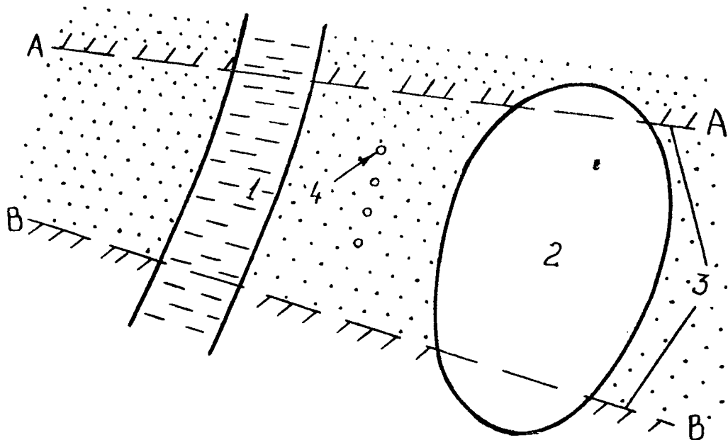
Рис. 2.12. Схема области фильтрации
