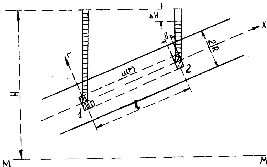
Рис. 1.6. Схема к выводу формулы Гагена-Пуазейля
