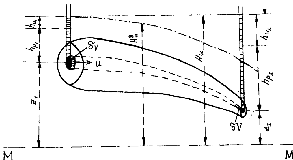
Рис. 1.4. Трубка тока в идеальной жидкости
