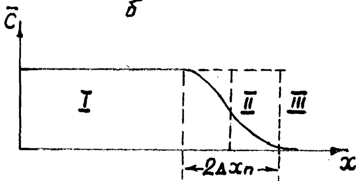
Рис. 6.10. Схема миграции в водоносном пласте (а) и характерный график пространственного изменения концентрации (б)
