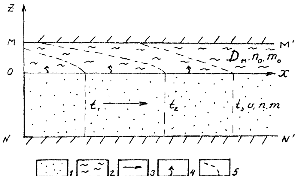
Рис. 6.12. Схема миграции подземных вод в двуслойном пласте: 1 - хорошопроницаемый слой; 2 - слабопроницаемый слой; направления потоков: 3 - конвективного; 4 - диффузионного; ММ' и NN' - границы расчетного элемента, непроницаемые для воды и вещества; 5 - положение концентрационного фронта на различные моменты времени t
