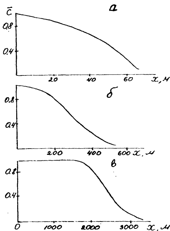
Рис. 6.13. Характерные графики изменения концентрации по направлению переноса в гетерогенных комплексах (положения а, б и в отвечают увеличению времени переноса)
