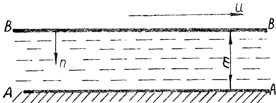
Рис. 1.1. Схема к оценке сил вязкого трения в жидкости
