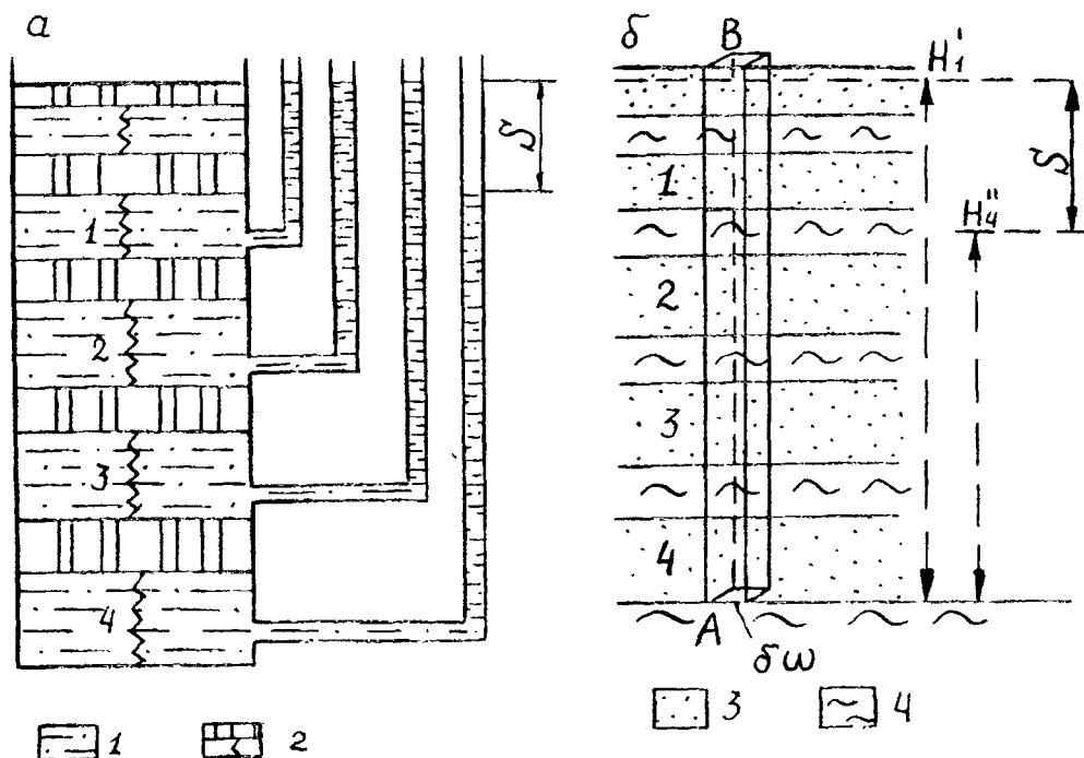
Рис. 1.15. Схема, иллюстрирующая взаимодействие эффективных и нейтральных напряжений:
