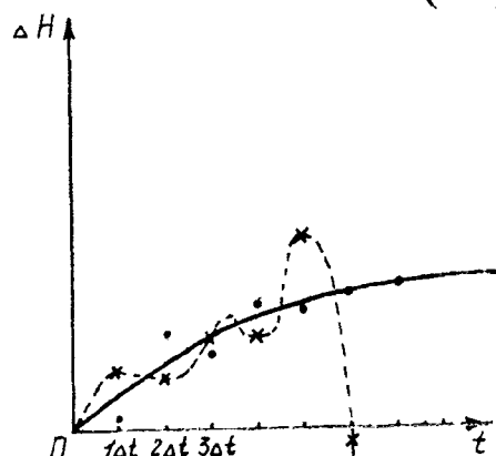
Рис. 4.9. Схематизированное представление результатов расчета фундаментальной фильтрационной задачи: 1 — данные расчета по неявной схеме; 2 — то же, по явной схеме; 3 — точное аналитическое решение
