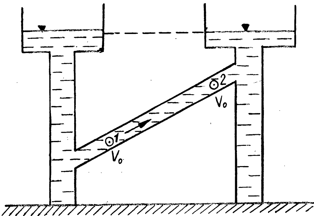
Рис. 1.5. Схема к оценке изменения энергии фиксированного объема в движущейся жидкости
