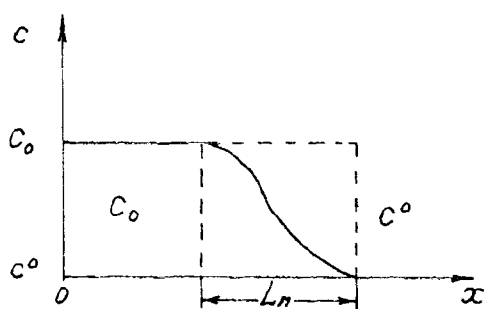
Рис. 6.6. Характерный график пространственного изменения концентрации при наличии диффузии или гидродисперсии
