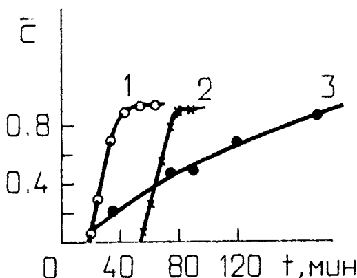
Рис. 6.18. Характерные выходные кривые для индикатора:
