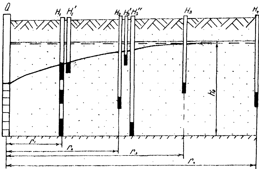
Рис. 7.3. Схема опытного куста при откачке в однородном безнапорном пласте:
