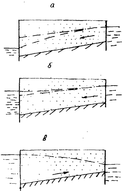
Рис. 3.7. Схемы безнапорной фильтрации при наклонном водоупоре
