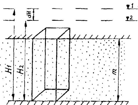
Рис. 1.18. Схема к оценке упругой емкости пласта
