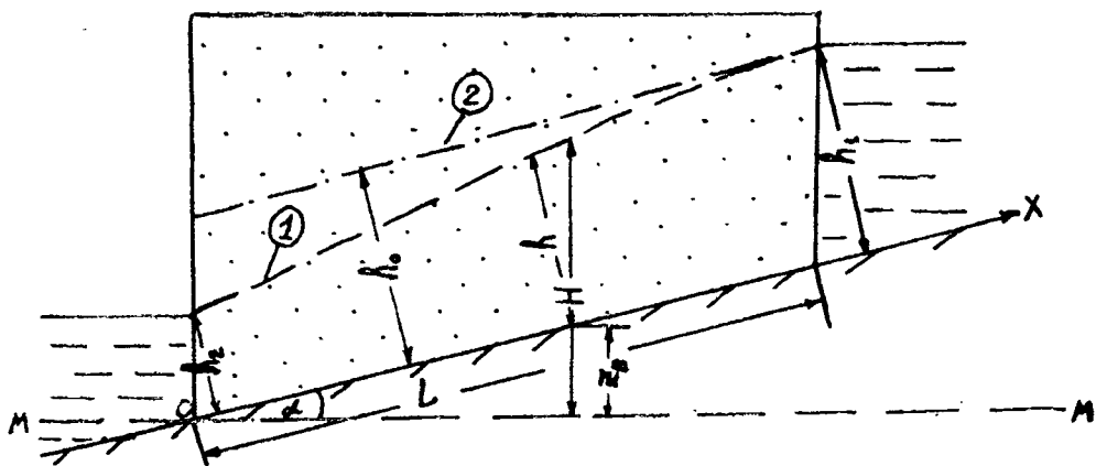
Рис. 3.6. Схема безнапорной фильтрации при наклонном водоупоре: 1 - депрессионная кривая; 2 - поверхность уровня расчетного равномерного потока
