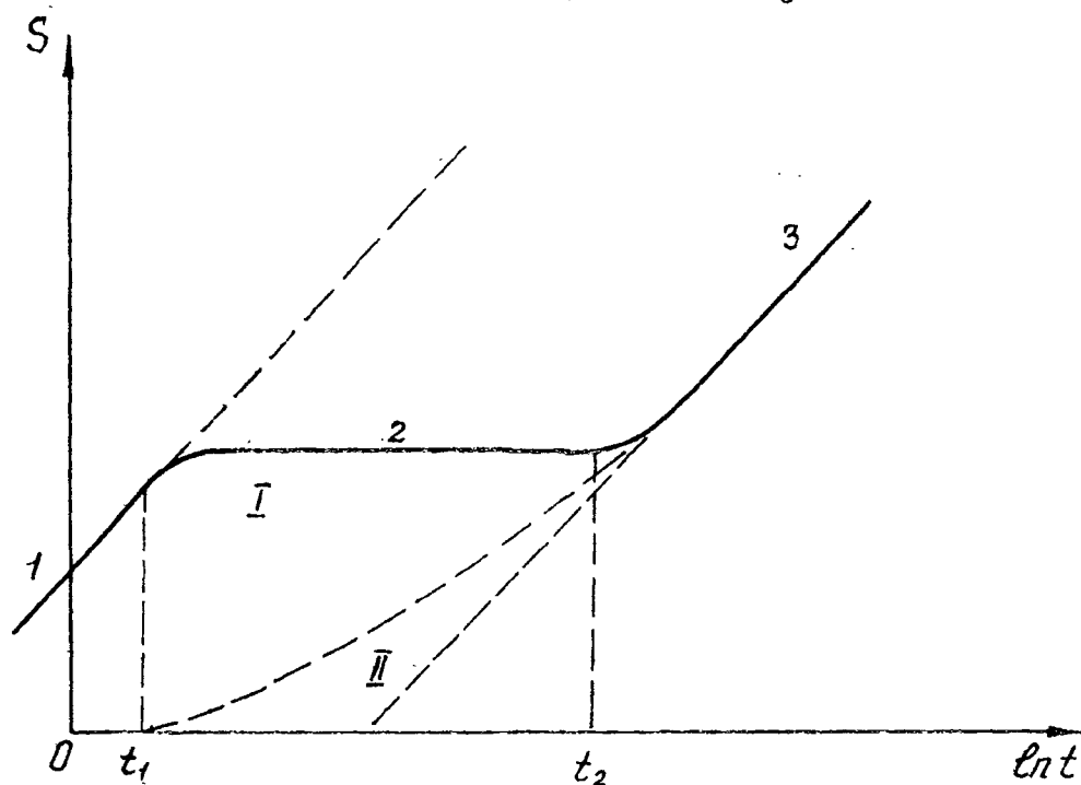
Рис. 5.10. Типовой индикаторный график откачки из двухслойного безнапорного пласта:
