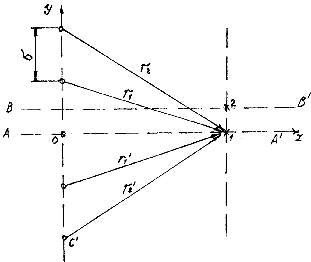
Рис. 3.13. Схема к расчету контура скважин в неограниченном пласте
