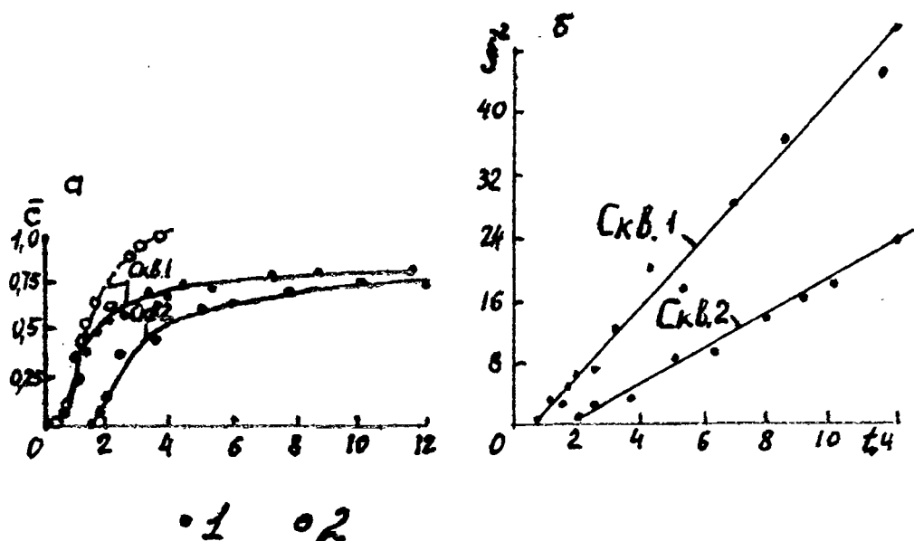
Рис. 7.4. Графики изменения относительных концентраций индикаторов в наблюдательных скважинах (а) и представление опытных данных при графоаналитическом способе их интерпретации (б):
