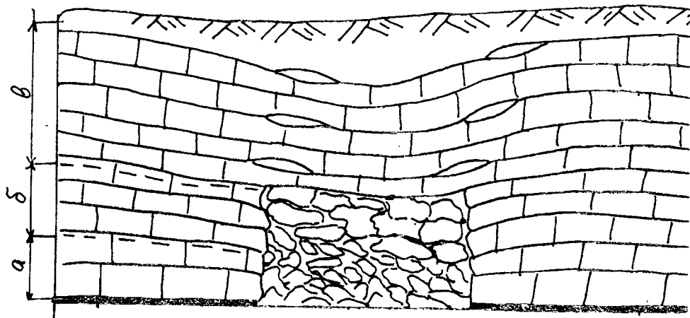
Рис. 8.5. Схематический разрез подработанной толщи горных пород
