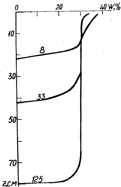
Рис. 6.25. Характерные опытные графики зависимости влажности от глубины просачивания (цифры на кривых - время от начала опыта, мин.)
