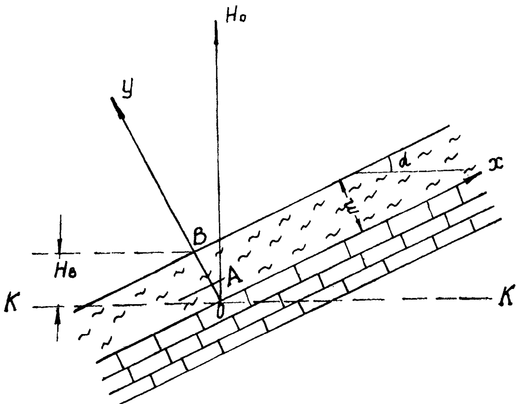
Рис. 8.1. Схема расчета эффективных напряжений вблизи откоса
