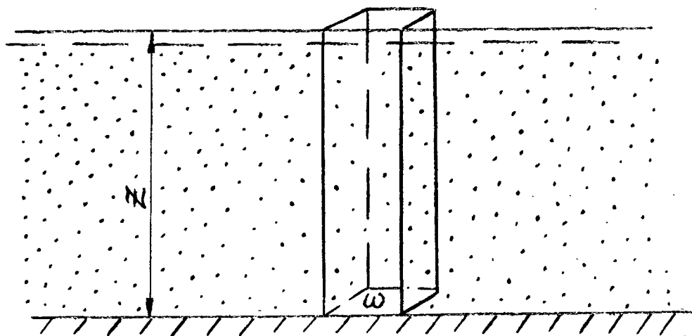
Рис. 1.14. Схема, иллюстрирующая действие сил гидростатического взвешивания в безнапорном пласте
