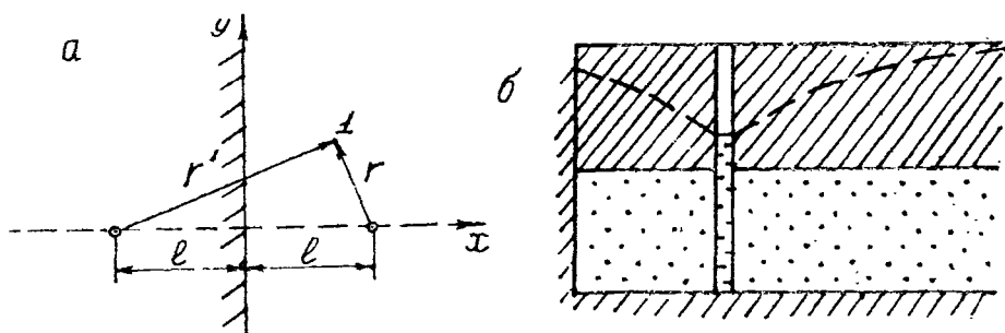
Рис. 4.5. Фильтрация к скважине вблизи непроницаемой границы: а - план; б - разрез
