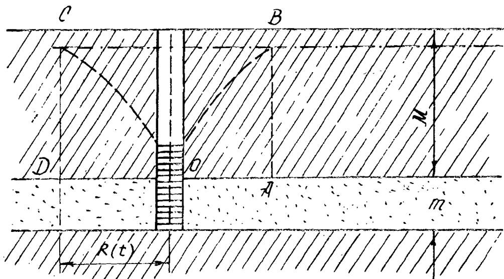
Рис. 5.11. Схема, иллюстрирующая эффект жесткости кровли напорного водоносного пласта при откачке
