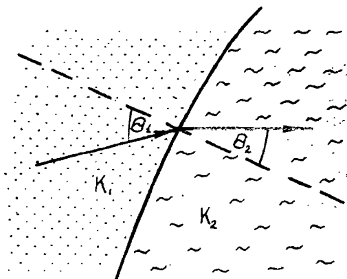
Рис. 2.11. Преломление линий тока на границе двух зон с различной проницаемостью
