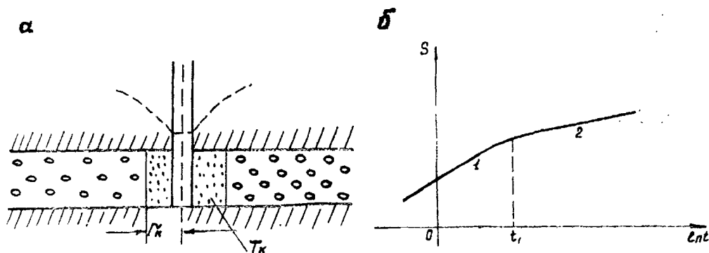
Рис. 5.16. Схемы откачки из скважины при наличии скин-эффекта: а - разрез прискважинной зоны; б - типовой индикаторный график
