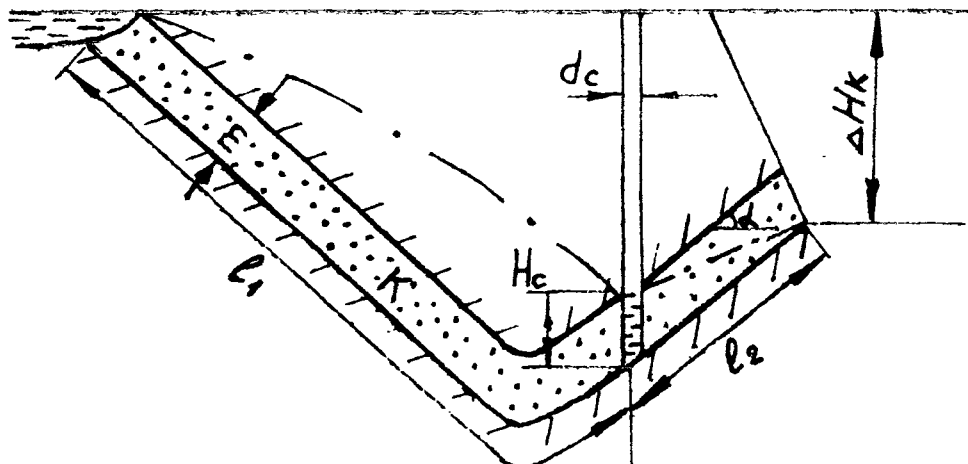
Рис. 8.8. Схема фильтрации к карьеру в условиях наклонного залегания водоносного пласта
