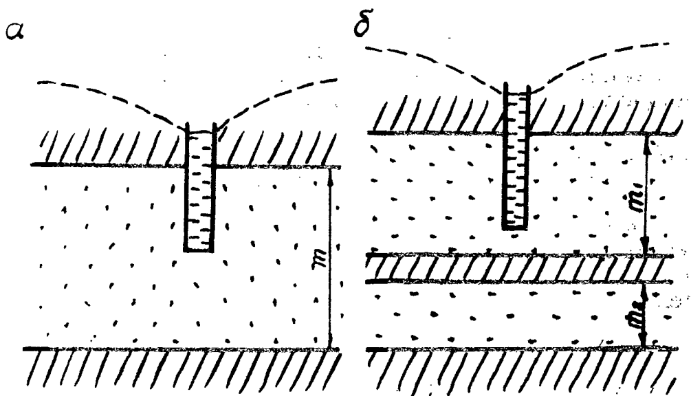
Рис. 5.15. Схемы откачки из несовершенной скважины: а - однородный пласт; б - пласт с водоупорным прослоем
