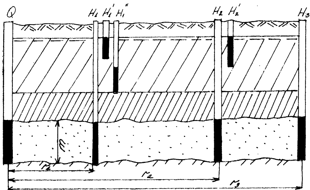
Рис. 7.2. Схема опытного куста при откачке в двухслойном пласте; Q - центральная скважина; H_1 - H_3 - пьезометры на основной слой; H_1' , H_2' , H_1'' - пьезометры-«дублиеры» на слабопроницаемый слой
