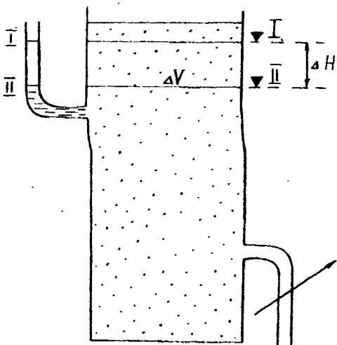
Рис. 1.17. Схема опыта по определению гравитационной водоотдачи
