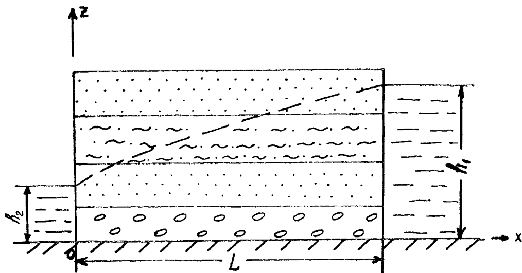
Рис. 3.3. Схема фильтрации в безнапорном слоистом пласте
