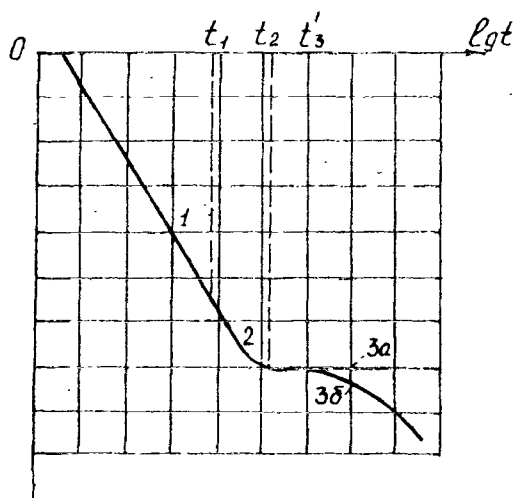
Рис. 5.6. Типовые индикаторные графики откачки при наличии перетекания
