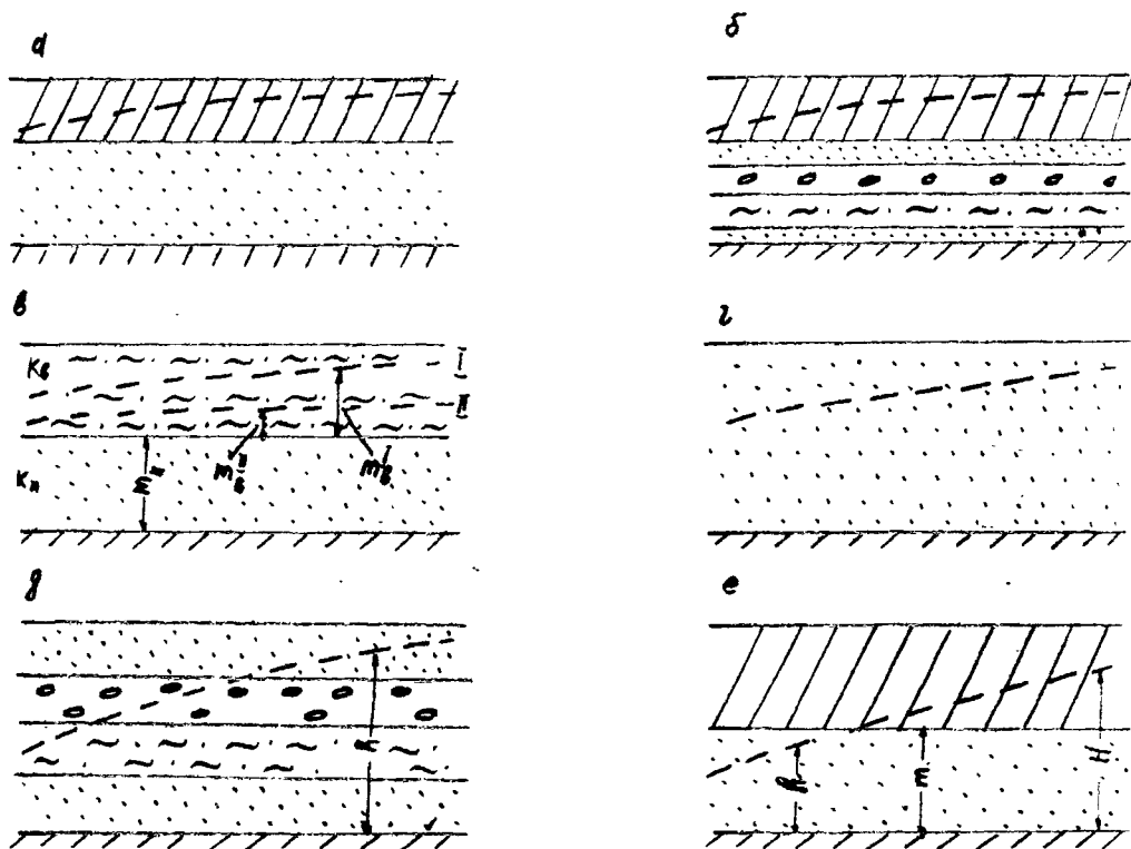
Рис. 2.16. Основные расчетные схемы плановой фильтрации
