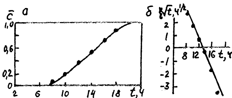
Рис. 6.17. Выходная кривая миграционного опыта (а) и ее представление в «спрямляющих» координатах (б)
