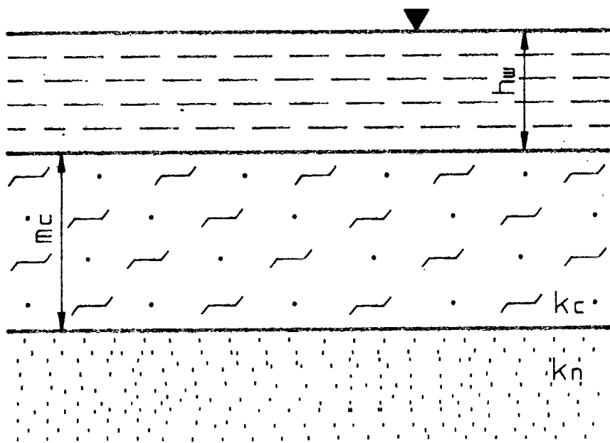
Рис. 6.27. Схема оценки условий образования насыщенного потока при наливе в двухслойную толщу
