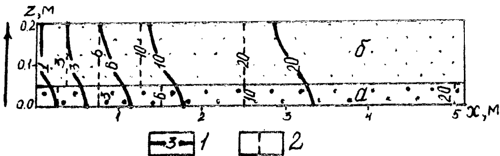
Рис. 6.14. Характер массопереноса в двухслойном пласте ( по результатам математического моделирования):
