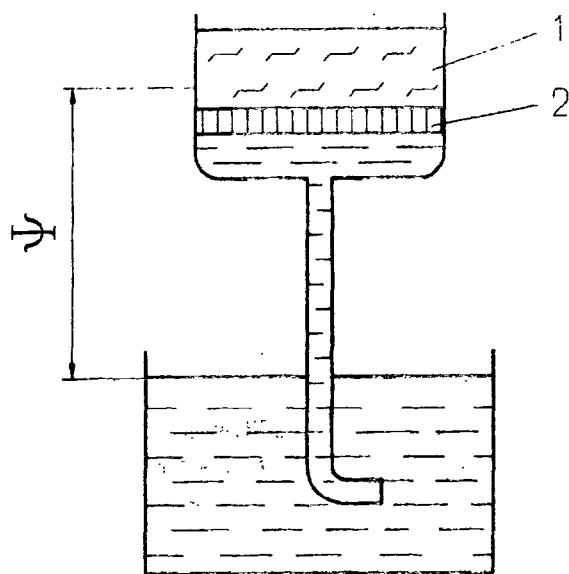
Рис. 6.20. Схематическое представление измерения всасывающего давления: 1 - образец; 2 - тонкопористая мембрана
