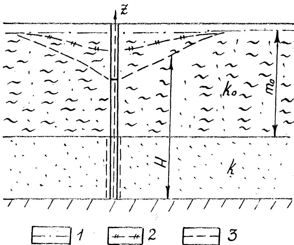
Рис. 5.5. Схема безнапорного двухслойного пласта: 1 - исходное положение уровней; 2 - положение свободной поверхности при откачке; 3 - напорная линия нижнего слоя при откачке
