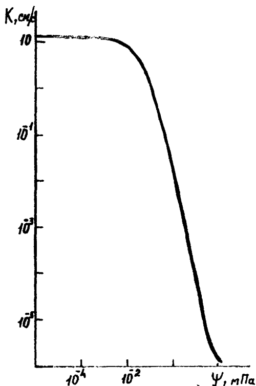
Рис. 6.24. Характерная опытная кривая зависимости коэффициента влагопереноса от всасывающего давления [6]
