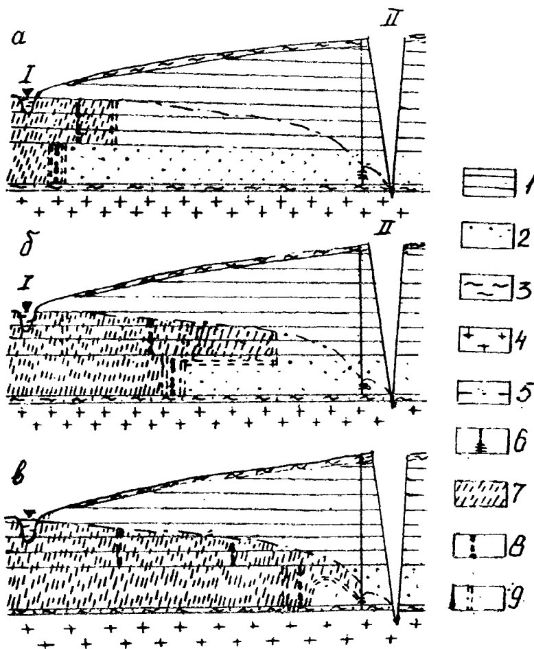
Рис. 8.11. Схемы прогнозной оценки загрязнения подземных вод на участке хвостохранилище (I) - карьер (II) на начальные (а), промежуточные (б) и конечные (в) моменты времени:
