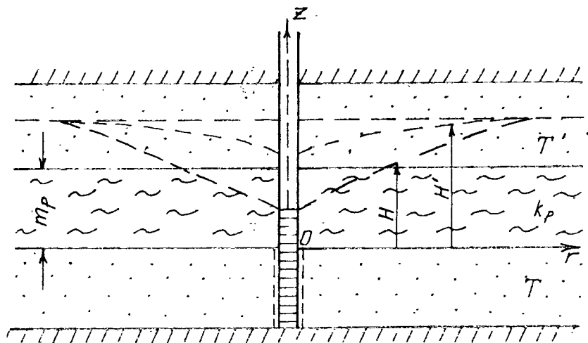
Рис. 5.2. Схема взаимодействующих пластов
