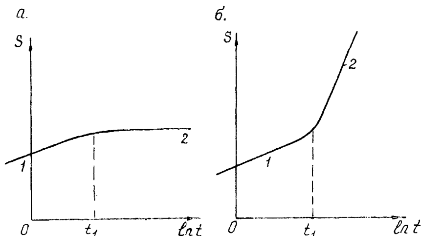
Рис. 5.13. Индикаторные графики откачек, проводимых вблизи границ водоносных пластов:
