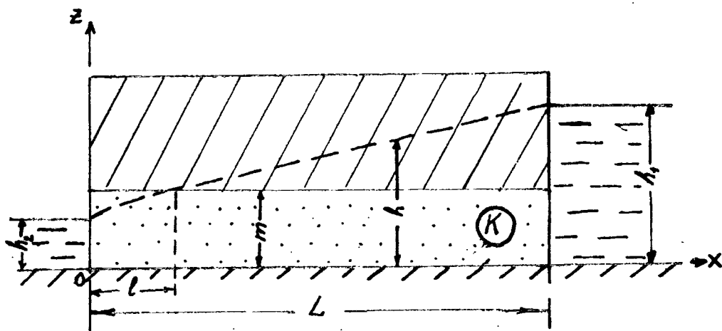
Рис. 3.4. Схема напорно-безнапорной фильтрации между двумя бассейнами
