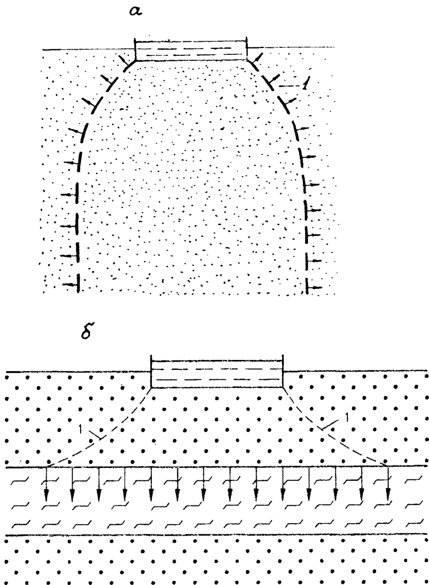
Рис. 6.26. Боковое растекание воды при наливах в шурфы: а - однородные породы; б - слоистый комплекс; 1 - положение фронта увлажнения
