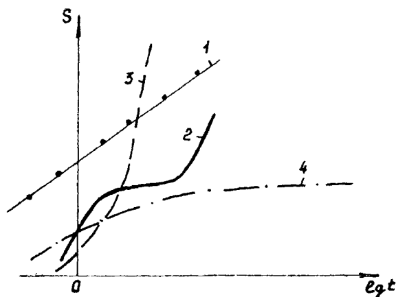
Рис. 5.18. Характерные индикаторные графики откачки:
