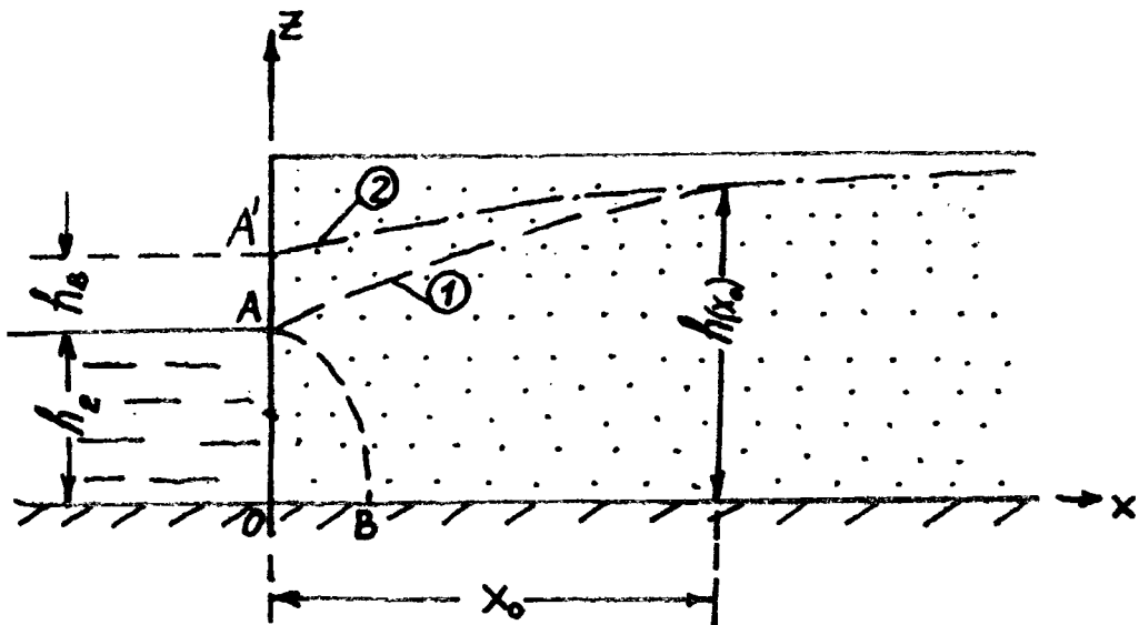
Рис. 3.2. Схема фильтрационного потока вблизи промежутка высачивания:
