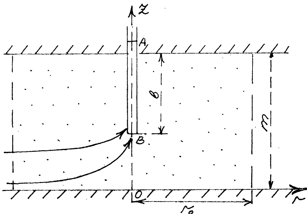
Рис. 3.16. Схема искривления линий тока вблизи несовершенной скважины
