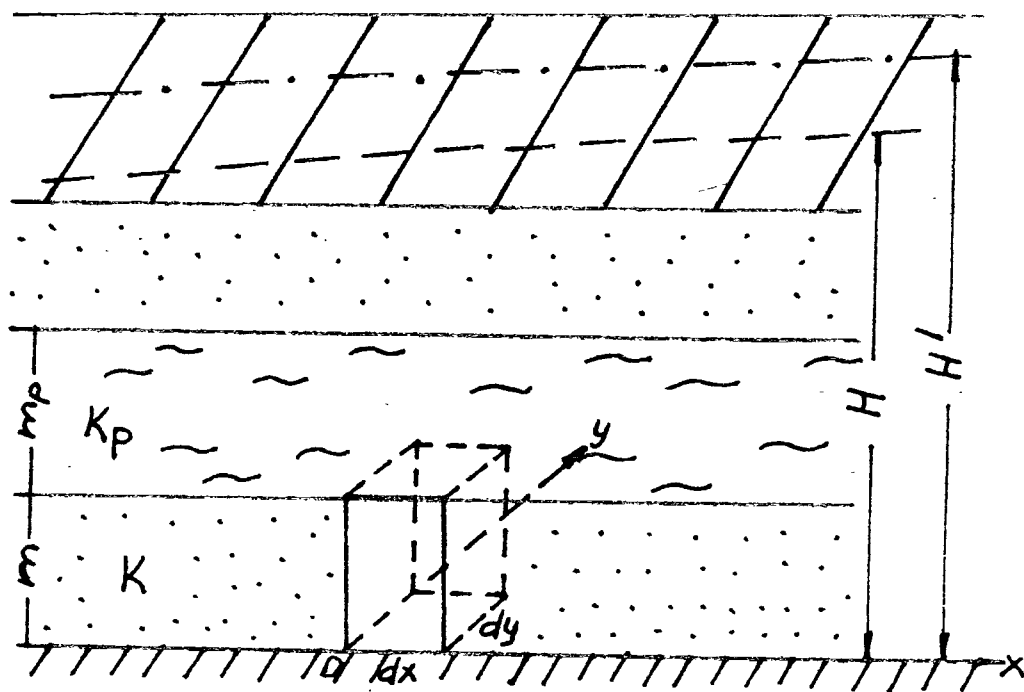
Рис. 2.7. Схема к выводу уравнения неразрывности в пласте с перетеканием
