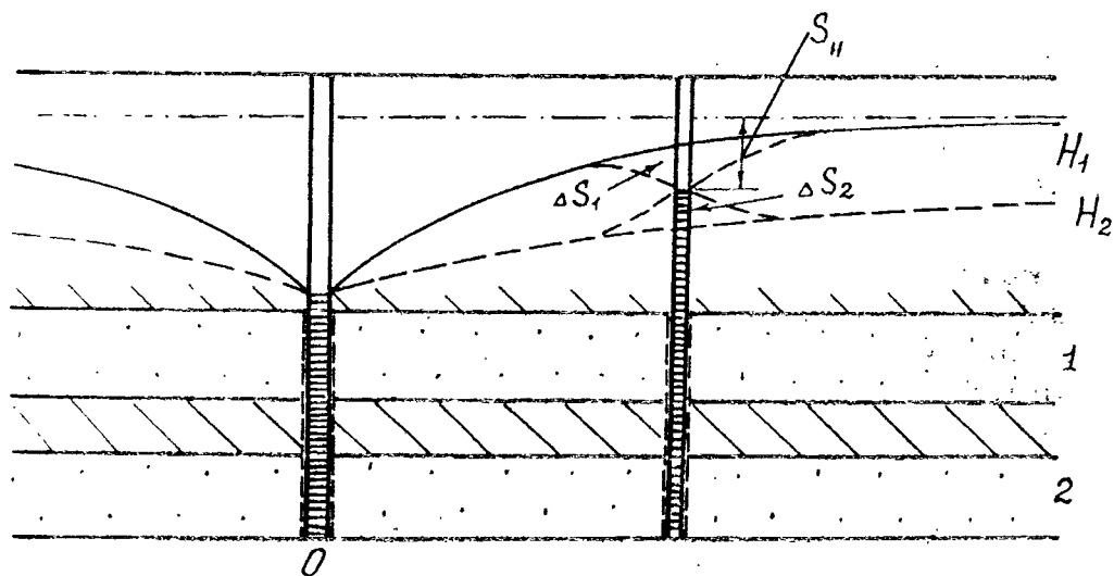
Рис. 5.7. Схема двухпластовой системы
