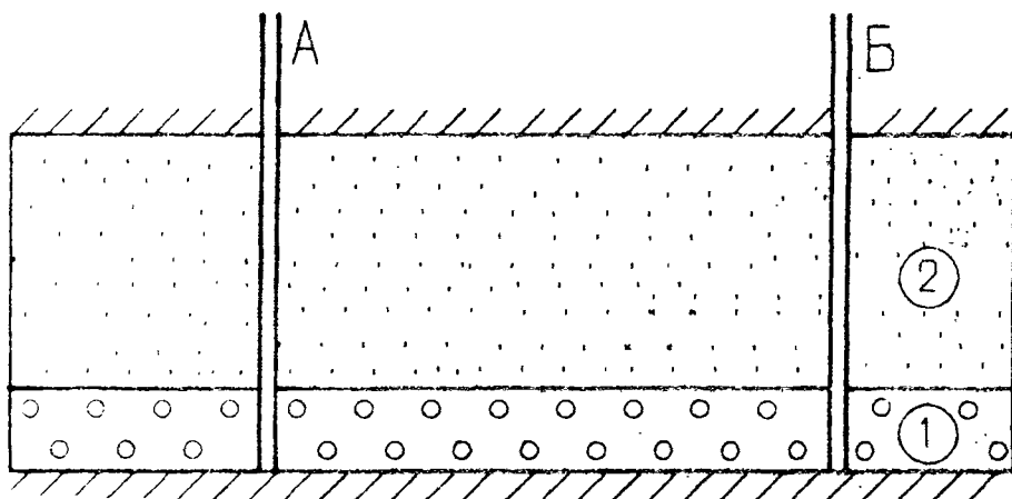
Рис. 6.19. Схема опробования двухслойного водоносного пласта
