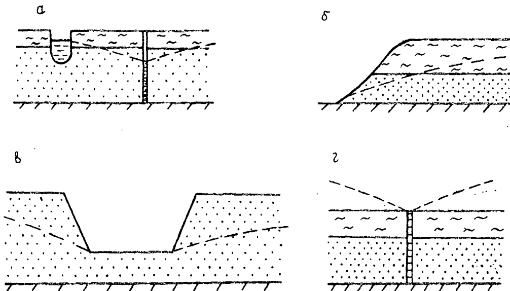
Рис. 2.13. Варианты границ пласта с условиями I рода
