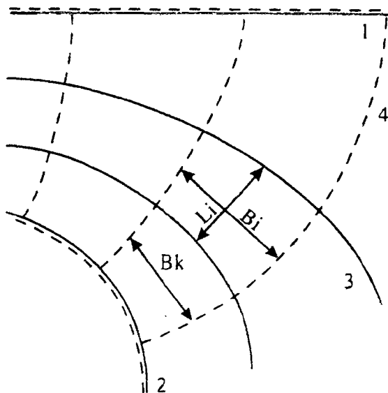
Рис. 8.9. Схема определения расчетной длины ленты тока:
