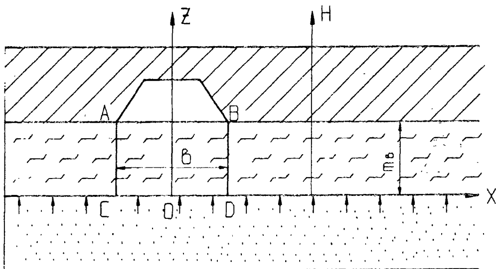
Рис. 8.4. Схема оценки возможности прорыва подземных вод в штрек
