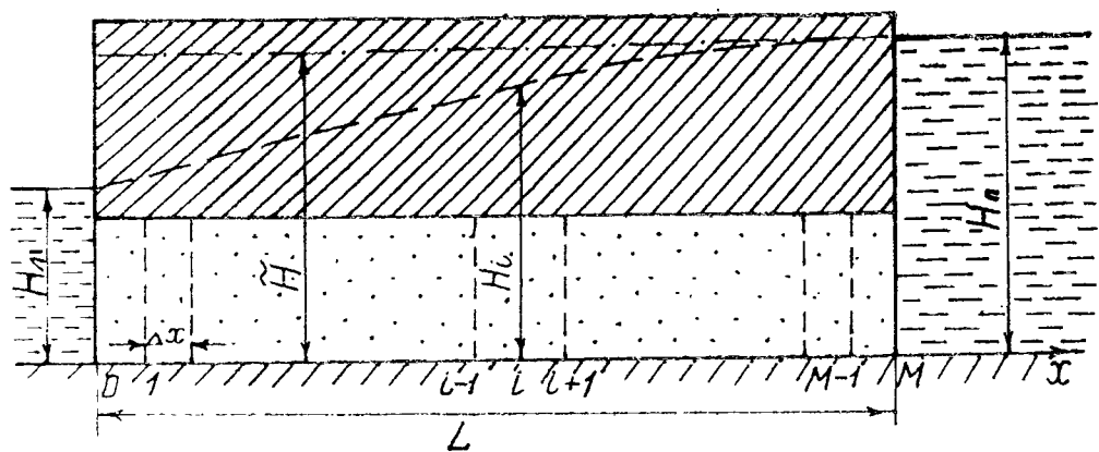
Рис. 4.8. Схема пространственной разбивки области фильтрации
