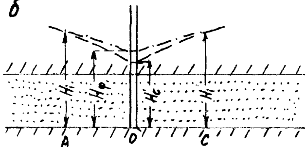
Рис. 3.20. Схемы к обоснованию методики представления скважин на сеточной модели в плане (а) и разрезе (б)
