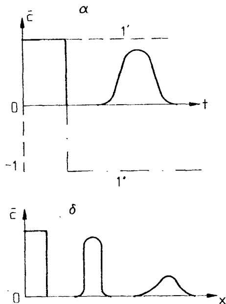
Рис. 6.11. Характерные графики изменения относительной концентрации при пакетном запуске индикатора:
