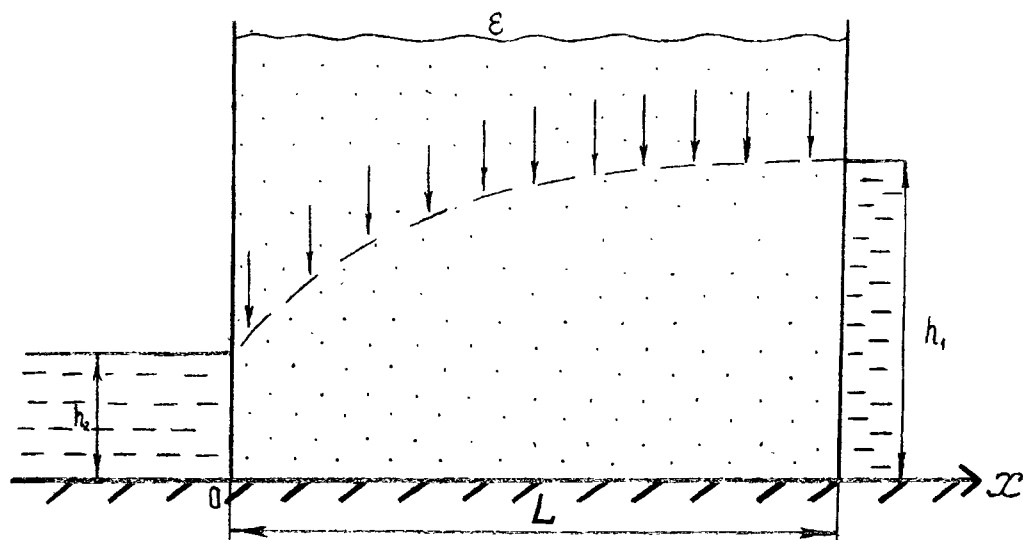
Рис. 3.1. Схемы напорной (а) и безнапорной (б) фильтрации между двумя бассейнами
