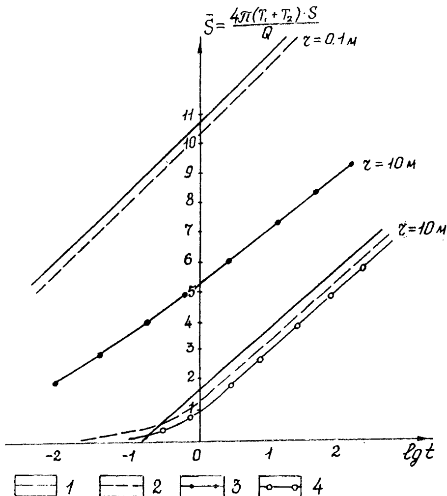
Рис. 5.8. Расчетные графики приведенных понижений для двухслойной системы:
