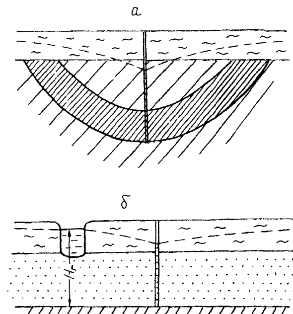
Рис. 2.9. Схемы закрытого водоносного пласта (а) и безнапорного пласта с границей обеспеченного питания (б)
