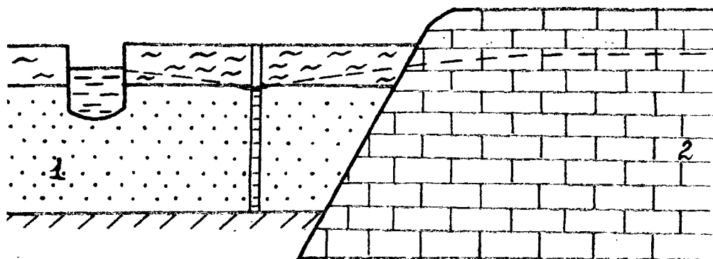
Рис. 2.10. Схемы совершенной скважины в неограниченном пласте (а) и области фильтрации, содержащей границу раздела — контакт водоносных пород с различными фильтрационными свойствами (б)
