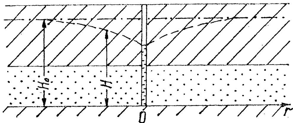
Рис. 4.4. Схема фильтрации к скважине в неограниченном пласте
