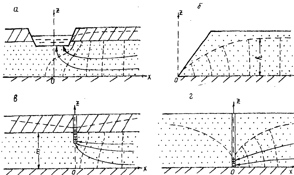
Рис. 2.15. Схематическое представление линий тока и линий равных напоров на участках, прилежащих к границам водоносных пластов:
