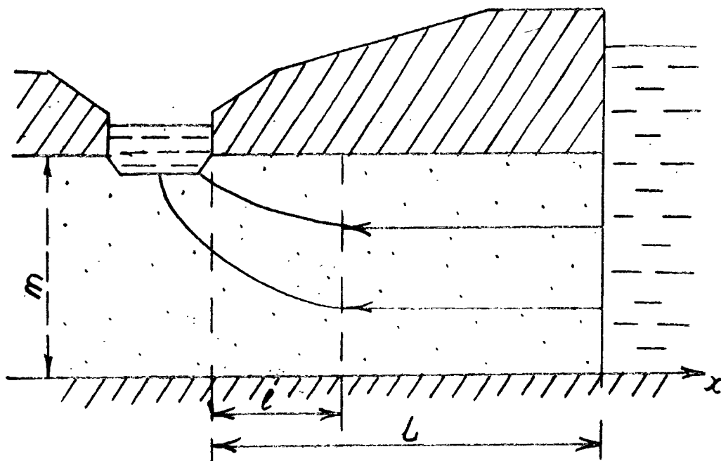
Рис. 3.12. Схема искривления линий тока вблизи реки с несовершенным руслом
