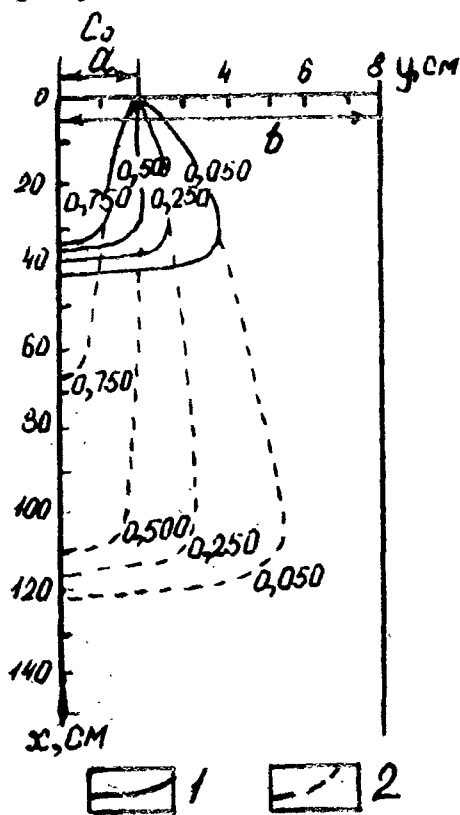
Рис. 6.8. Схема оценки совместного влияния продольной и поперечной дисперсии на распространение индикатора от источника фиксированной длины: 1 - концентрационное поле, рассчитанное для момента времени t = 1,39 ч после начала инъекции индикатора; 2 - то же, для t = 4,16 ч. Числа на графике - значения относительной концентрации c / c_0 при c_0 = 1 ; а - длина участка инъекции; б - расстояние между непроницаемыми границами (ширина области одномерной фильтрации)
