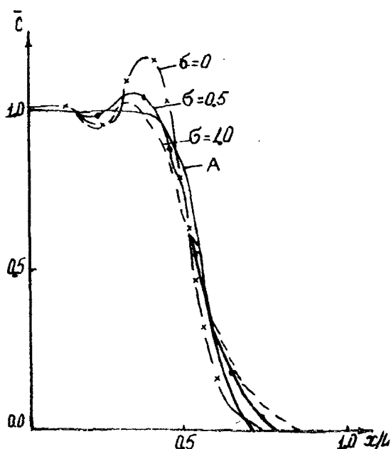
Рис. 8.13. Влияние эффекта осцилляций на точность численного решения для различных схем.
