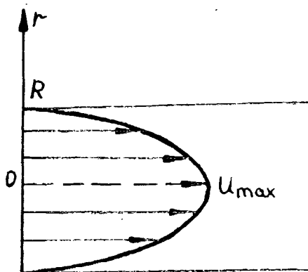
Рис. 1.7. Распределение скорости по поперечному сечению трубы
