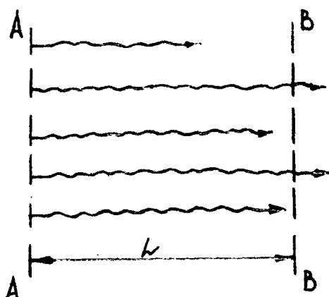
Рис. 6.7. Схема движения частиц жидкости в пористой среде
