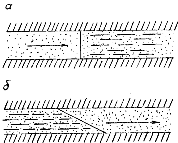
Рис. 6.1. Схемы миграции двух жидкостей различного состава
