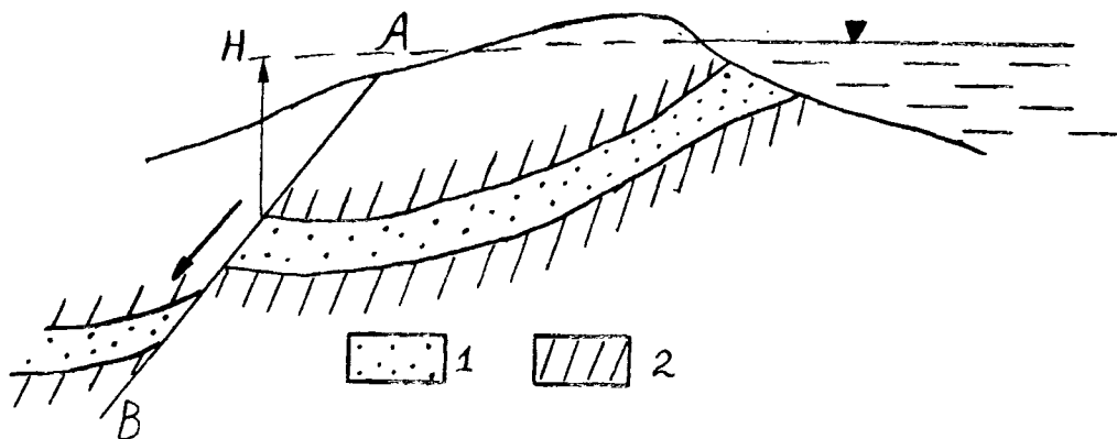
Рис. 1.16. Механизм влияния напорных вод на сейсмическую устойчивость массива горных пород:
