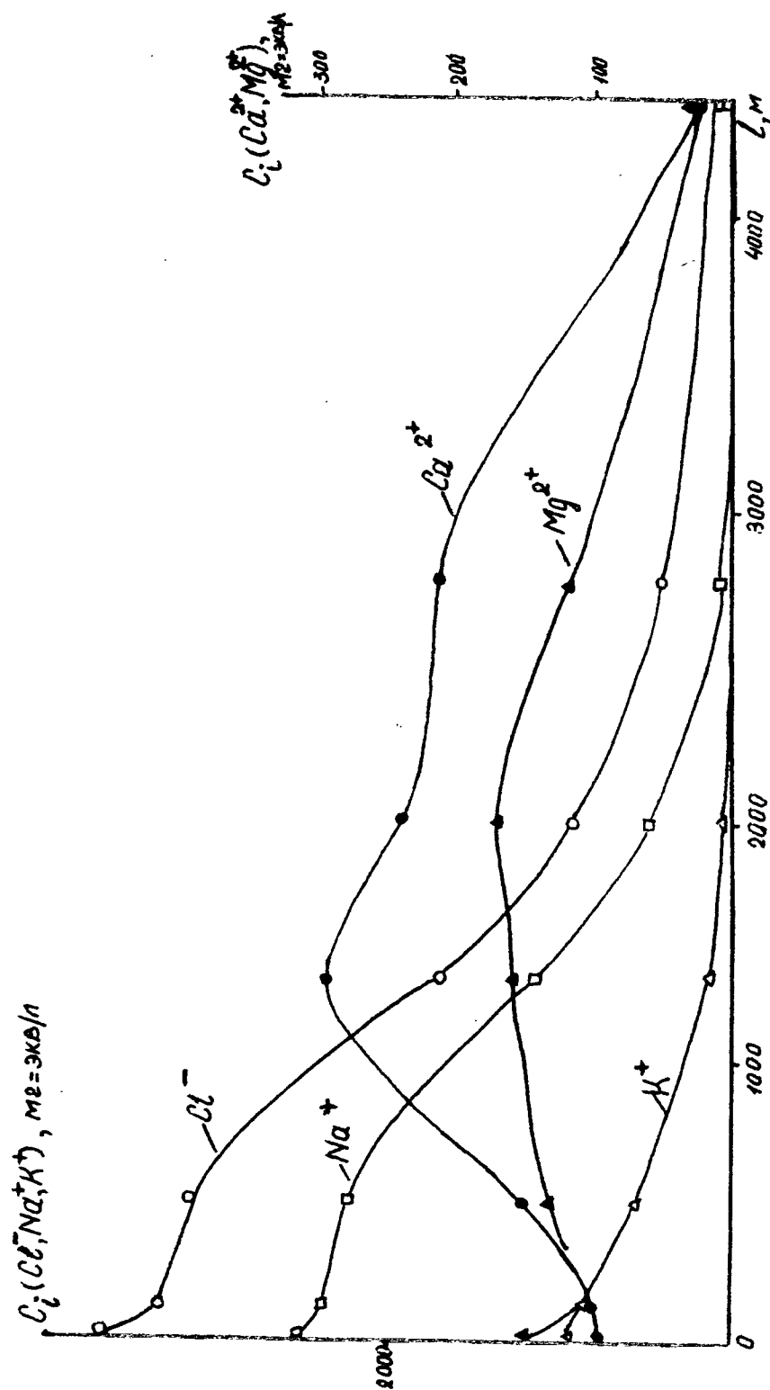
Рис. 6.4. Закономерности изменения содержания ионов при миграции хлоридно-натриевых рассолов в комплексе карбонатно-глинистых пород (1 - расстояние от рассолонакопителя)
