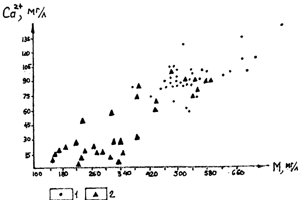
Рис. 7.5. Результаты химических анализов проб воды, отобранных из эксплуатационных (1) и наблюдательных скважин без прокачки (2)
