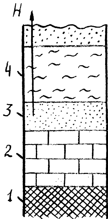
Рис. 1.20. Схематическая колонка нижней пачки осадочных пород Южно-Белозерского месторождения:
