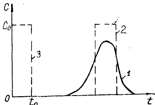
Рис. 1.23. График изменения концентрации индикатора C :
