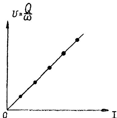
Рис. 1.21. График зависимости скорости фильтрации от градиента
