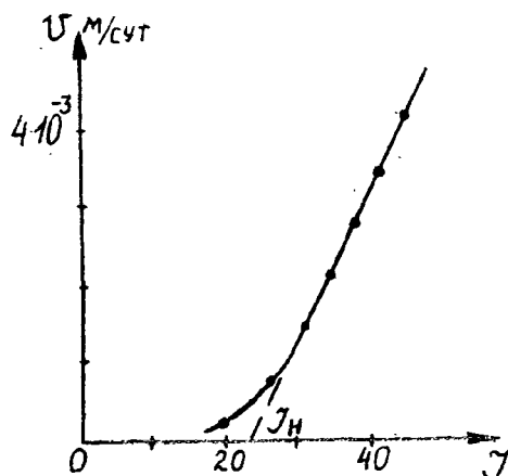
Рис. 1.22. График зависимости скорости фильтрации от градиента
