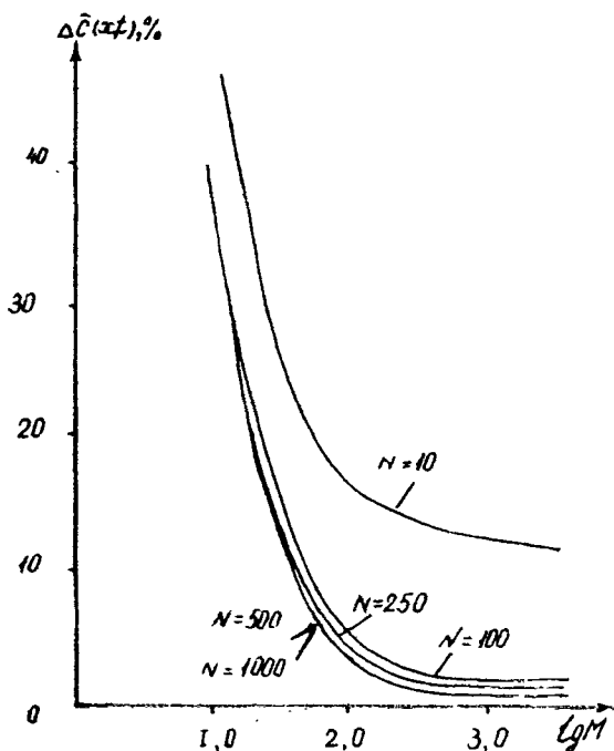
Рис. 8.12. График зависимости относительной погрешности сеточного решения \Delta \tilde{c}(x,t) задачи конвективно-диффузионного переноса от дробности пространственной разбивки
