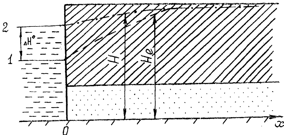
Рис. 4.2. Развитие подпора вблизи водохранилища:
