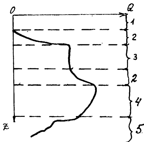
Рис. 8.6. Характерный график расходометрического каротажа, скважины в подработанном массиве.
