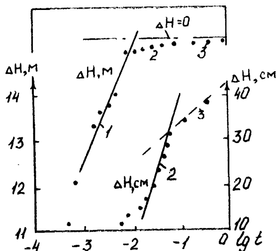
Рис. 5.19. График восстановления уровня \Delta H после откачки
