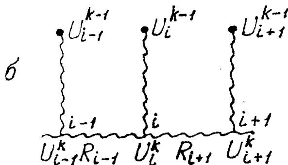
Рис. 4.7. Моделирование нестационарной фильтрации:
