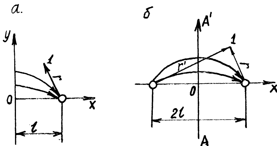
Рис. 3.10. Схемы к задаче о скважине вблизи реки: а - исходная схема; б - вспомогательная схема; 1 - расчетная точка
