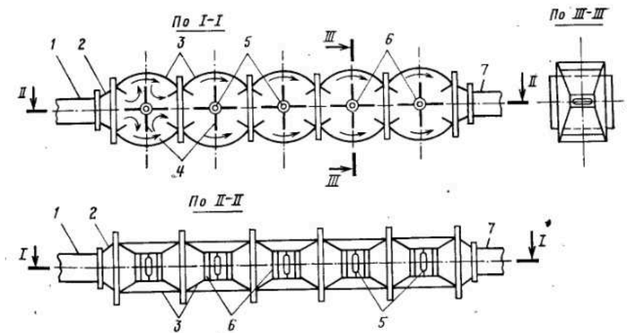
Рис.3.14 Бактерицидная установка ОВ-АКХ-1:
