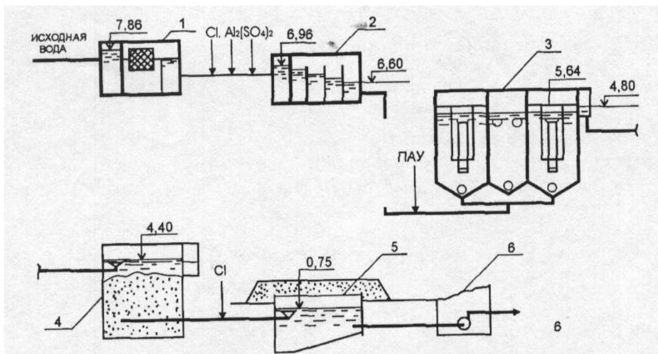
Рис. 3.29 Технологическая высотная схема очистной станции с осветлением в слое взвешенного осадка на скором фильтре:
