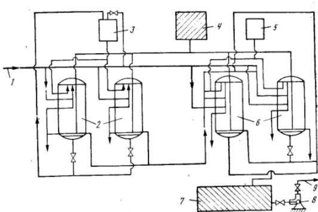
Рис.3.21 Схема двухступенчатого натрий-катионитового умягчения воды:
