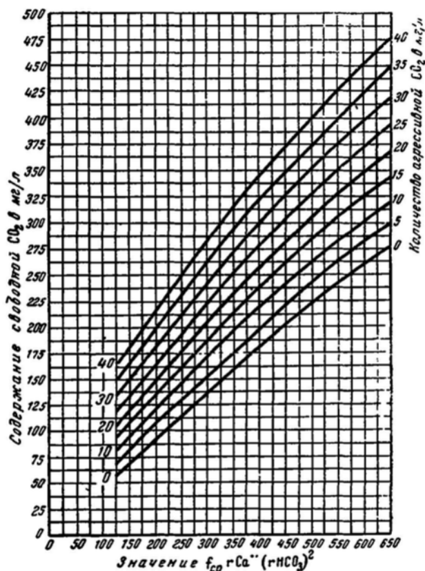
Рис. 3. График для вычисления агрессивной углекислоты при f_{cp} \cdot r\text{Ca}'' \cdot (\text{rHCO}_3)^2 \geq 125
