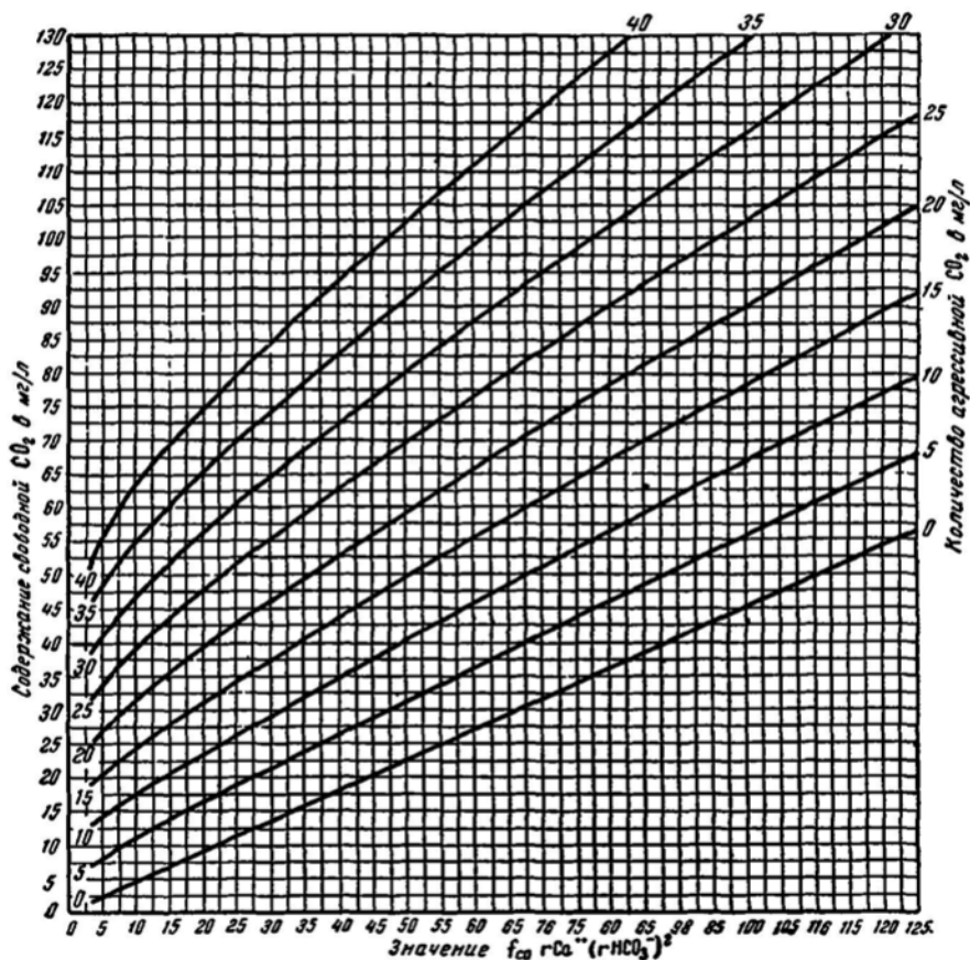
Рис. 2. График для вычисления агрессивной углекислоты при f_{\text{ор}} r\text{Ca}^{++} (r\text{HCO}_3^-)^2 \leq 125
