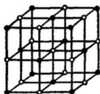
Рис. 1. Строение кристалла NaCl
