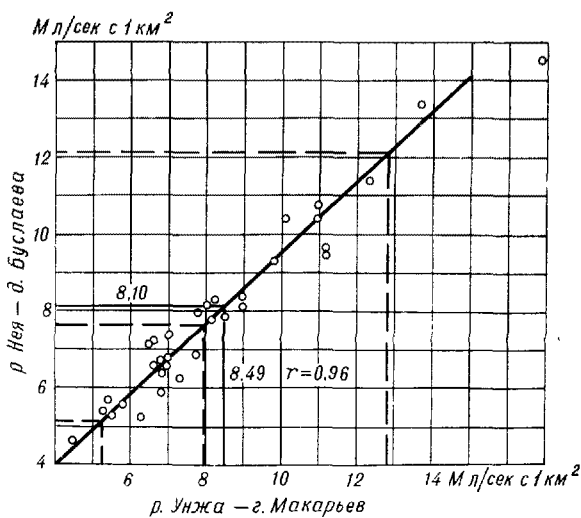
Рис. 3.9. График связи годовых модулей стока р. Унжи у г. Макарьева и р. Нейя у д. Буслаева.
