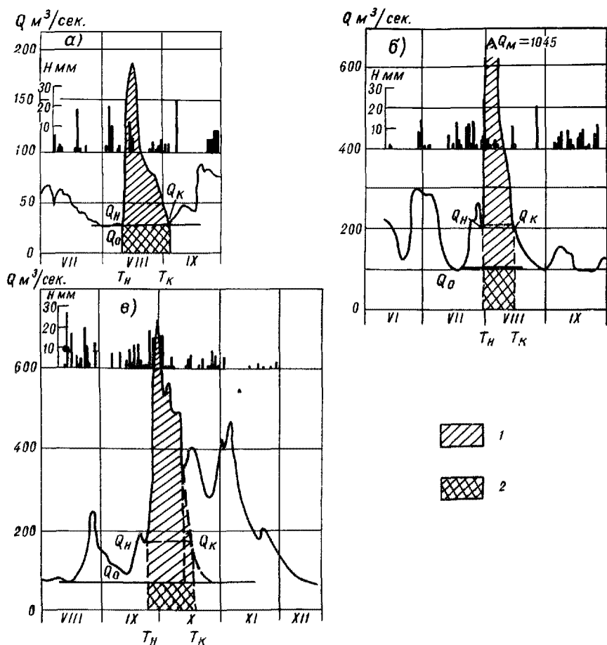
Рис. 2.26. Расчленение стока дождевых паводков на поверхностный и базисный р. Мсты — д. Девкино.
