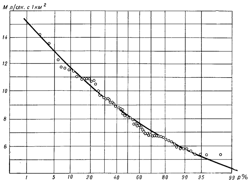
Рис. 3.10. Кривые обеспеченности годовых модулей стока р. Унжи у г. Мантурово.
