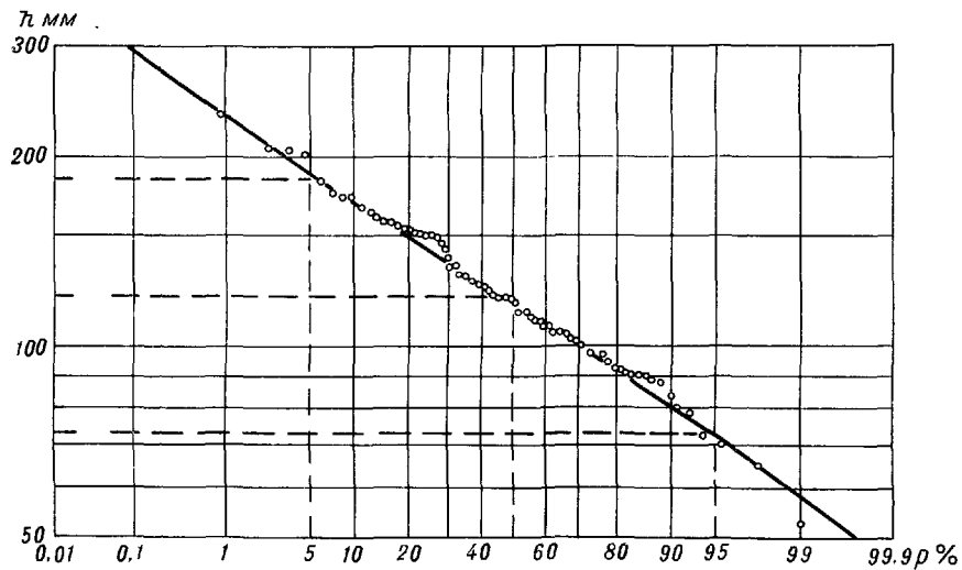
Рис. 7.5. Многолетняя кривая обеспеченности слоя стока весеннего половодья в бассейне р. Тихвинки у с. Горелухи и использование ее для приведения к многолетнему периоду слоя, C_0 и C_s при коротких рядах наблюдений графо-аналитическим методом по трем точкам.
