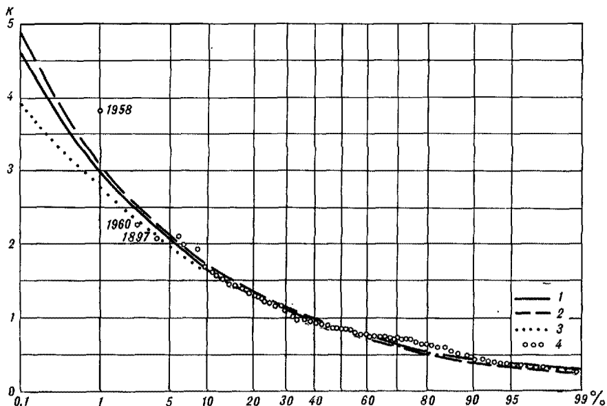
Рис. 7.2. Кривые обеспеченности максимальных расходов воды дождевых паводков р. Амура у с. Покровки за 67 лет наблюдений.
