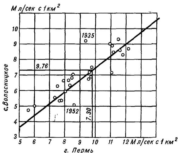
Рис. 3.5. Связь годовых модулей стока р. Камы у г. Перми и р. Камы у с. Волосникового ( r=0,97 ).
