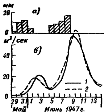
Рис. 8.8. Ход осадков (а) и сток (б) в бассейне р. Кульдур — ст. Известковой.
