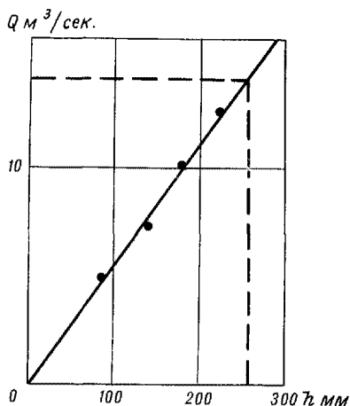
Рис. 7.13. Зависимость максимального среднесуточного расхода от слоя стока р. Люницы у д. Мосолино.
