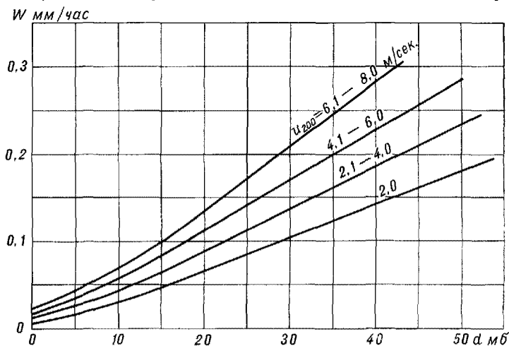
Рис. 2.15. Интенсивность испарения жидких осадков W_{\text{ж}} из осадкомера.
