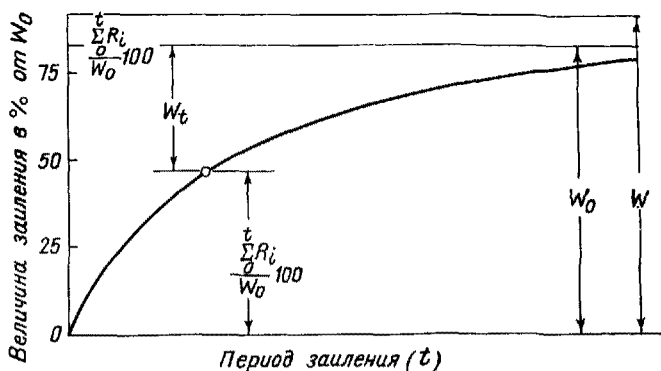
Рис. 9.1. Схема заиления водохранилища с течением времени.
