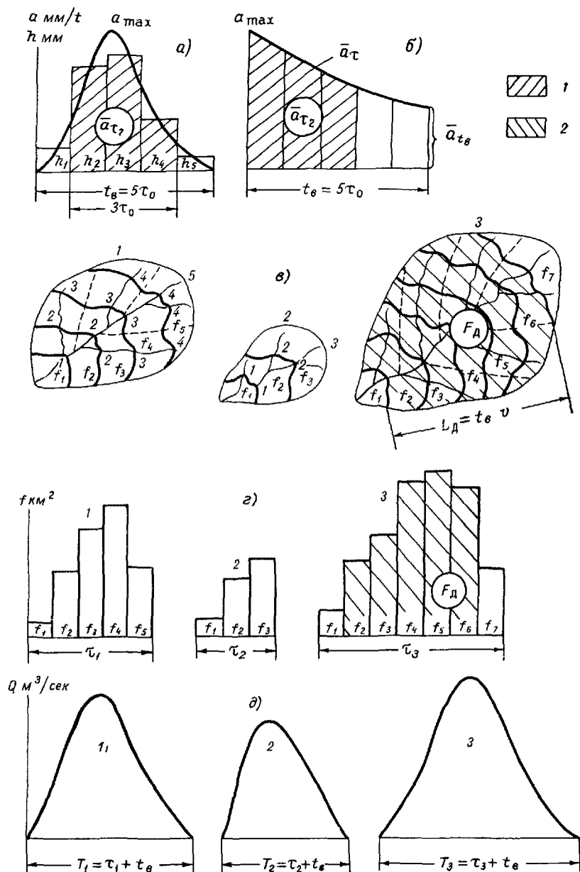
Рис. 7.7. Схема формирования паводков при разных соотношениях \tau и t_\theta
