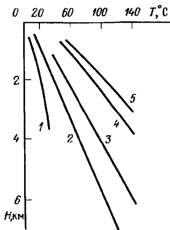
Рис. 9. Графики изменения температуры T на глубине H в артезианских областях (по Г. А. Юдину, 1982 г.).
