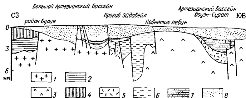
Рис. 46. Схематический геологический профиль через Большой Артезианский бассейн и АБ Боуэн-Сурат.
