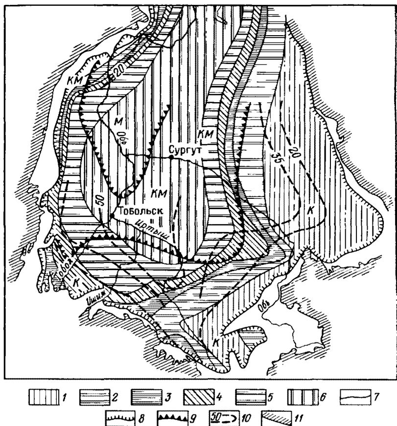
Рис. 26. Гидрохимическая карта альб-ант-сеноманских оглождений Западно-Сибирской АО [39].
