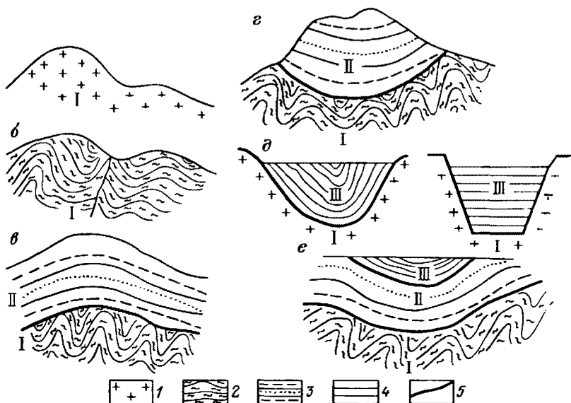
Рис. 3. Структурно-геологическая типизация гидрогеологических массивов: а — \Gamma\text{М}_\text{и} ; б — \Gamma\text{М}_\text{м} ; в — \Gamma\text{АМ} ; г — ГИМ; д, е — ААБ. I — интрузивные породы; 2 — метаморфические породы; 3 — осадочные породы сильнолитифицированные; 4 — то же, среднелитифицированные; 5 — граница между ярусами фундамента. Ярусы фундамента: I — нижний, II — средний, III — верхний
