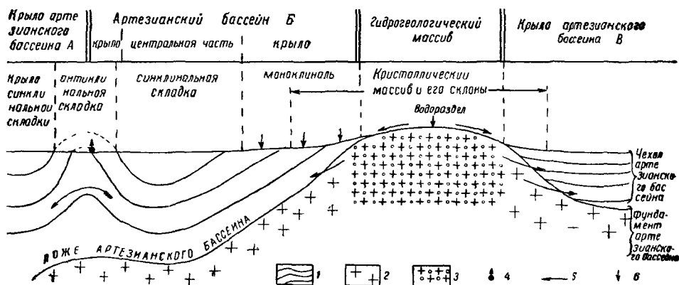
Рис. 1. Характеристика гидрогеологических условий для различных структур 1—слоистые толщи; 2—кристаллические породы фундамента артезианских бассейнов, 3—кристаллические породы, слагающие гидрогеологический массив, 4—восходящий источник, 5—перелив подземных вод из одной структуры в другую; 6—инфильтрация атмосферных осадков
