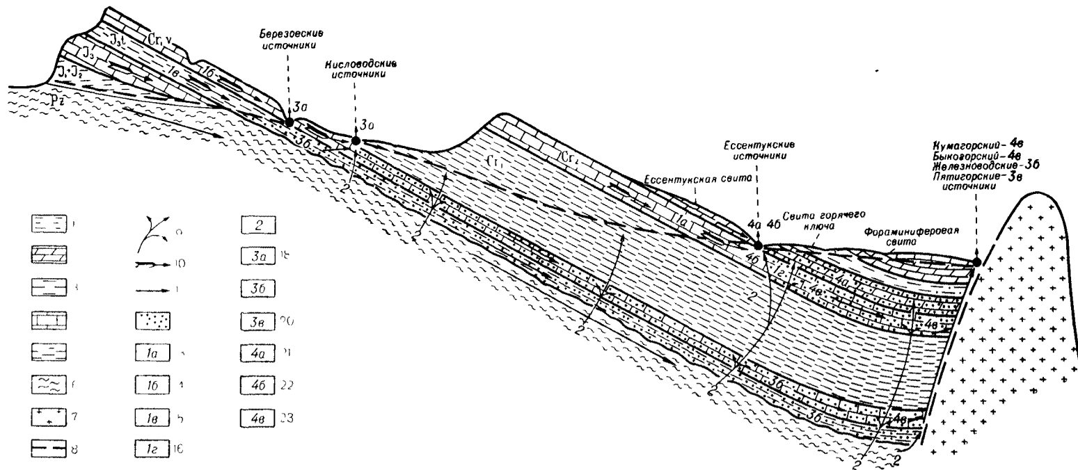
Рис. 10. Схема формирования минеральных вод района КМВ По С. А. Шагоянцу
