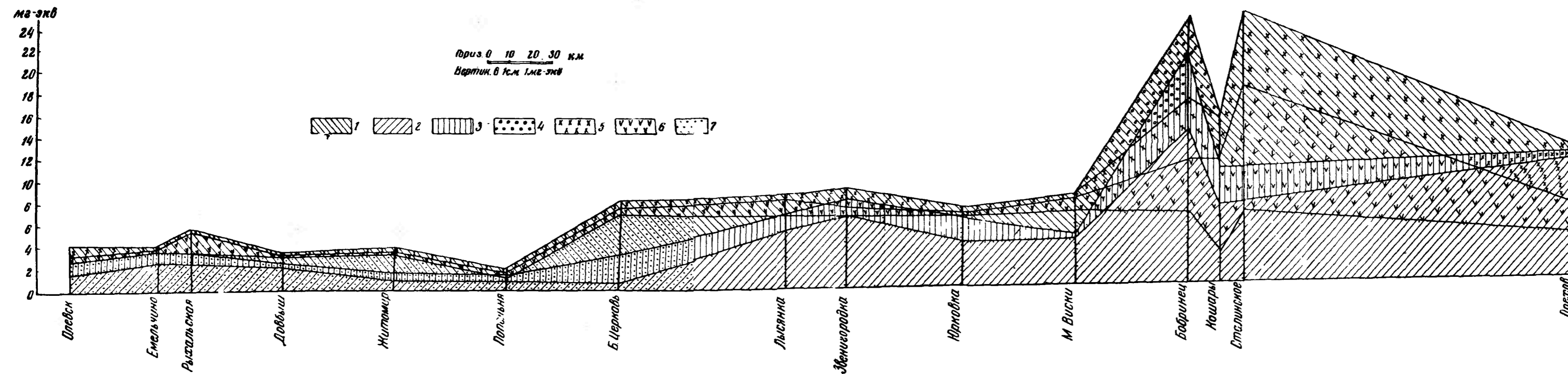
Рис. 9. Гидрохимическая характеристика трещинных вод по профилю Олевск—Орскв Составил Ф. А. Руденко
