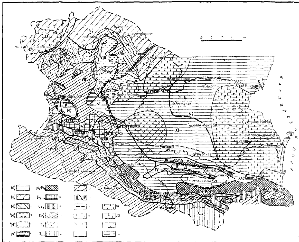
Рис. 6. Карта водоносности дочетвертичных пород Северного Кавказа Составил С. А. Шагоян
