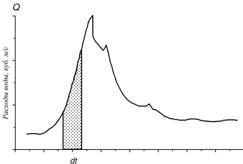
Рис. 11. Гидрограф и элементарный объем стока
