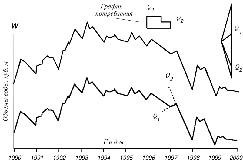
Рис. 19. Расчеты регулирования на двухступенчатый график потребления
