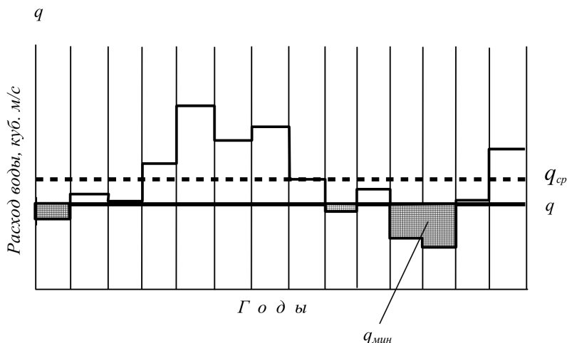
Рис. 8. Схема недельного регулирования стока
