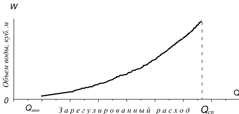
Рис. 16. Зависимость зарегулированного расхода от объема водохранилища
