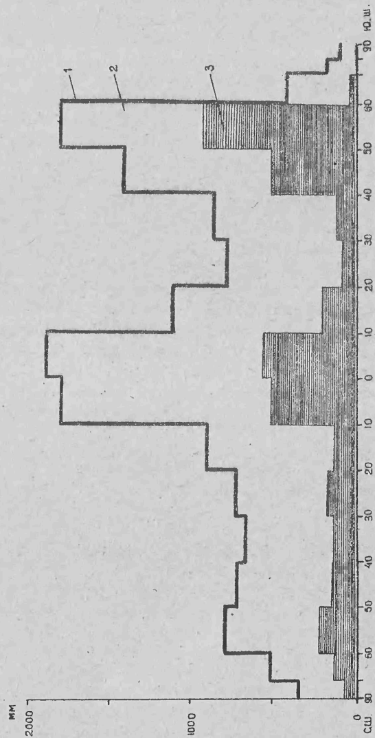
Рис. 1. Широтное распределение осадков (1), испарения (2) и стока (3) на земном шаре
