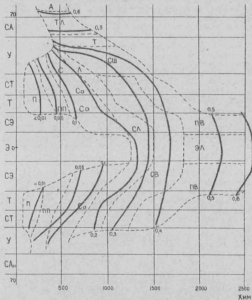
Рис. 4. Коэффициент стока разных природных зон (упрощенно). Географические пояса: Э - экваториальный; СЭ - субэкваториальный; Т - тропический; СТ - субтропический; У - умеренный; СА - субарктический; САН - субантарктический.
