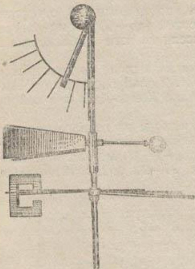
Рис. 68. Флюгер Вильда.
