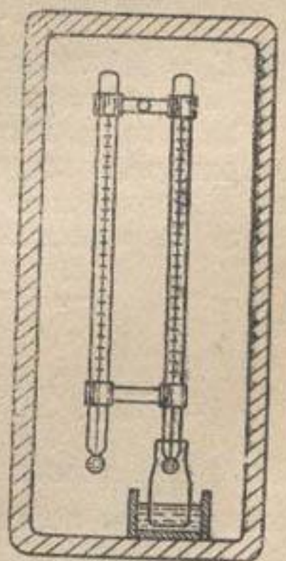
● Рис. 34. Психрометр.
