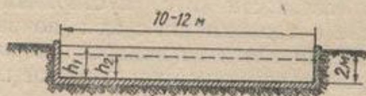
Рис. 37. Береговой испаритель.
