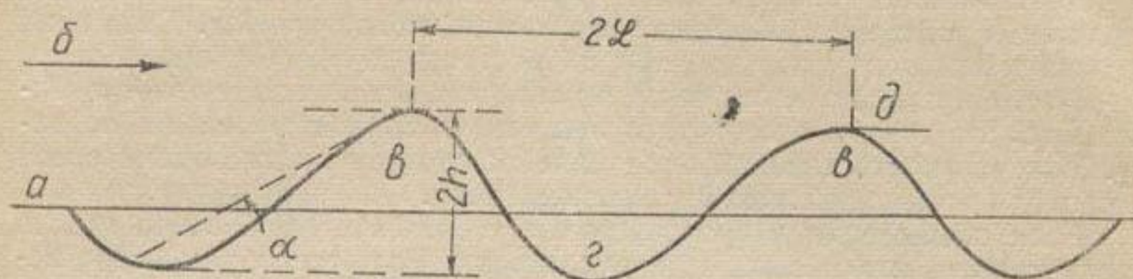
Рис. 125. Элементы ветровой волны: а — статический уровень; б — направление ветра; в — гребень волны; г — впадина; δ — вершина волны; α — крутизна волны.
