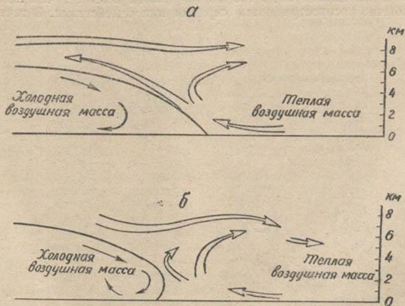
Рис. 27. Схема холодных фронтов первого рода (а) и второго рода (б).
