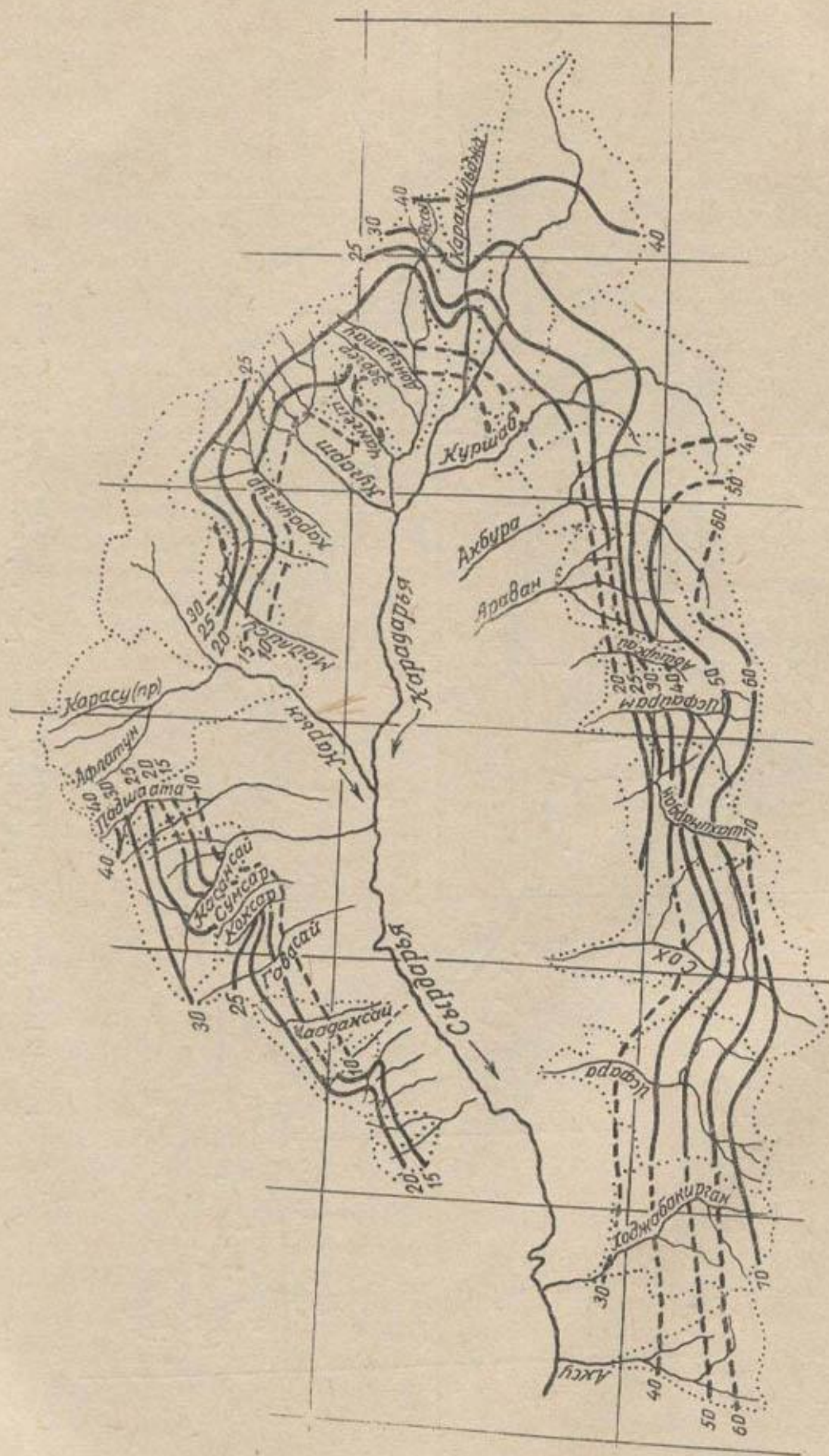
Рис. 123. Схематическая карта стока рек Ферганской котловины за период июль—сентябрь (в процентах от годового).
