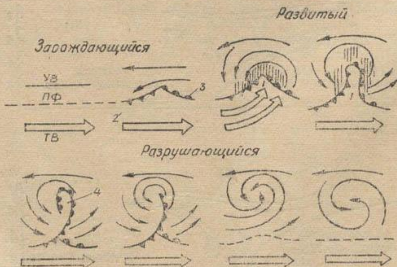
● Рис. 29. Схема развития и разрушения циклона: УВ — умеренный воздух; ПФ — полярный фронт; ТВ — теплый воздух; 1 — теплый сектор; 2 — холодный фронт; 3 — теплый фронт; 4 — окклюзия.
