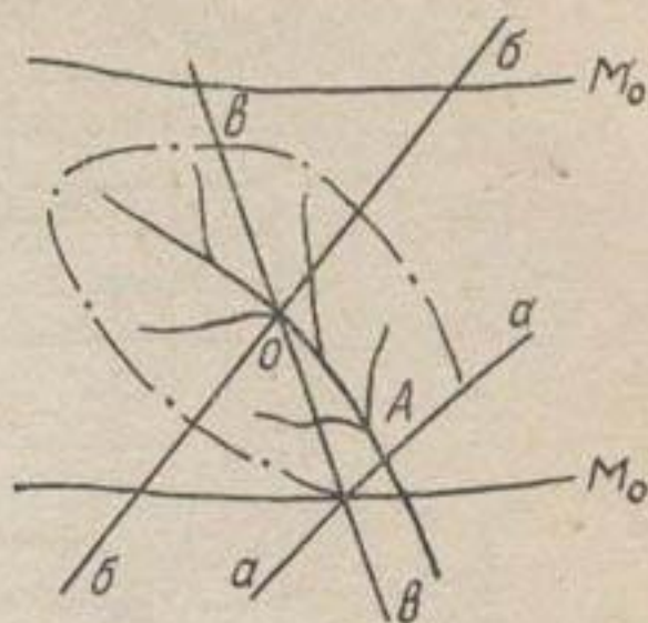
Рис. 100. Определение центра бассейна, распо- ложенного между двумя изолиниями:
