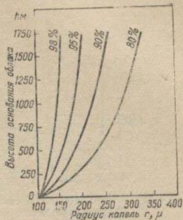
Рис. 49. Испарение капель, выпавших из облака при разных значениях относительной влажности (по Мейсону).
