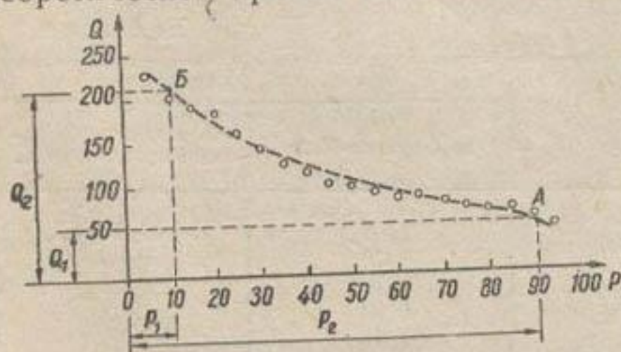
● Рис. 97. Выбор исходных точек A и B для определения параметров теоретической кривой обеспеченности по расположению натурных точек.
