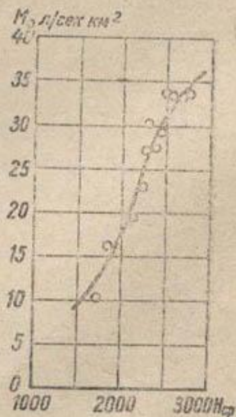
Рис. 87. Зависимость среднего многолетнего модуля стока ( M_0 ) от средней взвешенной высоты водосбора ( H_{ср} ) для рек южного склона Гиссарского хребта.
