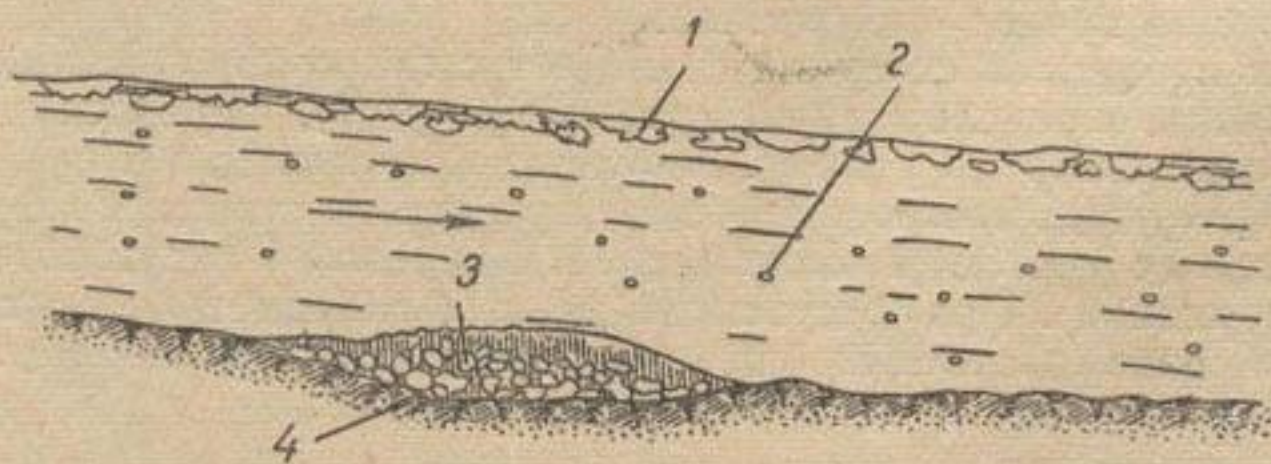
Рис. 159. Схема образования шуги (температура воды меньше нуля):
