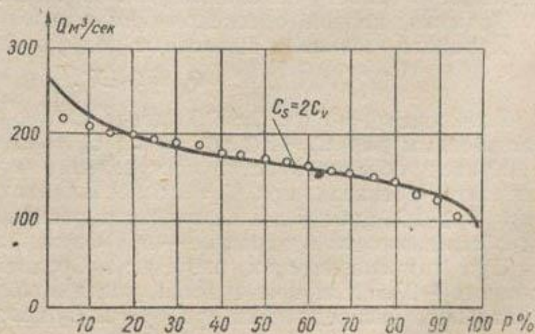
Рис. 95. Расхождение теоретической кривой с натурными точками при завышенном значении C_v .
