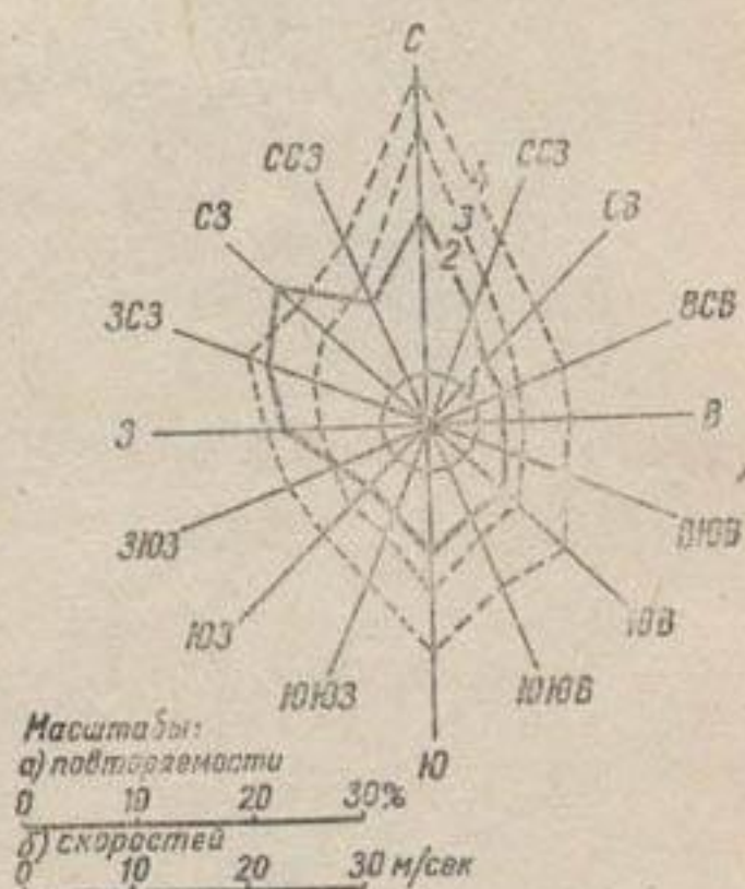
Рис. 70. Роза ветров:
