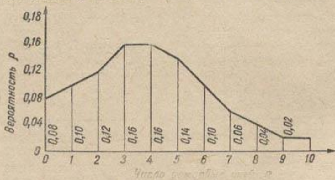
Рис. 3. Многоугольник распределения.
