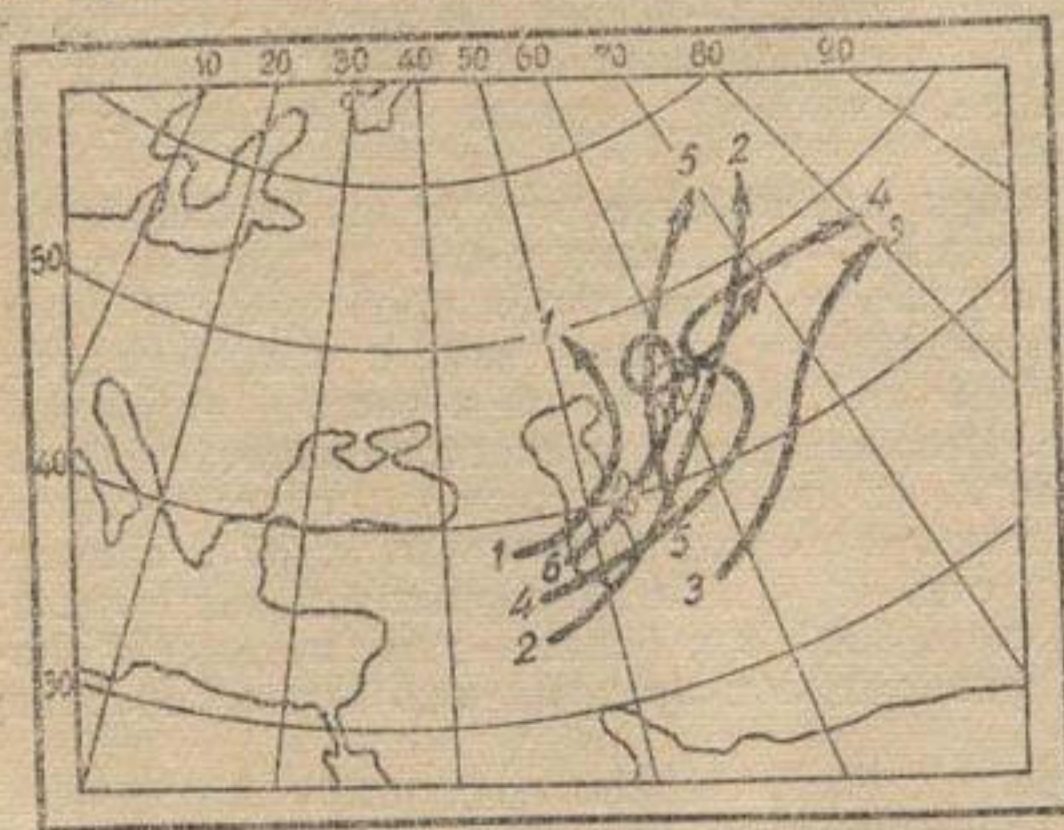
Рис. 31. Типовые траектории антициклонов.
