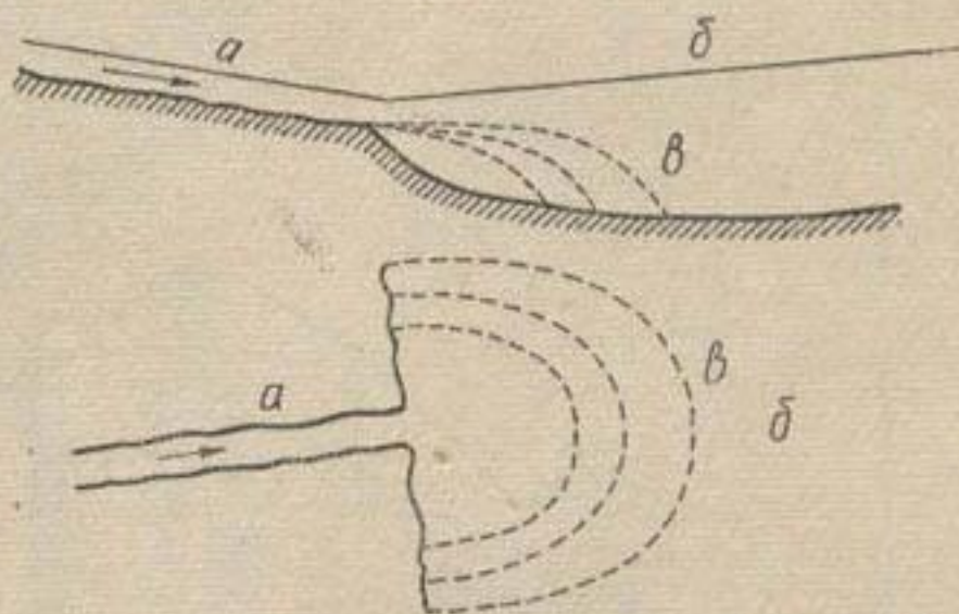
Рис. 135. Схема образования бара: а — река; б — море; в — отложение речных наносов (бар).
