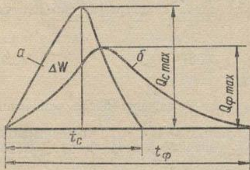
Рис. 77. Трансформация гидрографа стекания a в фактический гидрограф б ; \Delta W — объем воды, временно задерживающийся на склонах и в гидрографической сети.
