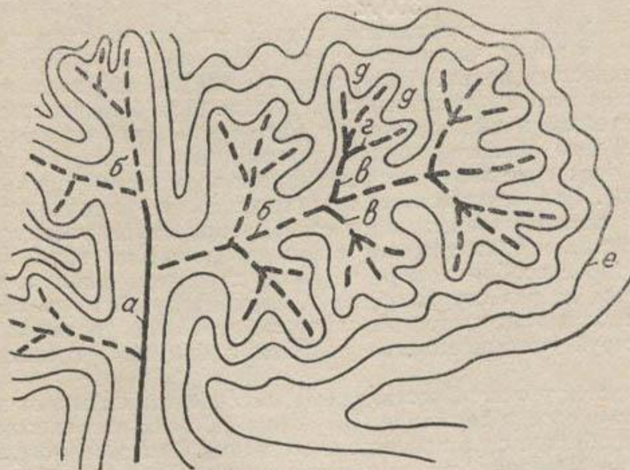
Рис. 73. Гидрографическая сеть:
