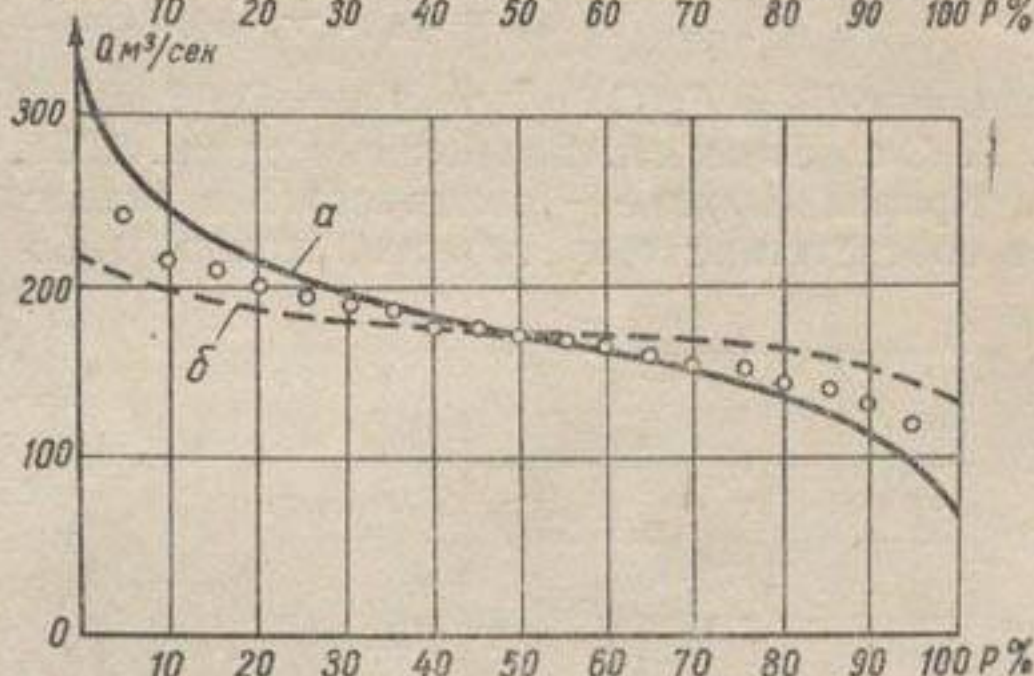
Рис. 93. Расхождение теоретической кривой обеспеченности с натурными точками из-за ошибки в величине C_v .
