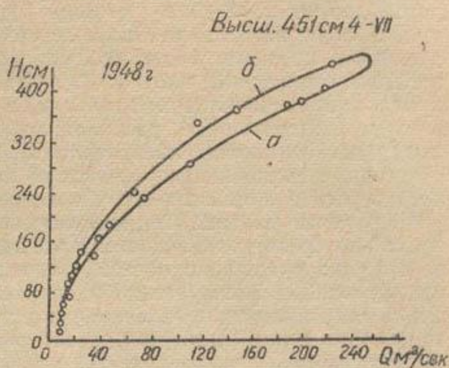
Рис. 158. Кривая Q = f(H) ; р. Фандарья, устье за 1948 г. а — на подъеме; б — на спаде паводка.
