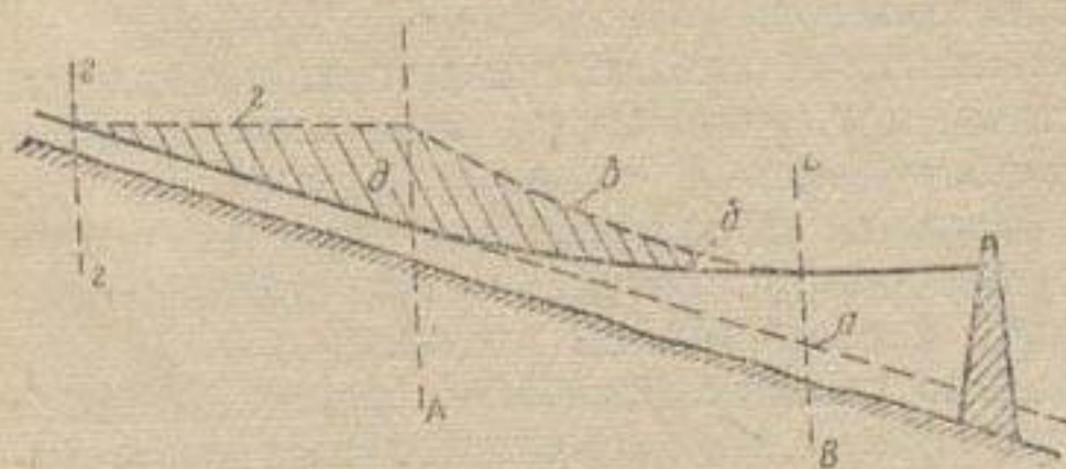
● Рис. 163. Схема образования зазора в верхнем бьефе плотинных гидроузлов:
