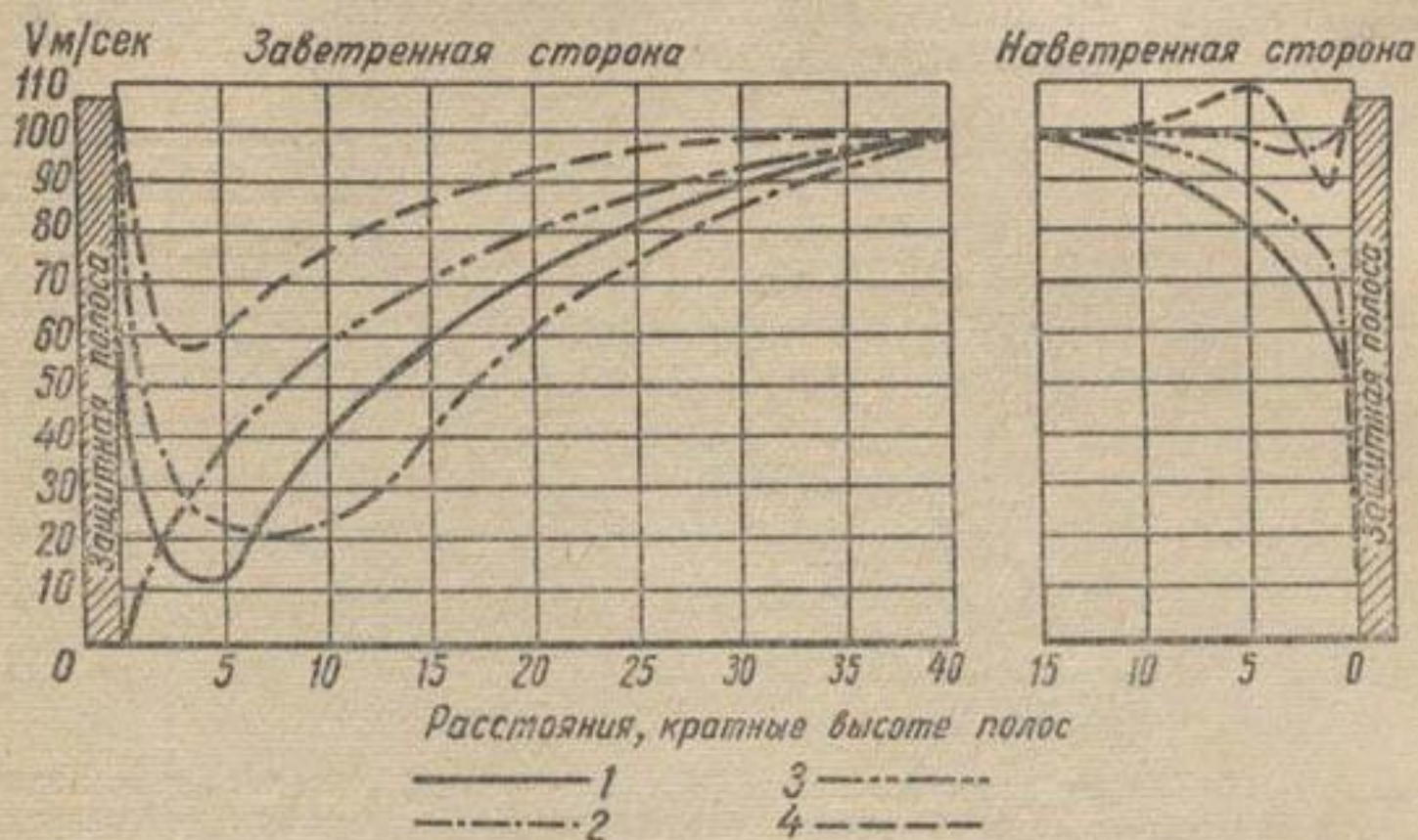
Рис. 40. Изменение скорости ветра на высоте 100 см, под влиянием полевых защитных лесных полос (в % от скорости ветра на открытом месте):
