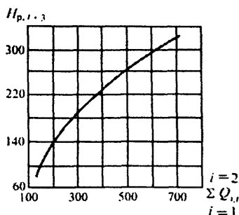
Рис. 3.6. Связь уровней р. Днестра у с. Речица ( H_{p, (n+3)} ) с суммой соответственных расходов воды р. Днестра у г. Жлобина и р. Березины у г. Светлогорска \left( \sum_{i=1}^{i=2} Q_{i, t} \right) при заблаговременности 3 сут.
