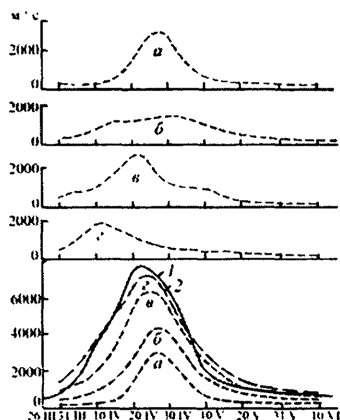
Рис. 7.35. Фактический (1) и предсказанный (2) по стоку с четырех частей бассейна гидрограф р. Оки у г. Горбатова за половодье 1968 г.: а - Ока до Каширы; б - Кашира-Касимов; в - Касимов Муром; г - Муром-Горбатов.
