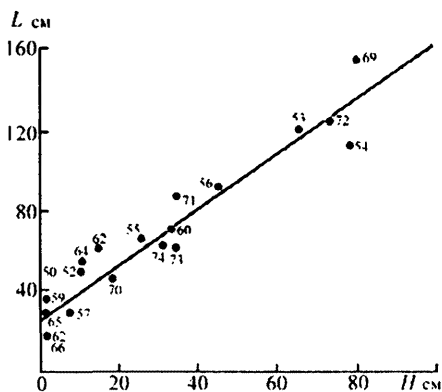
Рис. 7.6. Связь глубины промерзания почвы с мощностью расчетного водонепроницаемого слоя. Цифры у точек - годы.
