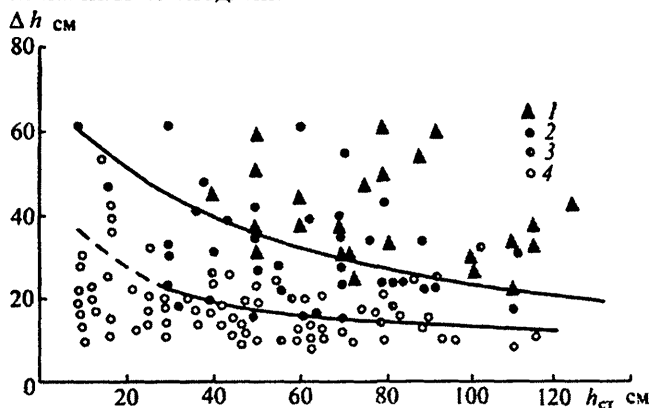
Рис. 12.7. Связь лавинообразования с приростом высоты слоя свежеснеговывпавшего снега ( \Delta h ) и высотой слоя старого снега в лавиносборах ( h_{ст} ).
