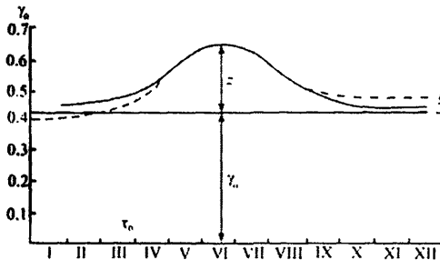
Рис. 8.4. Аппроксимация внутригодового хода вертикального градиента температуры воздуха: 1 фактический ход на склоне Ферганского хребта, 2 его аппроксимация.
