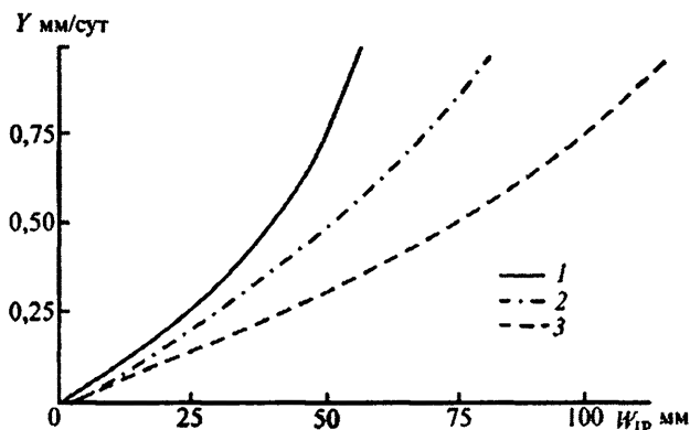
Рис. 7.9. Зависимость запасов грунтовых вод W_{\text{гр}} от суточного слоя стока рек Y на спаде паводков и в межень для водосборов лесной зоны ЕТР: 1 – водосборы с суглинистыми грунтами на 90 % площади; 2 – водосборы с суглинисто-супесчаными грунтами (пески занимают 35 % площади); 3 – водосборы с песчаными грунтами на 60 % площади.
