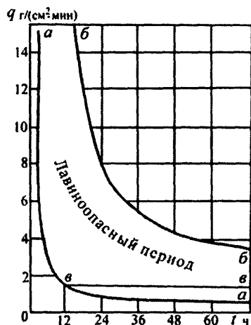
Рис. 12.8. Продолжительность периода лавинной опасности при метелях.
