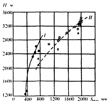
Рис. 8.1. Соотношение между максимальными снегозапасами и высотой места на склонах южной (I) и северной (II) экспозиции.
