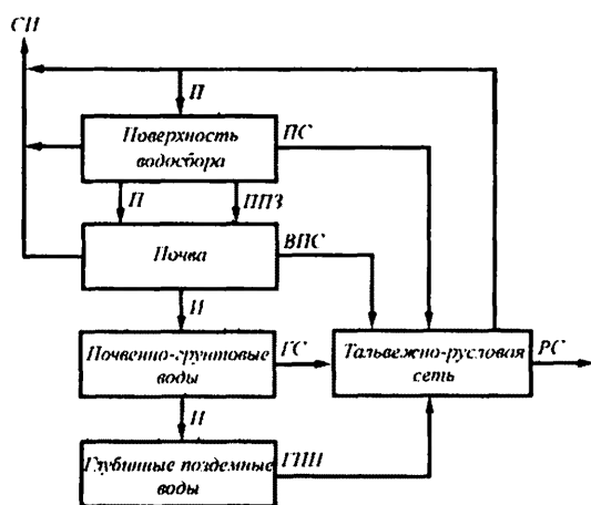
Рис. 7.1. Речной бассейн как динамическая система.
