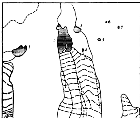
Рис. 12.1. Ледник Туюксу и моренные озера в бассейне р. Малой Алматинки.
