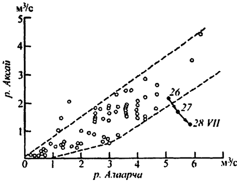
Рис. 12.4. Корреляционный график расхода воды р. Аксай (устье) и Алаарча (выше устья р. Джендысу) за 1961 г. (северный склон Киргизского хребта). Селевой поток прошел 29 июля.
