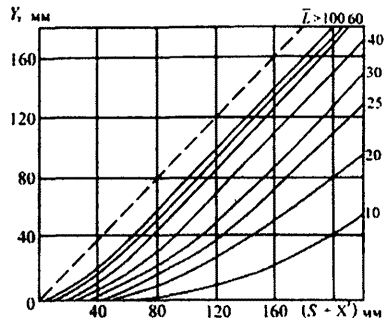
Рис. 7.17. Территориально общая зависимость слоя стока талых вод от снегозапасов и осадков (S + X') и средней глубины промерзания \bar{L} для водосборов IV района в годы, когда запасы влаги в метровом слое почвы W_{0,100} \geq 300 мм.
