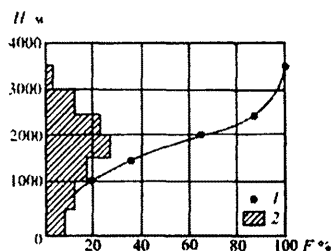
Рис. 8.2. Гипсографическая кривая бассейна реки: 1 — суммарная кривая; 2 — распределение площадей по высотным зонам.
