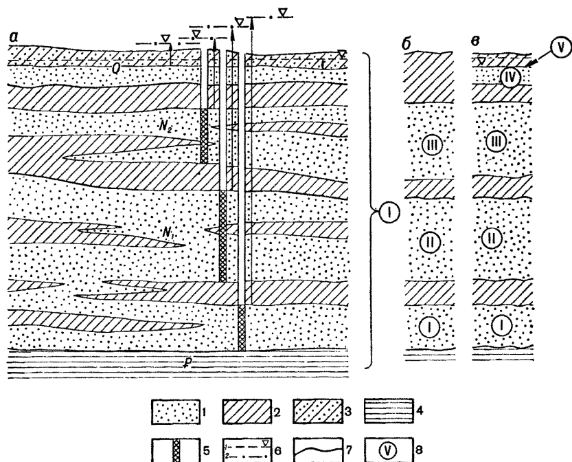
Рис. 21. Схематизация геолого-гидрогеологического разреза сложно-слоистой водоносной толщи для оценки ЭЗПВ:
