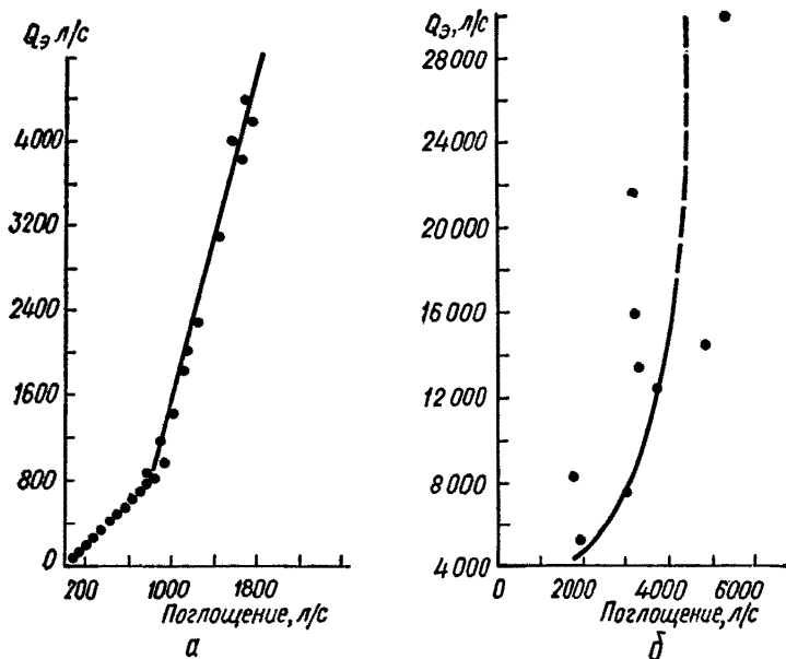
Рис. 36. Графики зависимостей величины поглощения поверхностного стока от суммарного расхода на входных створах 1 и 2:
