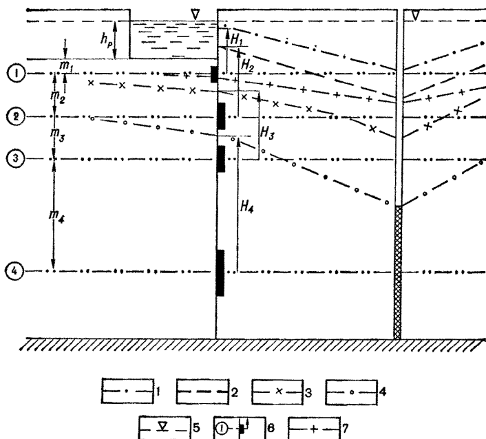
Рис. 65. Схема распределения напоров вблизи реки по глубине водозаборного сооружения:
