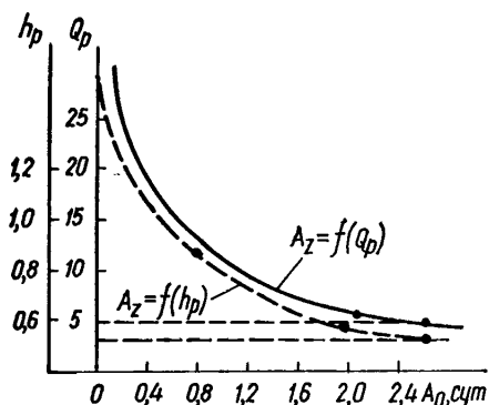
Рис. 66. Графики зависимости A_z = f(Q_p) , A_z = f(h_p) в долинах горных рек
