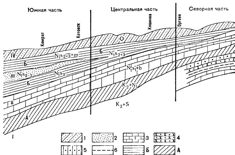
Рис. 68. Схематизация разреза Днестровско-Прутского междуречья для районирования территории при региональной оценке прогнозных эксплуатационных ресурсов подземных вод:
