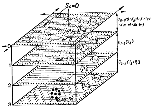
Рис. 27. Геофильтрационная модель Кольчугинского месторождения подземных вод для прогнозирования снижения уровня грунтовых вод (по Г. Е. Ершову, 1986). Условные обозначения см. рис. 26.
