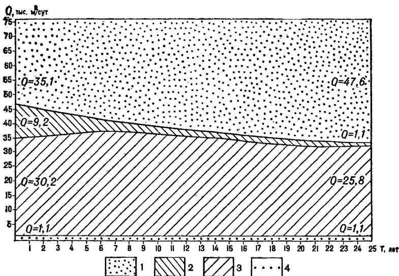
Рис. 52. График баланса прогнозного водоотбора (по фрагменту модели Кольчугинского месторождения) по результатам моделирования на ЦВМ (по данным Г. Е. Ершова, 1986):
