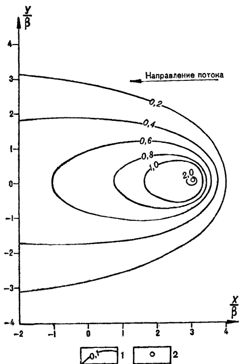
Рис. 48. Схема воронки депрессии в безнапорном потоке на наклонном водоупоре в изолиниях безразмерного понижения уровня \frac{S}{4\pi k h_e} = \exp\left(-\frac{r}{\beta} \cos \theta\right) K_0\left(\frac{r}{\beta}\right) : 1 — изолинии безразмерных понижений; 2 — водозаборная скважина
