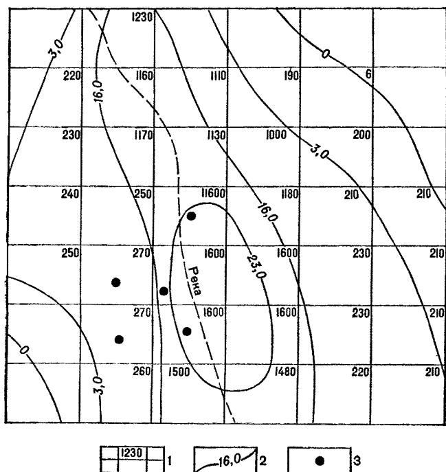
Рис. 51. Схематическая карта величин перетока через юрско-пермскую глинистую толщу в клязьминско-ассельский водоносный горизонт на фрагменте модели Кольчугинского месторождения (рис. 19) по данным моделирования на ЦВМ, водоотбор 51,8 тыс. м 3 /сут (по данным Г. Е. Ершова, 1986):
