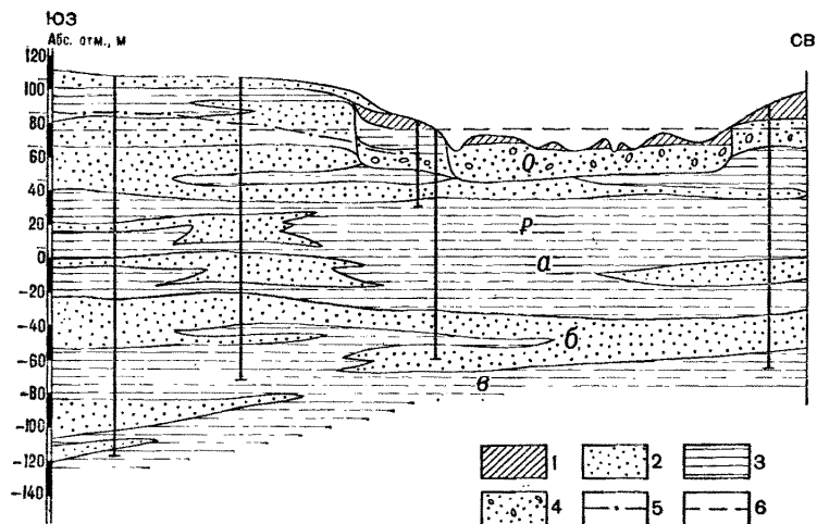
Рис. 32. Схематический гидрогеологический разрез водозаборного участка в районе г. Томска:
