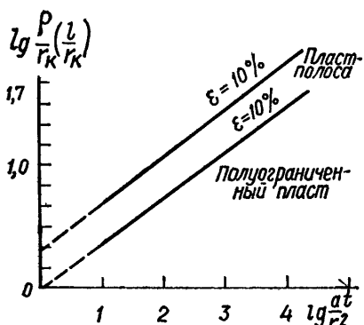
Рис. 28. График для определения условий, в которых расчеты в пласте-полосе и полуограниченном пласте можно вести с ошибкой 10 % по формулам для неограниченного пласта
