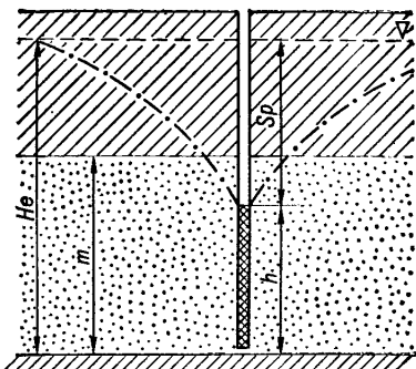
Рис. 38. Схема к расчету понижения уровня в одиночной скважине в условиях напорно-безнапорной фильтрации
