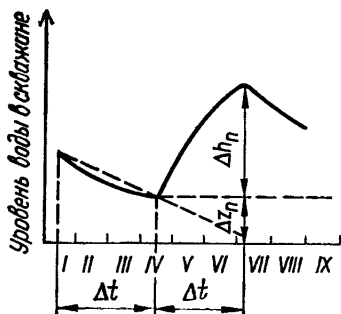
Рис. 10. Схема к расчету питания грунтовых вод путем анализа режима их уровня в одиночной скважине (по Н. Н. Биндеману, 1963)
