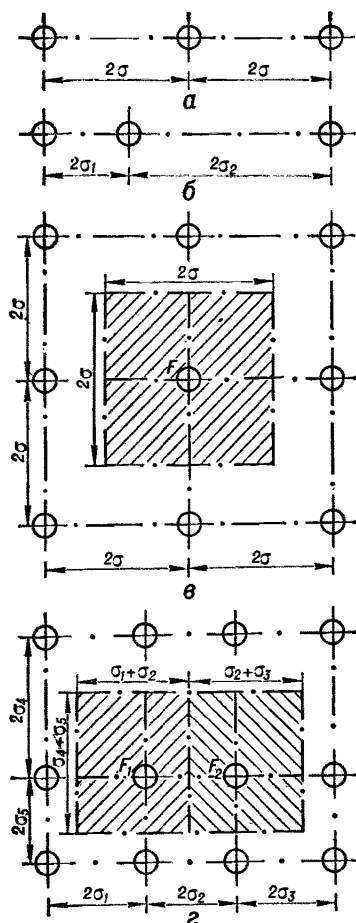
Рис. 40. Схема расположения скважин в обобщенных системах: линейной при равных расстояниях между скважинами (а) и разных (б); площадной (в и г)
