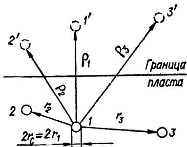
Рис. 44. Схема к расчету скважин в полуограниченном пласте
