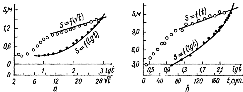
Рис. 53. Графики экспериментальных зависимостей для прогноза снижения уровня во времени гидравлическим методом:
