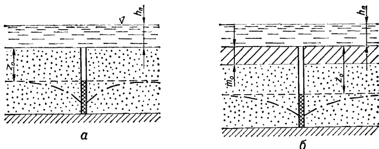
Рис. 67. Схемы к расчету восполнения сработанных запасов подземных вод при затоплении поймы:
