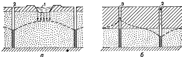
Рис. 61. Схемы сооружений искусственного пополнения подземных вод открытого (а) и закрытого (б) типов:
