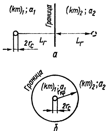
Рис. 45. Схема к расчету скважины в неоднородных пластах с прямолинейной (а) и круговой (б) границей раздела
