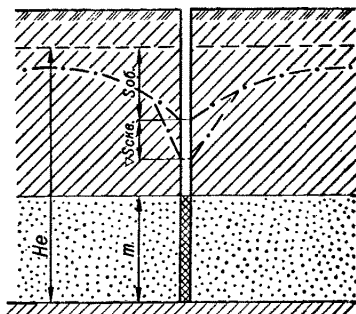
Рис. 39. Схема к расчету понижения в водозаборной скважине методом обобщенных систем
