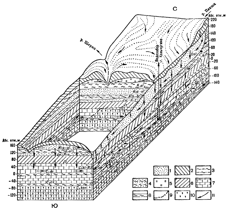
Рис. 19. Схема природной гидрогеологической модели Кольчугинского месторождения подземных вод (по В. С. Беляеву, Б. В. Боровскому, Г. Е. Ершову, 1986):
