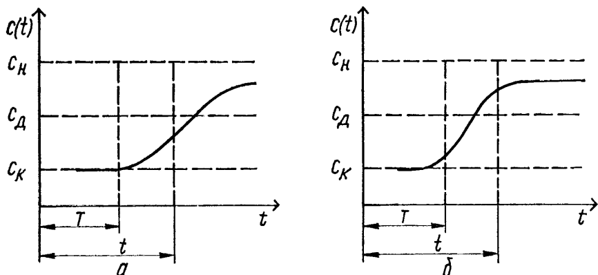
Рис. 57. Графики изменения качества воды во времени без превышения концентрации загрязняющих веществ (а) допустимой нормы и при формировании в течение расчетного периода эксплуатации некондиционных вод (б)
