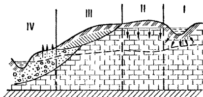
Рис. 30. Схема возможных условий на верхней границе безнапорного водоносного горизонта:
