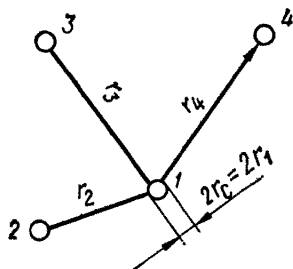
Рис. 37. Схема к расчету взаимодействующих скважин в неограниченном пласте
