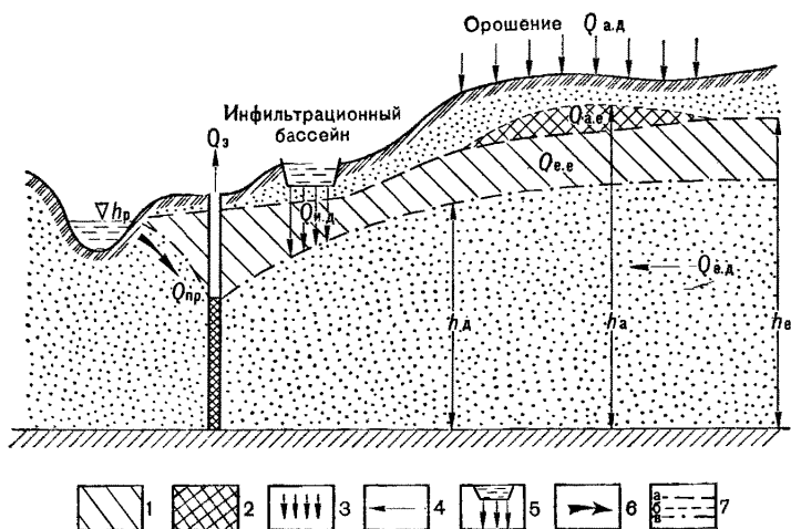
Рис. 4. Схема формирования ЭЗПВ ( Q_э ) за счет различных источников:
