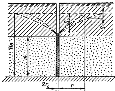
Рис. 42. Схема к расчету скважины при откачке с постоянным понижением уровня
