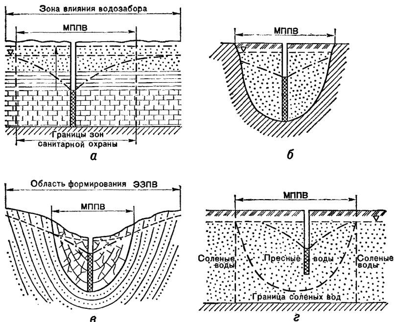
Рис. 6. Основные схемы выделения границ месторождений подземных вод:
