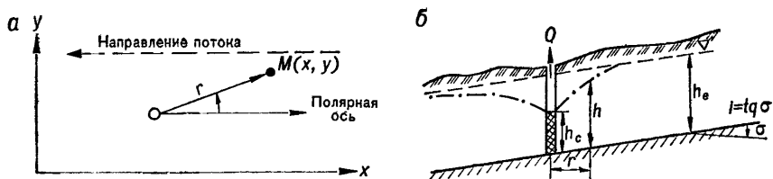
Рис. 47. Схема к расчету скважины в безнапорном пласте на наклонном водоупоре (по М. Хантушу, 1962):
