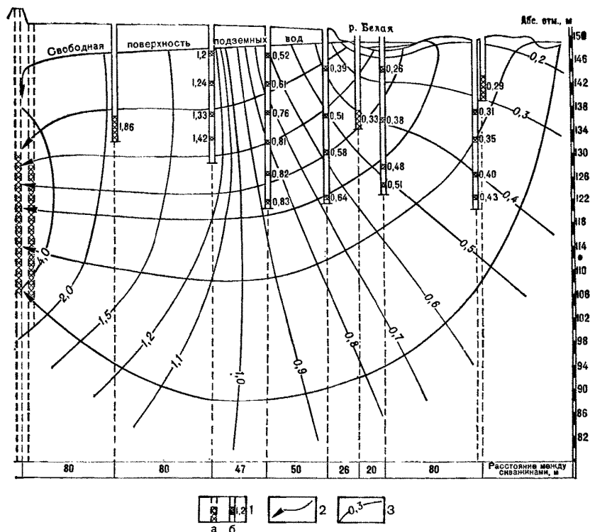
Рис. 25. Схематическая гидродинамическая сетка при работе водозаборного сооружения в долине р. Белой (по П. И. Аверкову и М. С. Верзакову, 1976):
