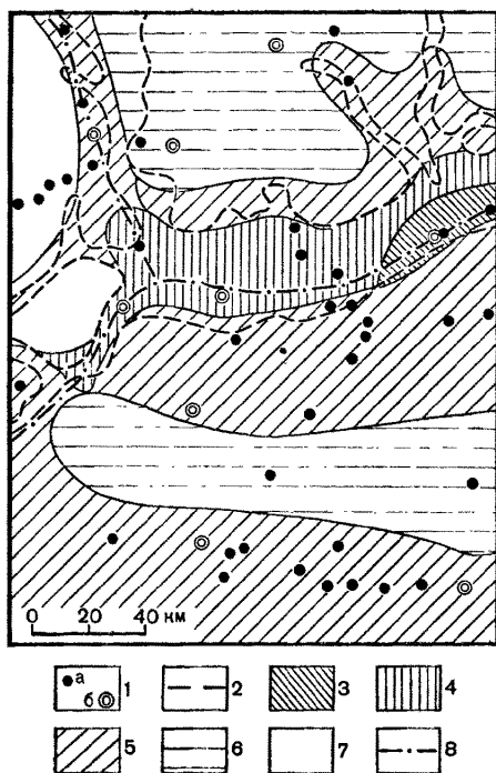
Рис. 24. Фрагмент карты вертикального коэффициента фильтрации верхнеюрских глин Средне-Клязьминского месторождения подземных вод (по Б. В. Боревскому, М. В. Кочеткову, Т. А. Плугиной, Н. Н. Шарапанову, 1981):
