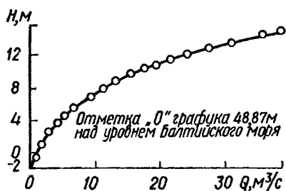
Рис. 12. Кривая расходов реки
