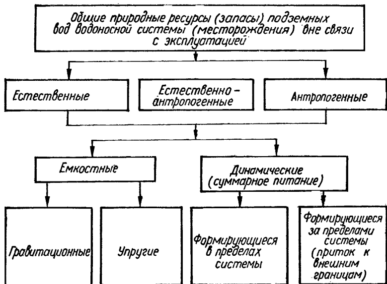
Рис. 2. Классификация ресурсов (запасов) подземных вод
