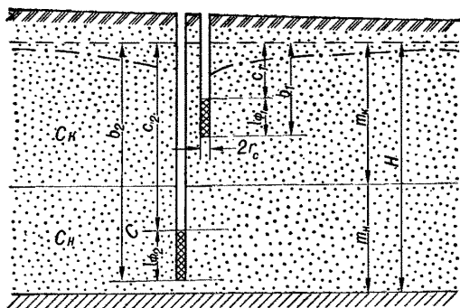
Рис. 58. Схема к расчету спаренных скважин для защиты водозаборного сооружения от подтягивания некондиционных вод снизу
