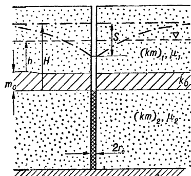
Рис. 46. Схема к расчету скважины в трехслойном пласте
