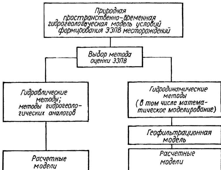
Рис. 18. Общая структура схематизации условий формирования ЭЗПВ оцениваемого месторождения
