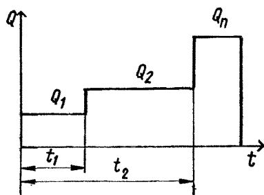
Рис. 41. График скачкообразного изменения дебита скважины
