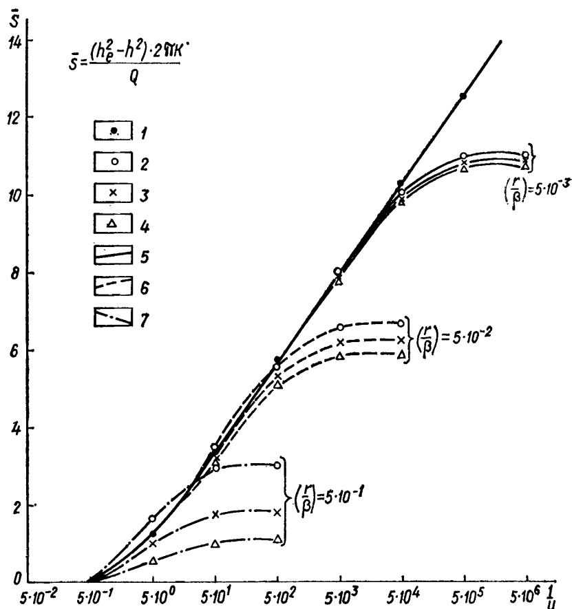
Рис. 49. Графики безразмерного понижения уровня в безнапорном потоке на наклонном водоупоре \bar{S} = f\left(\lg \frac{1}{u}\right) при u = \frac{r^2}{4at} :
