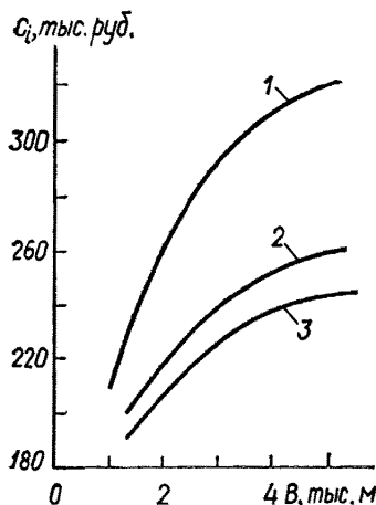
Рис. 69. График зависимости приведенных затрат от фактора перетекания B при различных значениях водопроводимости продуктивного горизонта, \text{м}^2/\text{сут} : 1 — 200; 2 — 250; 3 — 300
