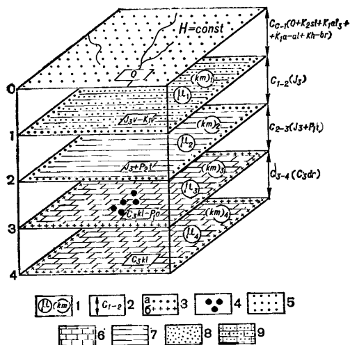
Рис. 26. Геофильтрационная модель Кольчугинского месторождения подземных вод для воспроизведения опыта эксплуатации:
