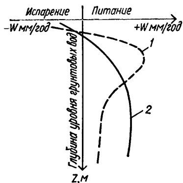
Рис. 11. График зависимости величины питания грунтовых вод от глубины залегания их уровня:
