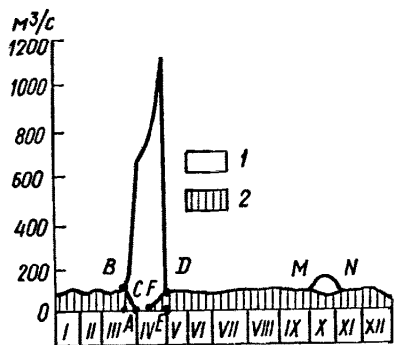
Рис. 15. Выделение подземного стока на гидрографе реки:
