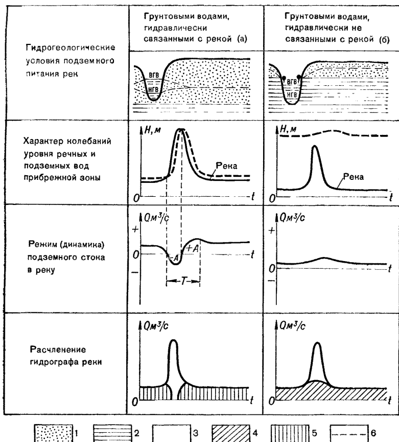
Рис. 14. Типовые схемы расчленения гидрографа реки (по Б. И. Куделину, 1960): 1 — водоносные породы; 2 — водоупорные породы; 3 — поверхностный сток; 4 — подземный сток из водоносных горизонтов, гидравлически не связанных с рекой; 5 — то же для гидравлически связанных с рекой; 6 — уровень подземных вод
