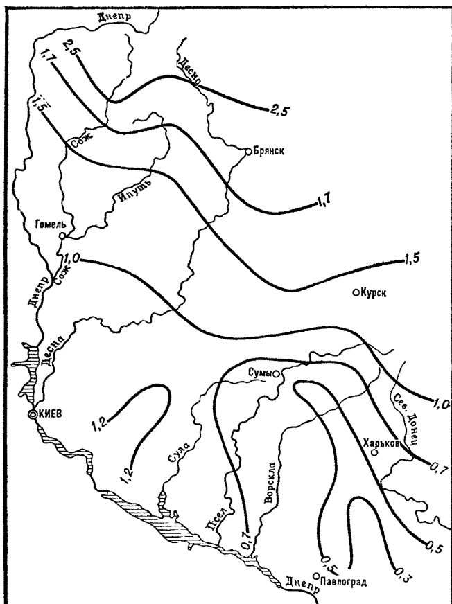
Рис. 16. Схематическая карта среднегодовых модулей подземного стока в реки, в л/с·км 2 (по Б. И. Куделину, 1960)
