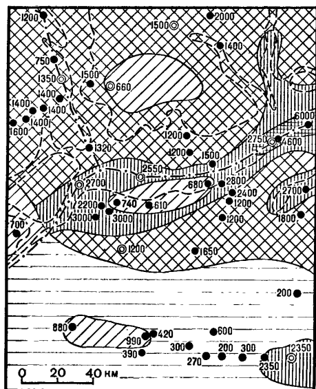
Рис. 23. Фрагмент карты водопроницаемости клязьминско-ассельского водоносного горизонта Средне-Клязьминского МПВ в Московском артезианском бассейне (по Б. В. Боровскому, М. В. Кочеткову, Т. А. Плугиной, Н. Н. Шапранову, 1981):
