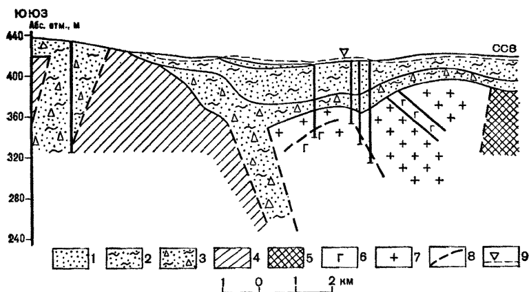
Рис. 31. Гидрогеологический разрез (район г. Щучинска, Казахстан):
