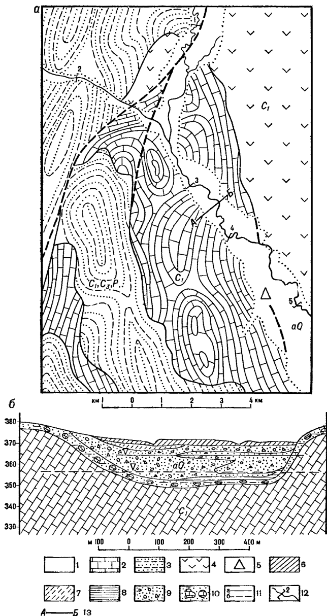
Рис. 34. Гидрогеологическая карта (а) и разрез (б) Мало-Кизильского месторождения подземных вод (по Г. А. Никитиной, 1976):
