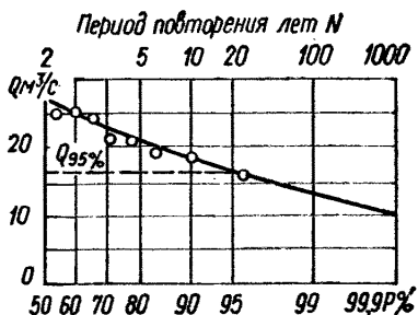
Рис. 13. Кривая обеспеченности расхода реки
