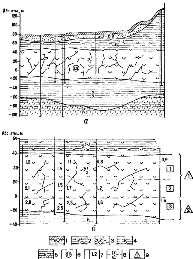
Рис. 20. Геолого-гидрогеологический разрез Шадринского месторождения подземных вод (а) и его схематизация для прогноза изменения качества на природной гидрогеологической модели (б):
