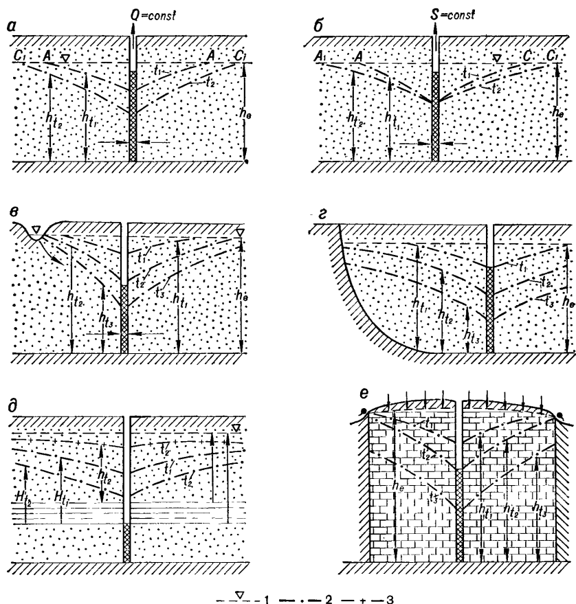
Рис. 5. Схема формирования воронки депрессии при работе водозаборных сооружений при типовых граничных условиях:
