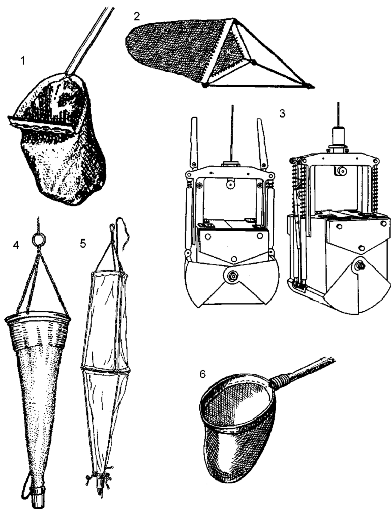
Рис. 4. Орудия сбора бентоса и планктона (по: Чертопруд, Чертопруд, 2003): 1 – скребок; 2 – закидная треугольная дрга; 3 – дночерпатель Экмана-Берджа в раскрытом и закрытом виде; 4 – качественная планктонная сеть Апштейна; 5 – количественная планктонная сеть Джеди; 6 – планктонный сачок
