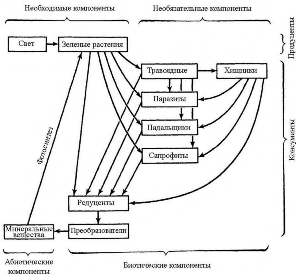
Рис. 8. Принципиальные уровни и компоненты самодостаточной экосистемы (по: Clarke, 1954)
