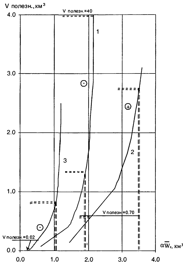
Рис.3.4. Кривые зависимости гарантированной водоотдачи ( a\bar{W}_r ) от полезного объема водохранилища ( V )
